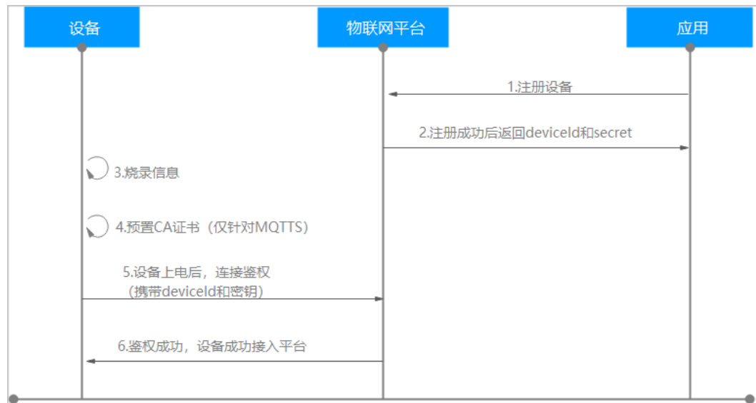
图 2-2 使用原生 MQTT/MQTTs 协议接入的鉴权流程
