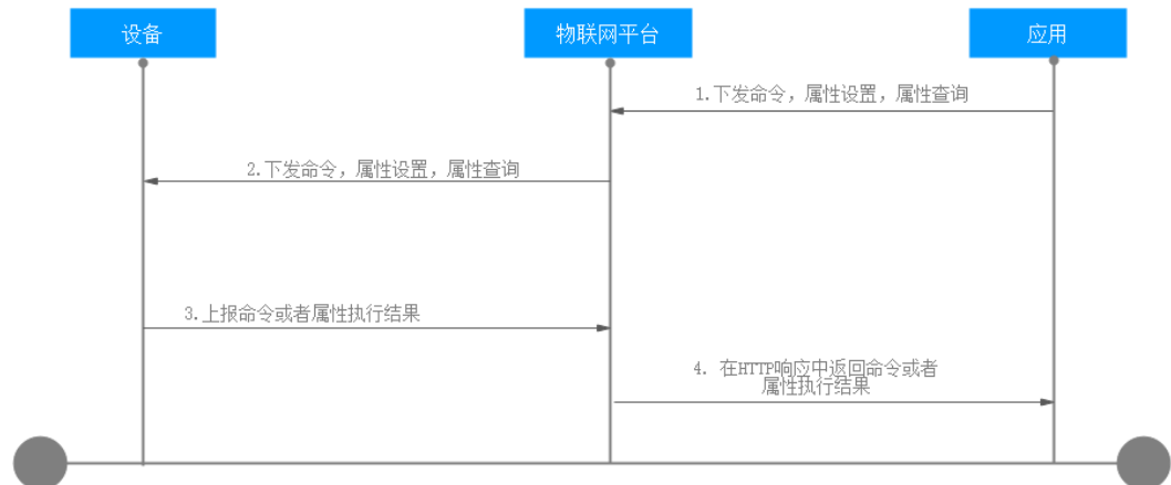
图 3-27 命令下发流程图
