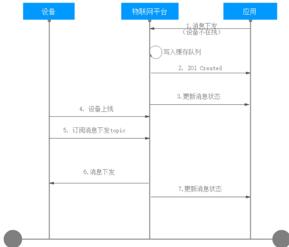
图 3-14 消息缓存下发流程
