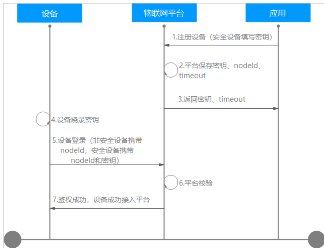
图 2-1 使用 LwM2M/CoAP 协议接入的鉴权流程
