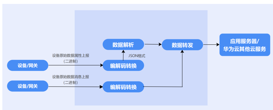
图 3-3 原始二进制数据上报概念图
