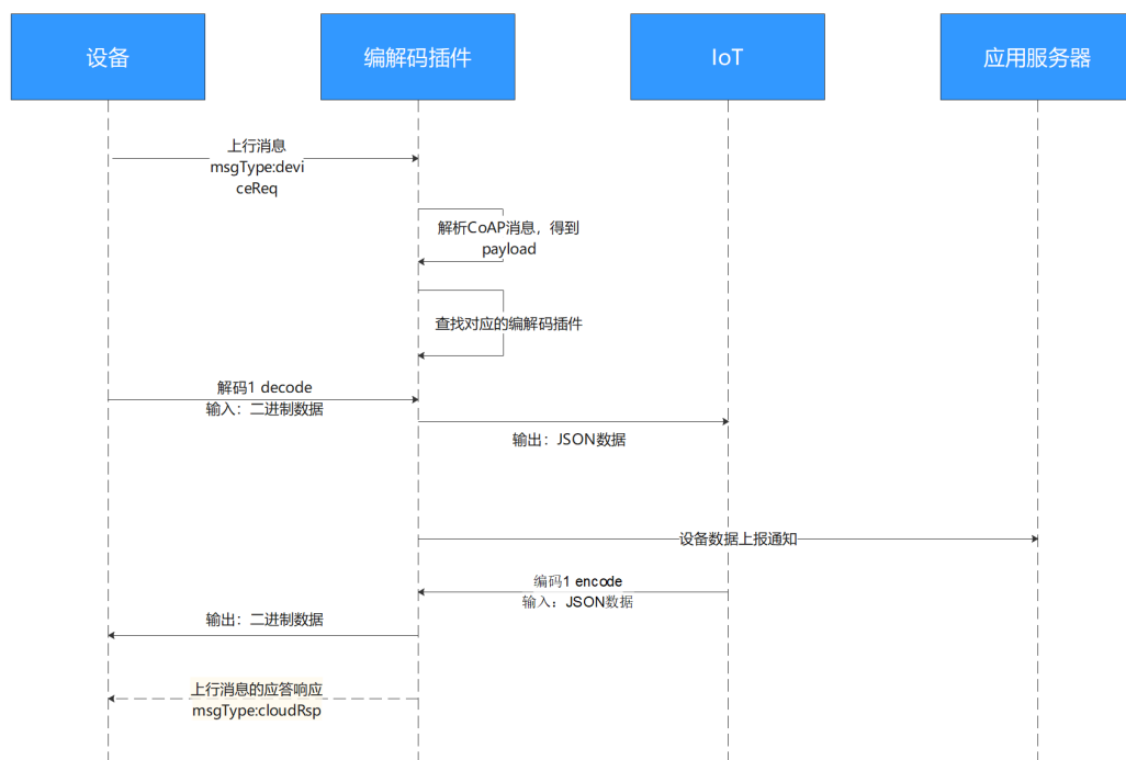
图 3-85 数据上报流程图
