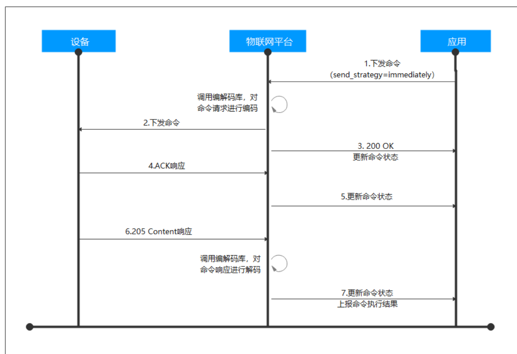
图 3-28 LwM2M/CoAP 命令下发流程
