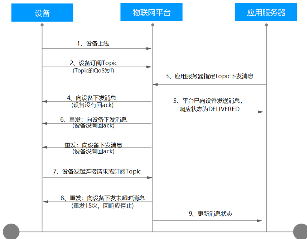
图 3-15 消息下发使用 Qos 1 流程图
