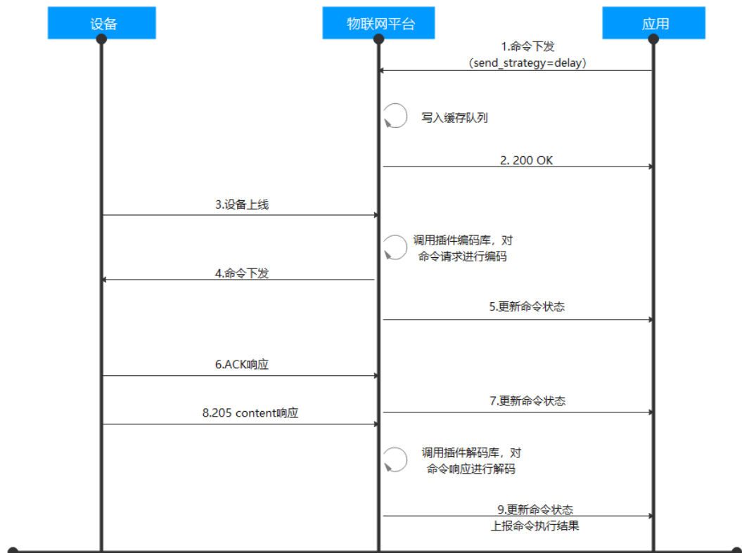
图 3-29 LwM2M/CoAP 命令缓存下发流程
