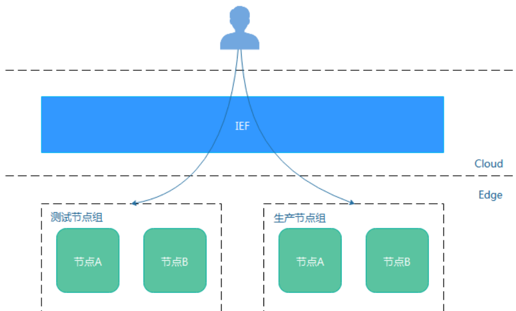
图 4-7 节点组
