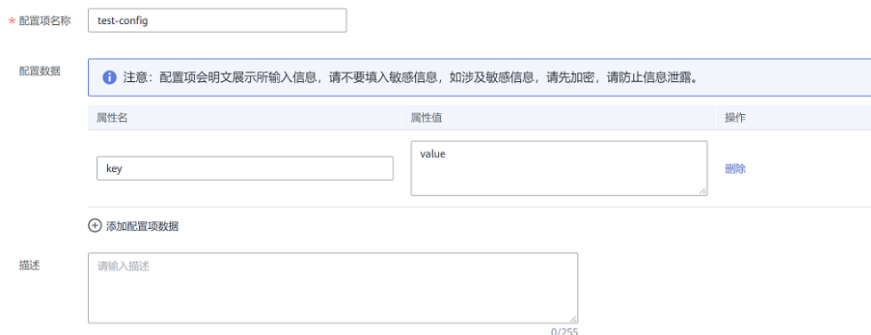
图 4-49 配置项
