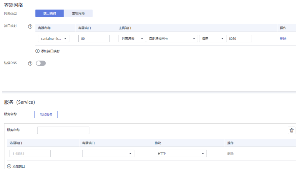
图 4-36 添加服务
