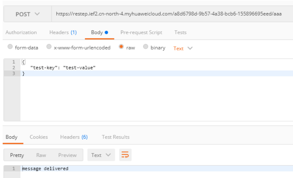
图 4-76 发送消息
