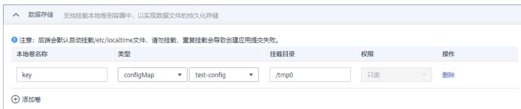
图 3-40 使用 ConfigMap
