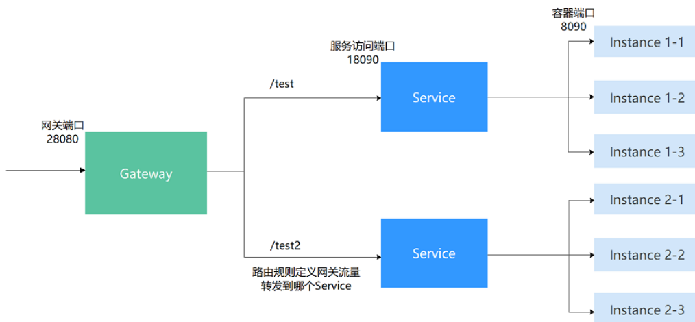
图 4-59 网关流量转发路径示意图
