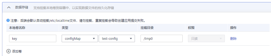
图 4-50 使用 ConfigMap
