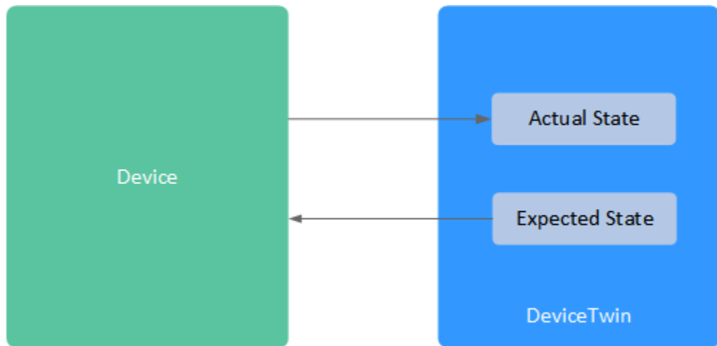
图 3-17 DeviceTwin
