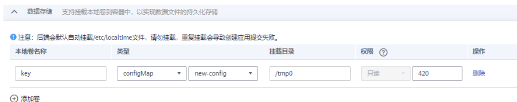
图 3-40 使用 ConfigMap
