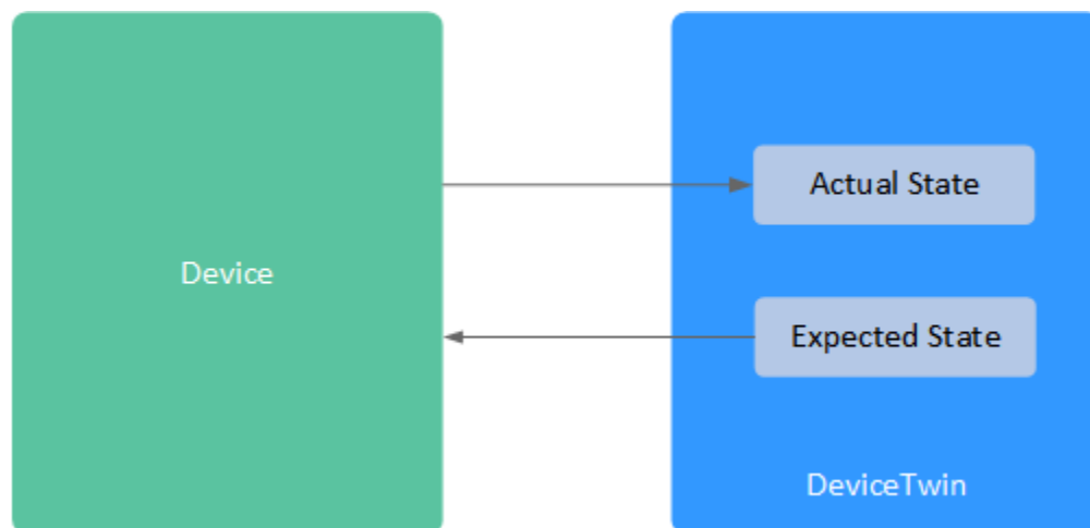
图 4-21 DeviceTwin
