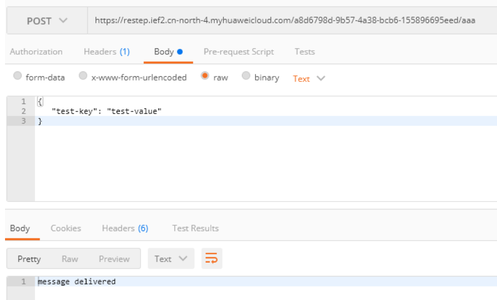
图 3-54 发送消息
