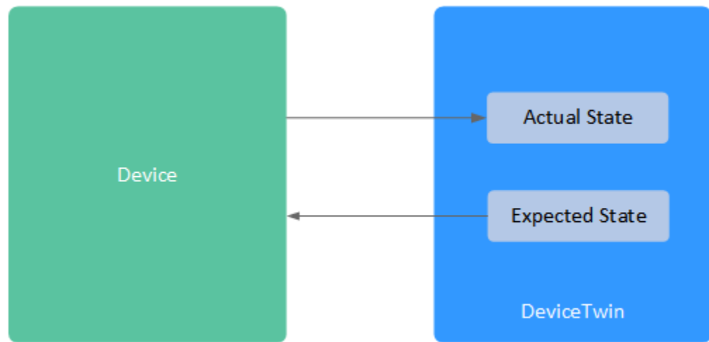
图 4-21 DeviceTwin
