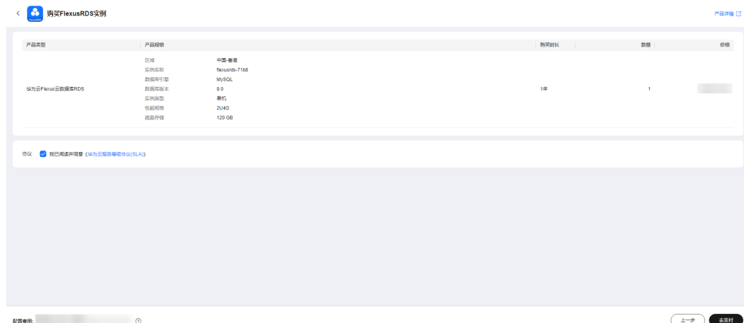
图 3-3 订单确认
