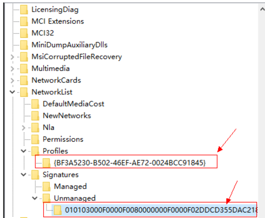
图 2-2 注册表
