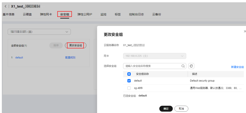
图 2-11 更改安全组
