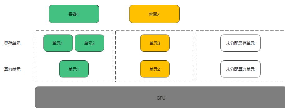
图 11-7 平均调度
