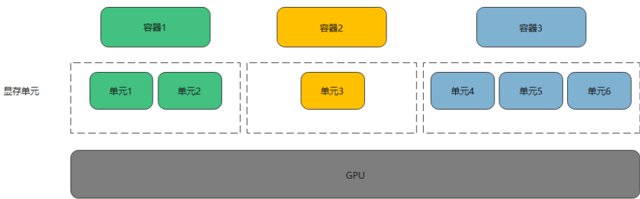
图 11-5 原生调度
