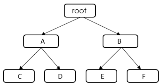
图 10-1 优先级取值
