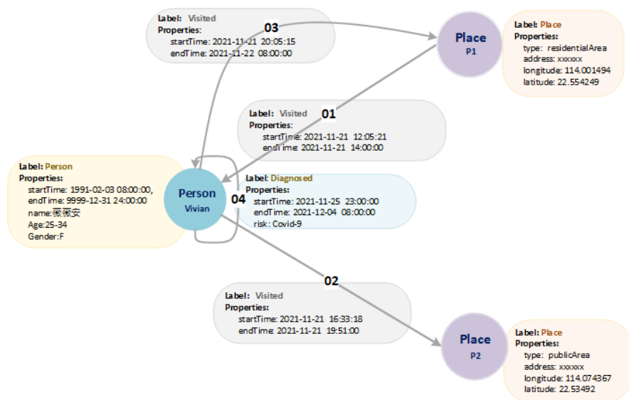
图 4-3 动态图数据示例
