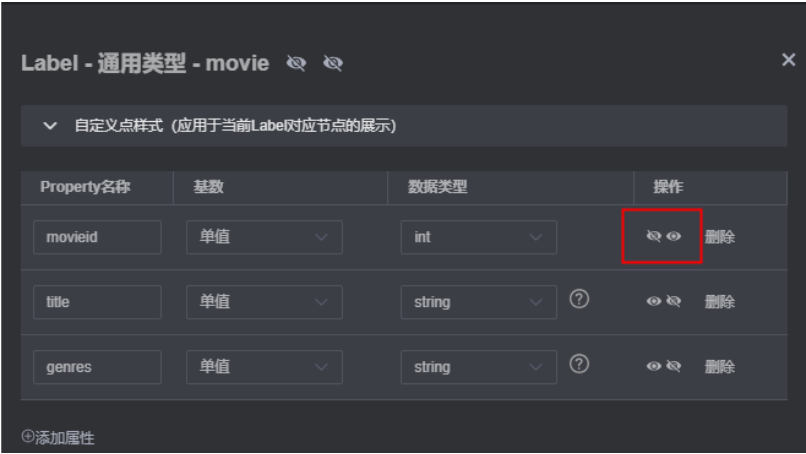
图 8-18 隐藏图属性敏感信息
