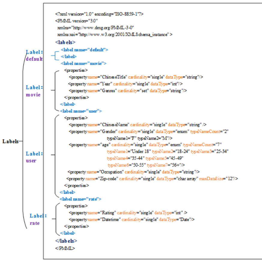
图 4-1 元数据组成结构
