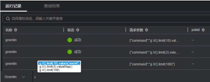
图 8-58 Gremlin 联想查询
