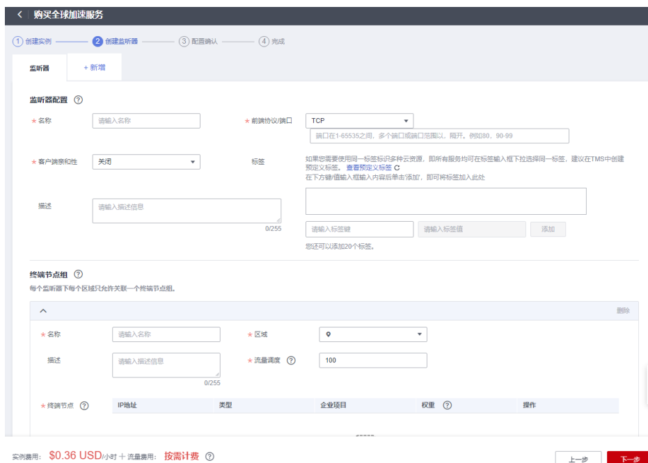
图 1-3 添加监听器
