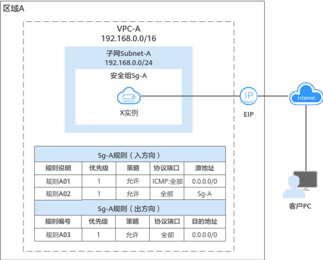
图 9-1 安全组架构图
