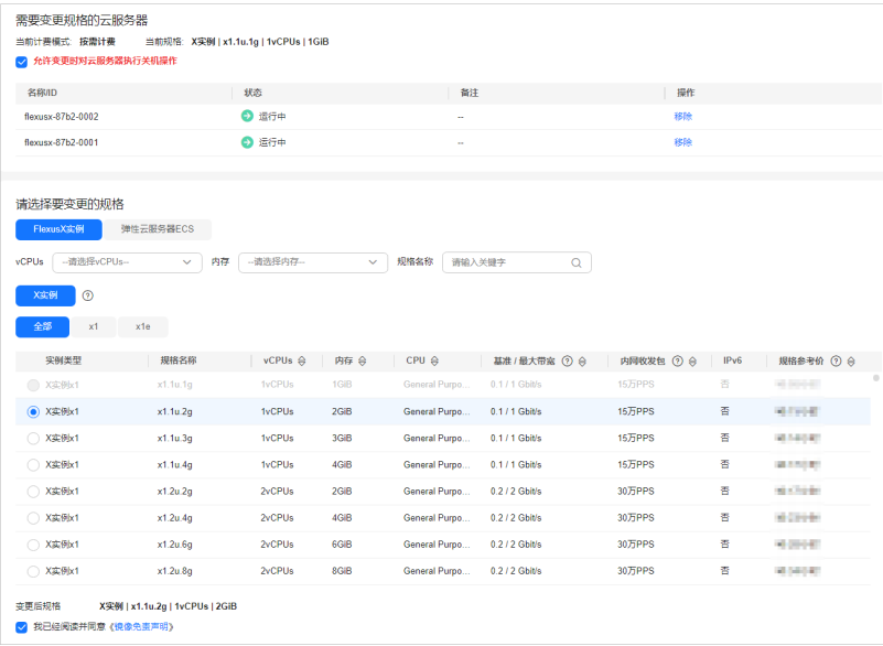
图 4-6 设置批量变更规格
