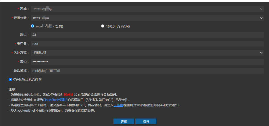
图 3-3 CloudShell 配置向导（公网 IP）
