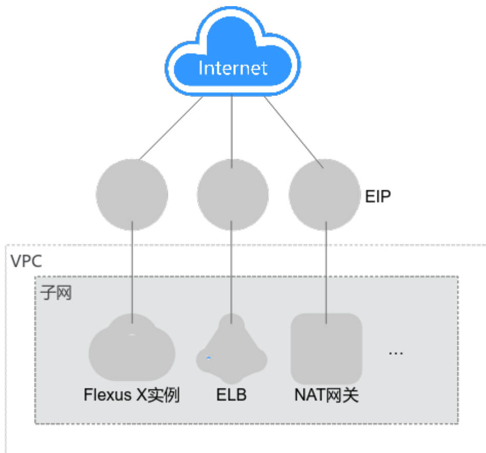
图 8-1 EIP
