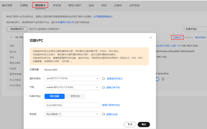
图 7-2 切换 VPC
