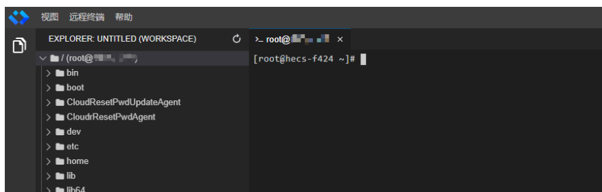
图 3-8 操作结果
