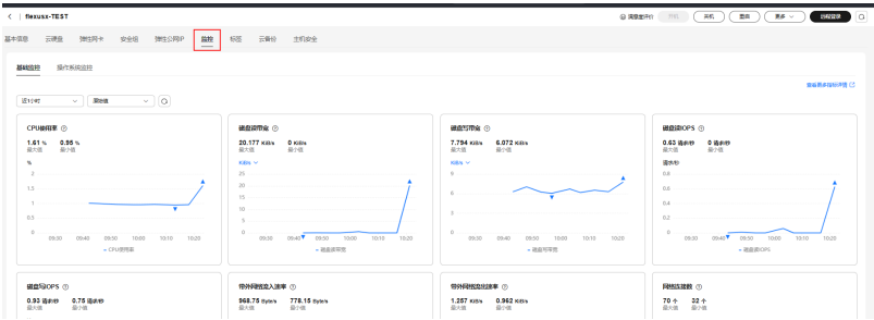
图 11-2 查看监控
