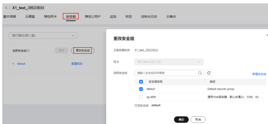
图 9-3 更改安全组
