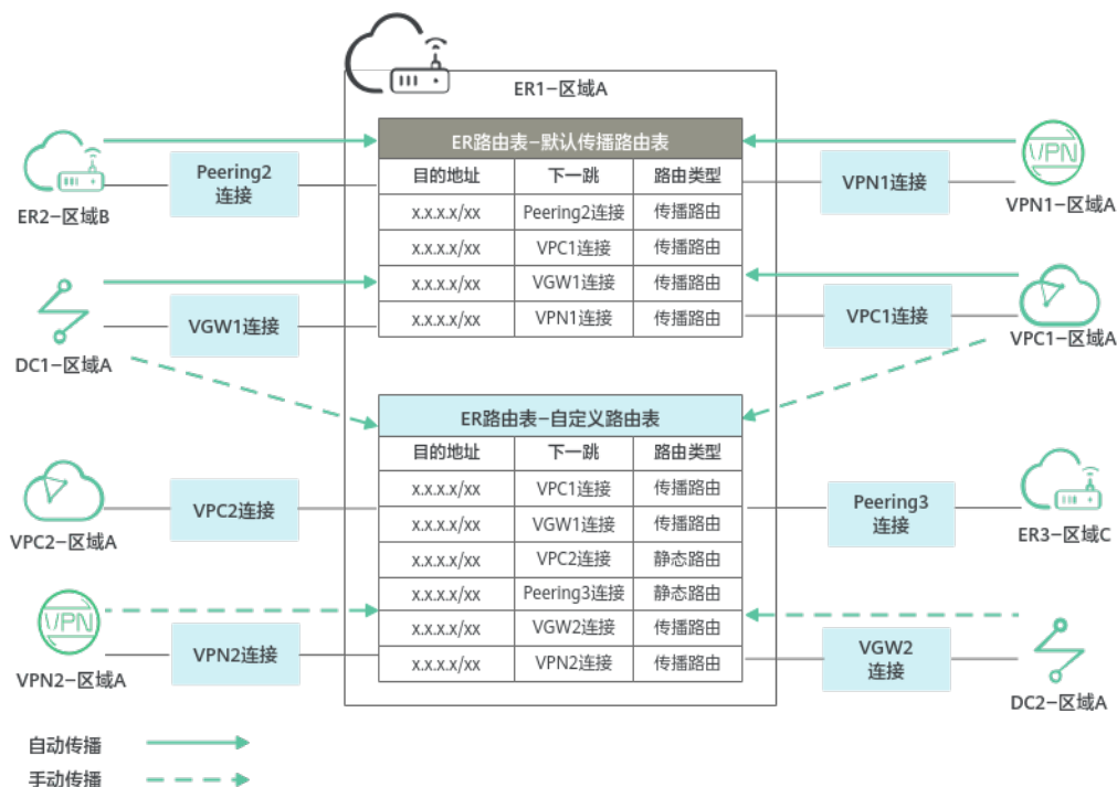
图 5-1 传播路由和静态路由概述
