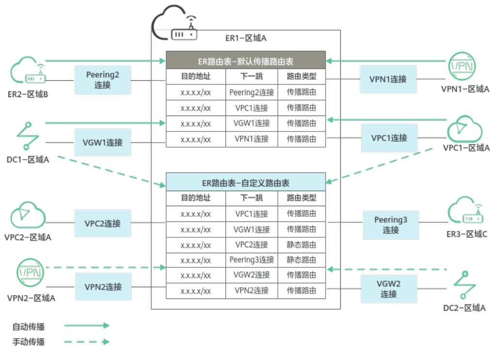
图 6-1 传播路由和静态路由概述
