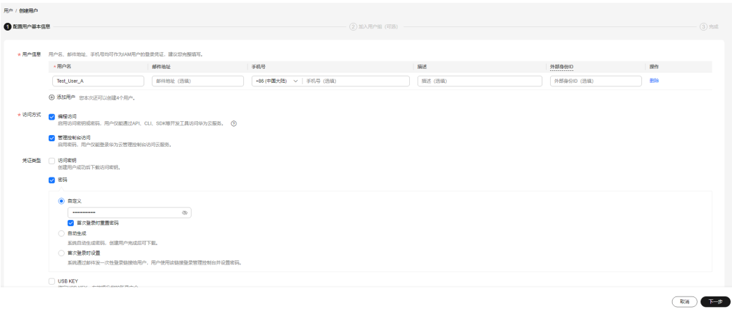
图 2-13 配置用户基本信息
