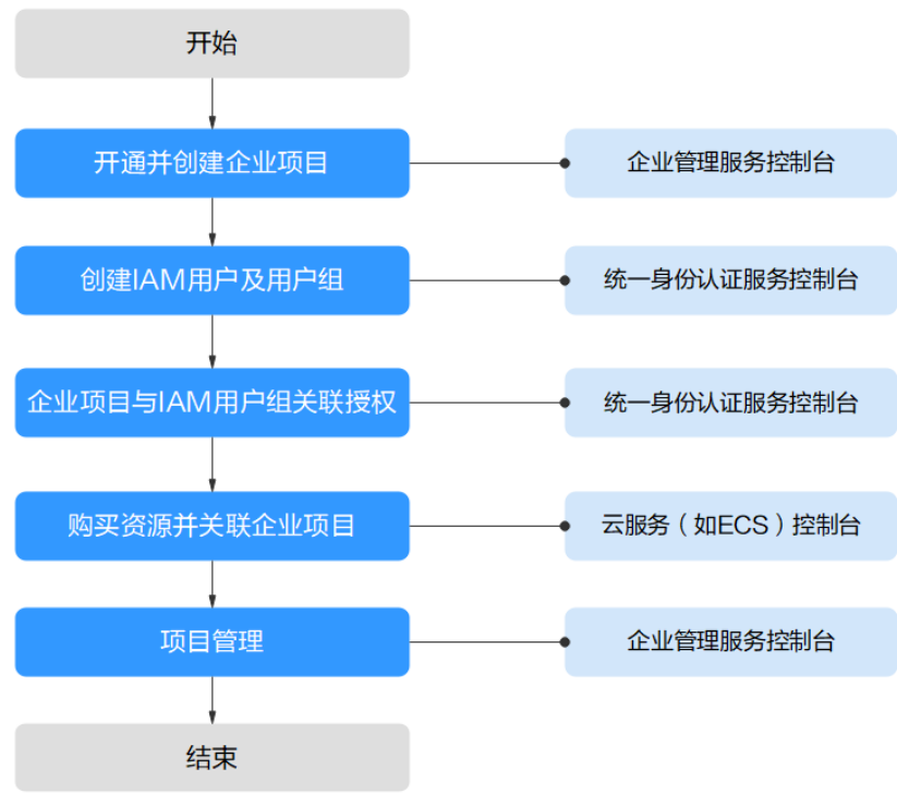
图 2-24 企业项目管理流程图
