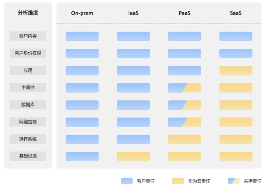
图 2-5 华为云安全责任共担模型
