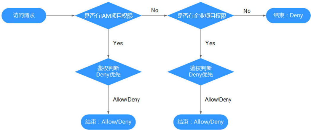
图 2-77 请求鉴权逻辑图
