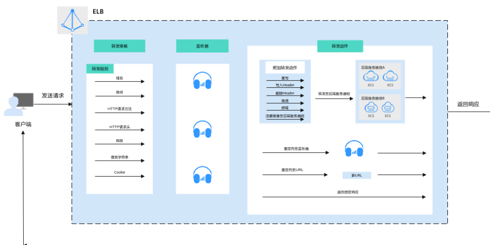
图 1-15 高级转发策略（独享型）示意图
