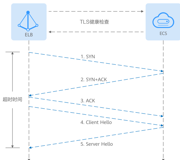
图 1-33 TLS 健康检查
