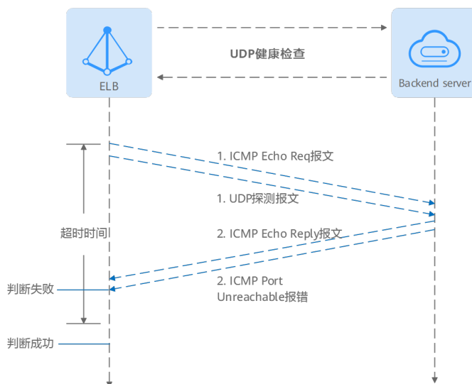
图 1-30 UDP 健康检查
