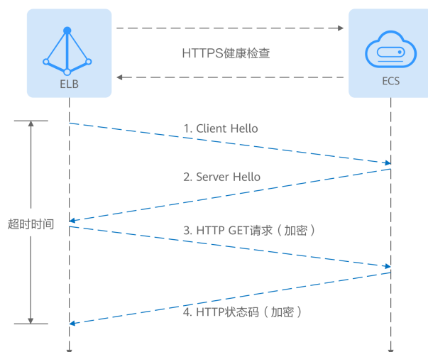
图 1-32 HTTPS 健康检查
