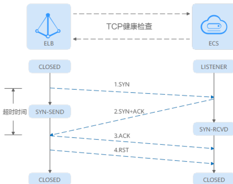
图 1-29 TCP 健康检查
