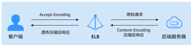
图 1-17 后端服务器进行压缩示意图
