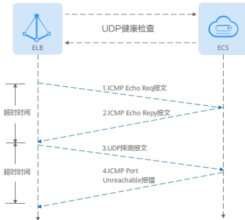
图 2-15 UDP 健康检查
