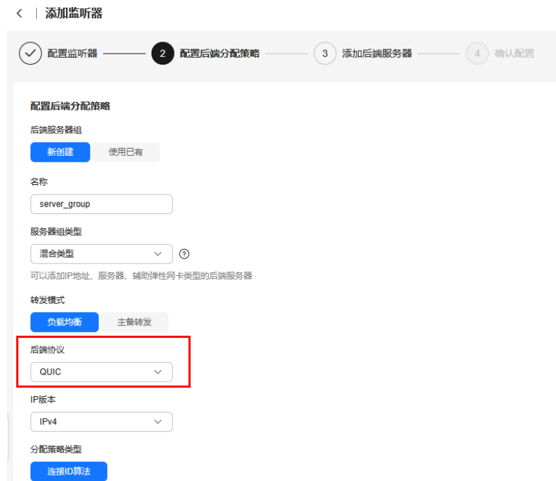
图 1-14 后端协议选择“QUIC”
