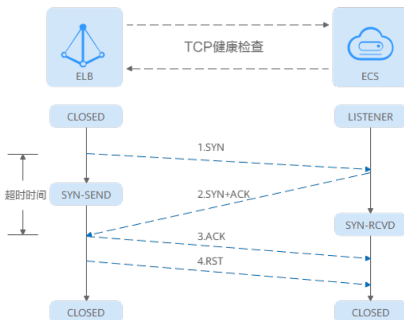
图 2-14 TCP 健康检查
