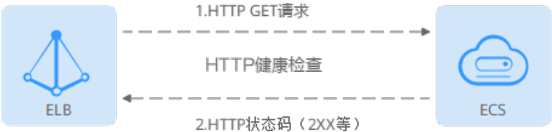
图 2-15 HTTP 健康检查
