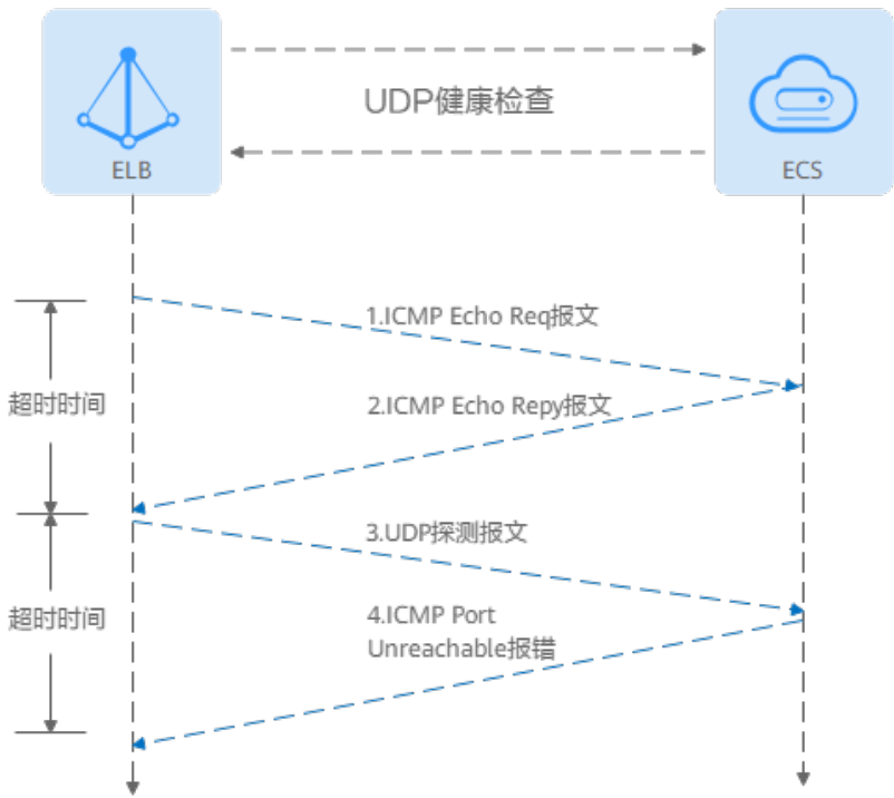
图 2-14 UDP 健康检查
