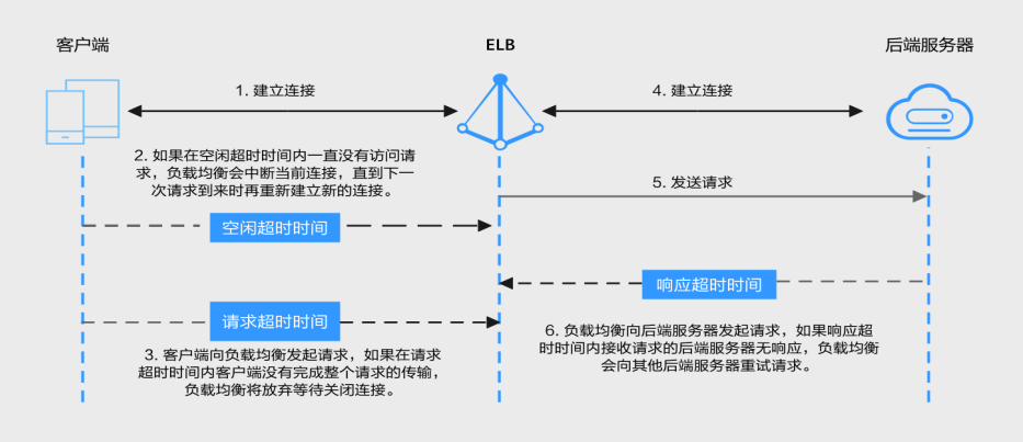
图 1-12 七层监听器超时时间示意图
