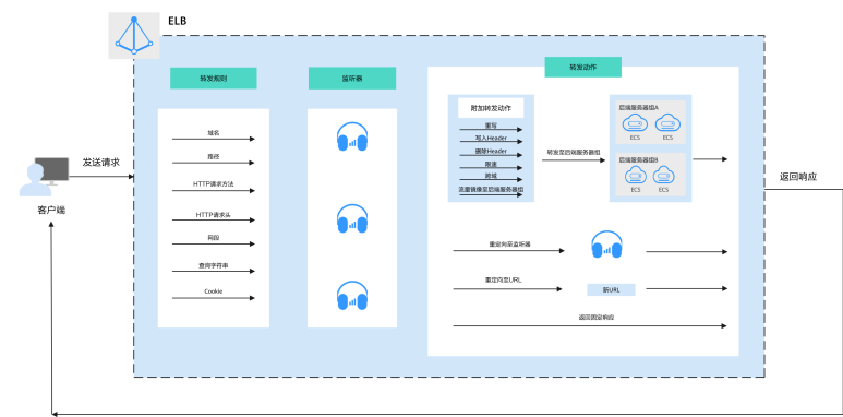
图 1-15 高级转发策略（独享型）示意图
