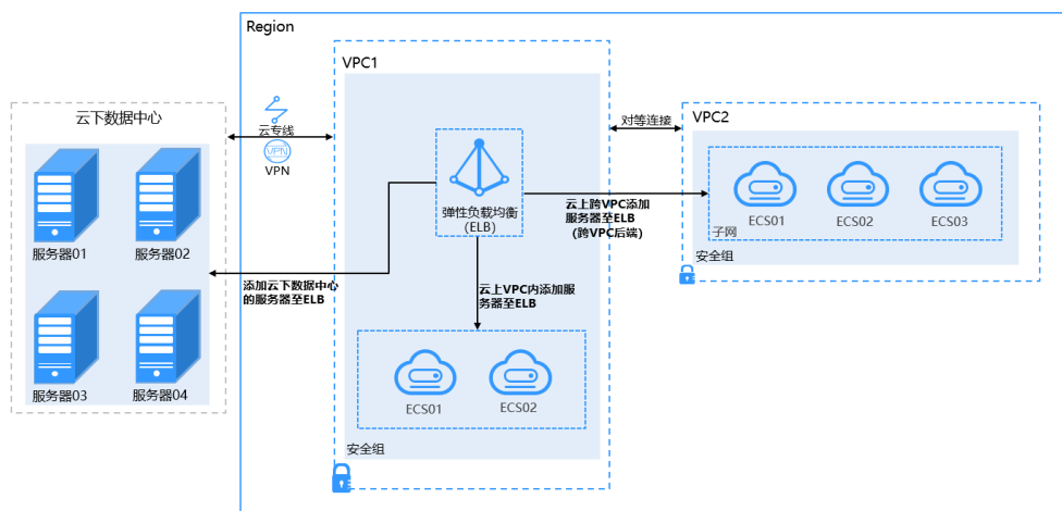
图 1-27 ELB 支持添加云上、云下的服务器
