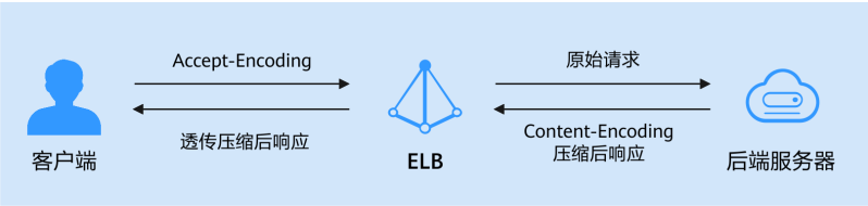
图 1-17 后端服务器进行压缩示意图
