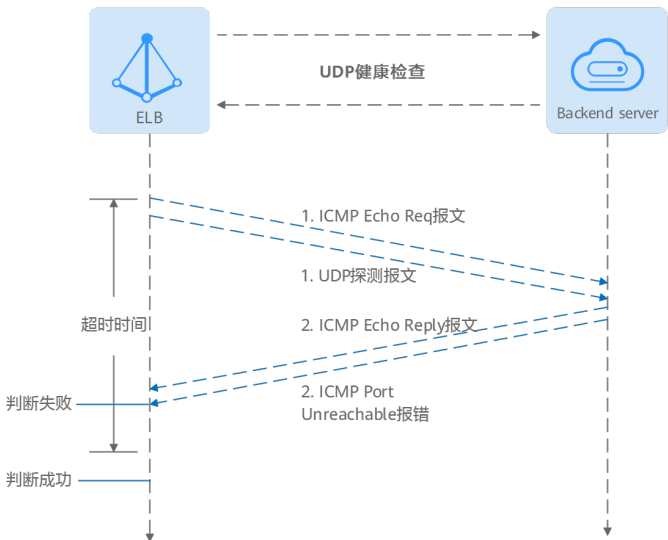
图 1-29 UDP 健康检查
