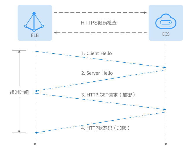
图 1-31 HTTPS 健康检查
