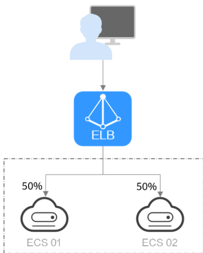
图 1-22 加权轮询算法流量分发
