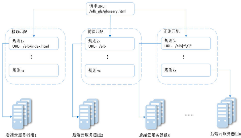
图 2-7 转发示例
