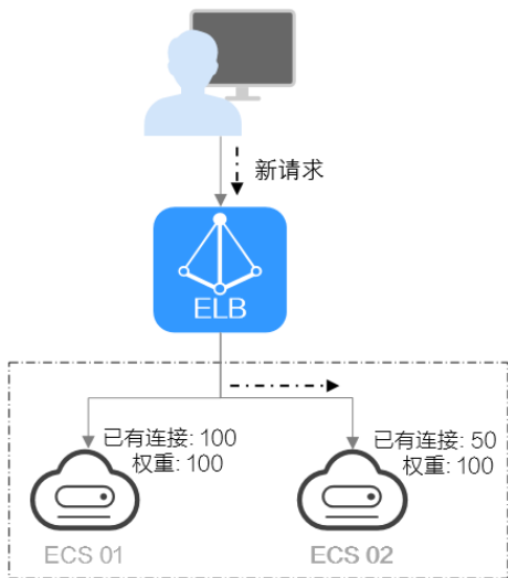
图 1-23 加权最少连接算法流量分发
