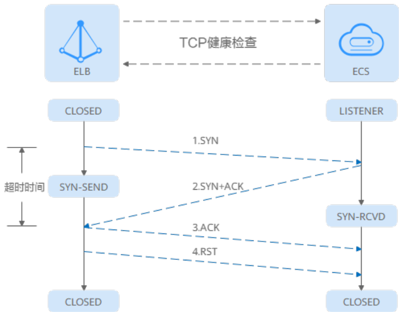
图 2-13 TCP 健康检查
