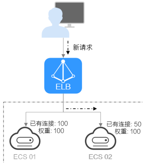
图 2-10 加权最少连接算法流量分发
