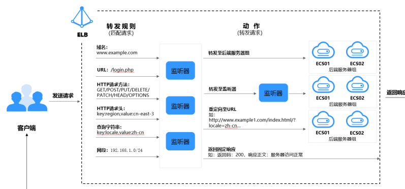
图 1-8 高级转发策略（独享型）示意图
