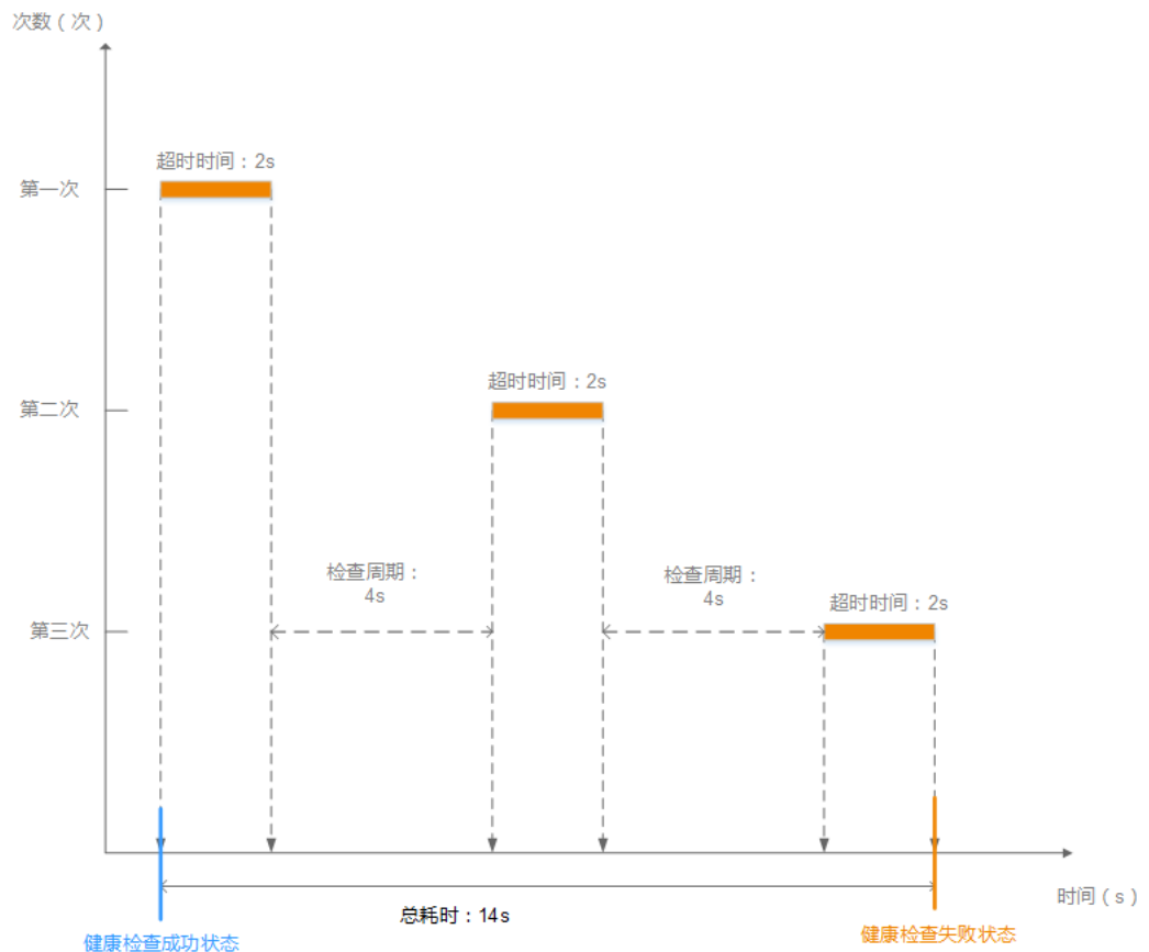
图 1-16 健康检查失败时间窗
