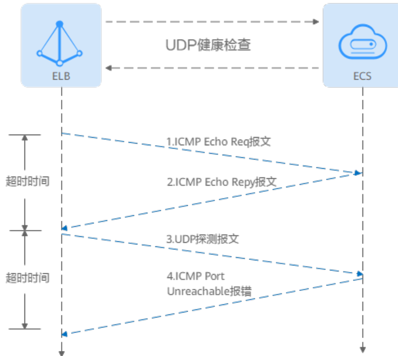
图 1-12 UDP 健康检查
