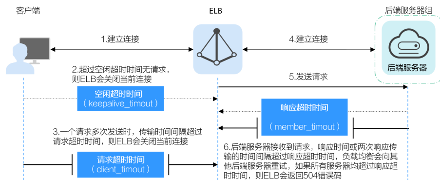
图 1-8 七层监听器超时时间示意图
