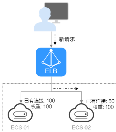
图 1-18 加权最少连接算法流量分发
