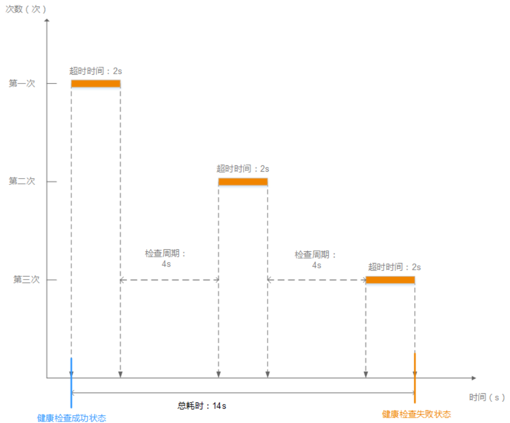
图 2-10 健康检查失败时间窗
