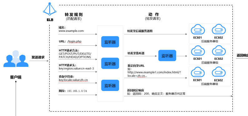
图 3-2 高级转发策略（独享型）示意图
