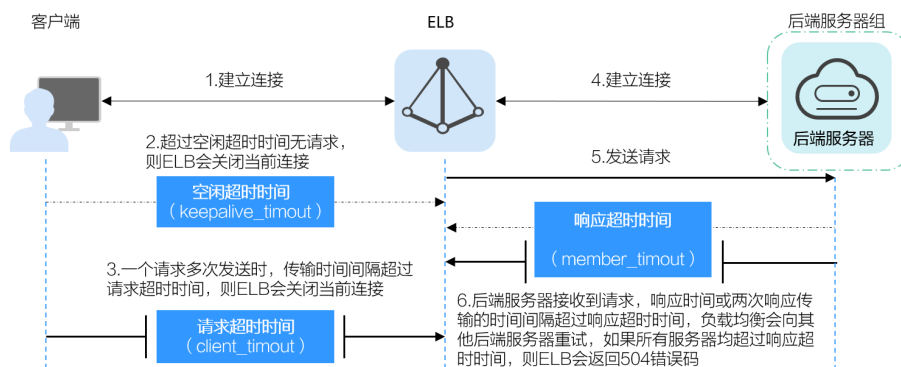
图 2-1 七层监听器超时时间示意图
