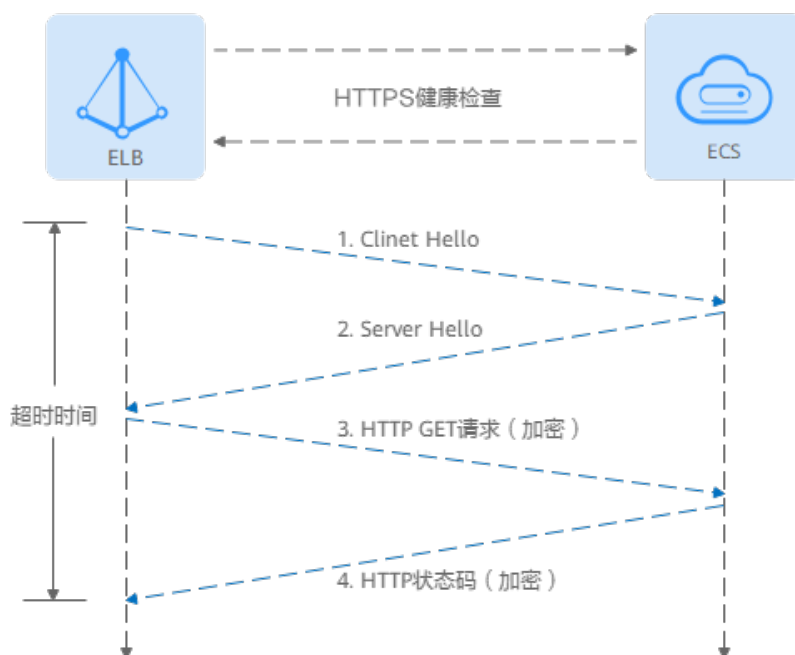
图 4-5 HTTPS 健康检查
