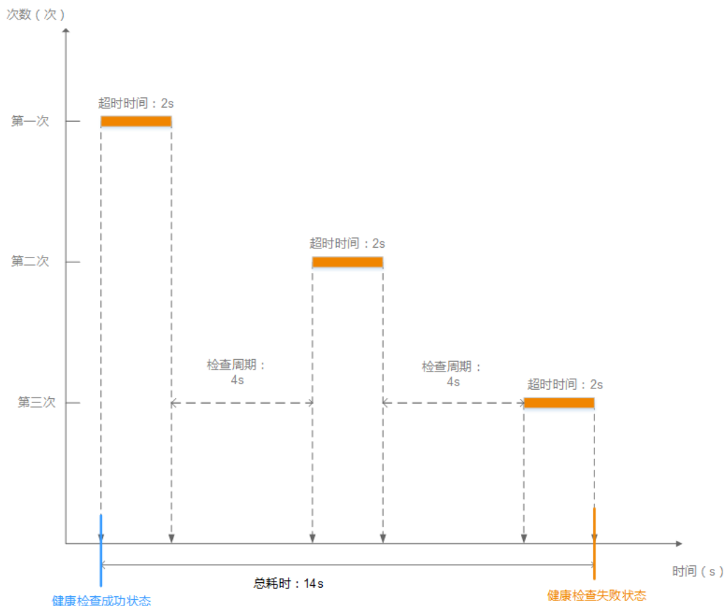
图 4-6 健康检查失败时间窗
