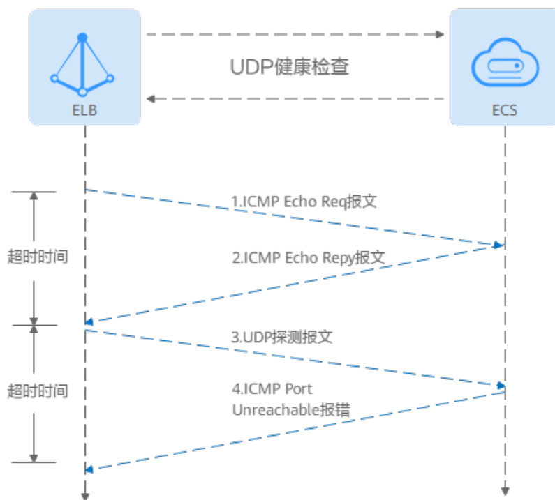
图 4-3 UDP 健康检查
