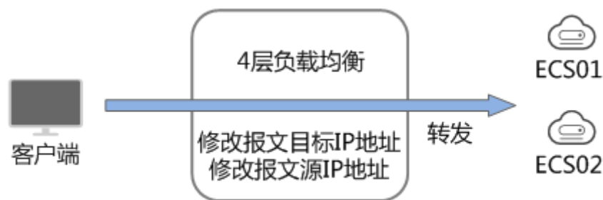
图 1-3 四层负载均衡
