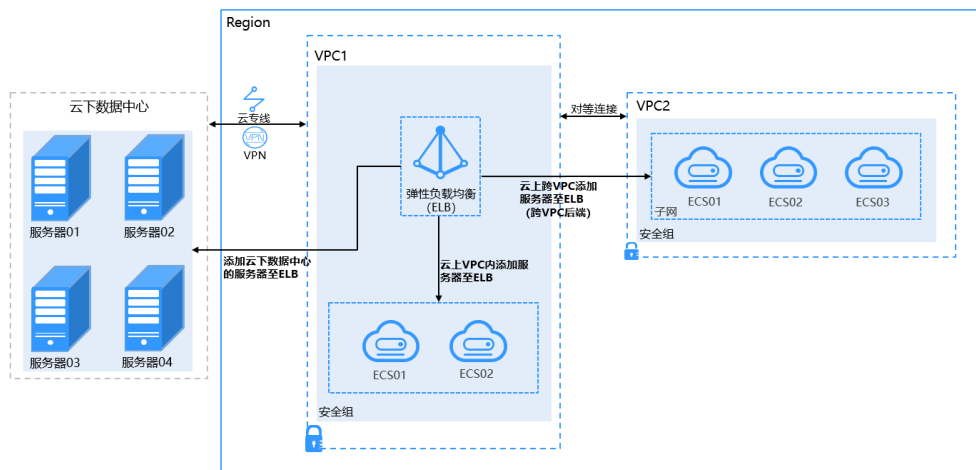
图 5-1 ELB 支持添加云上、云下的服务器
