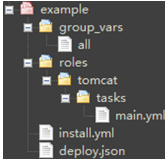
图 3-9 文件架构
