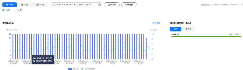
图 8-122 慢日志趋势
