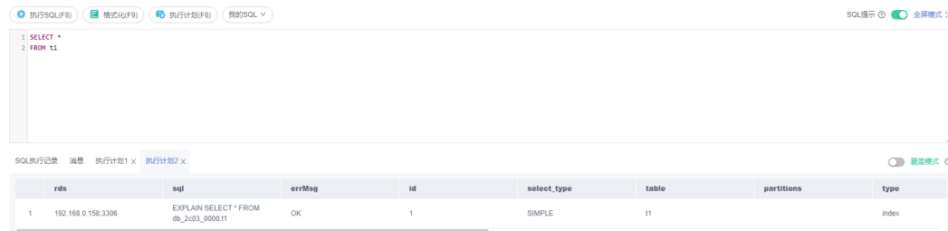
图 12-5 执行计划
