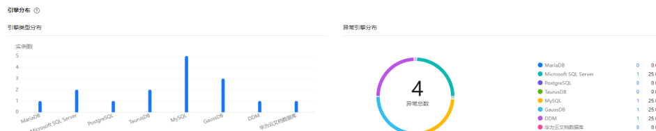
图 3-145 引擎分布
