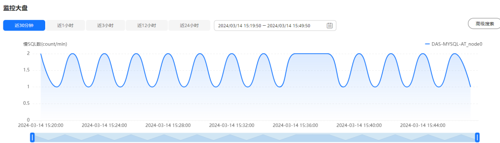
图 8-102 监控大盘
