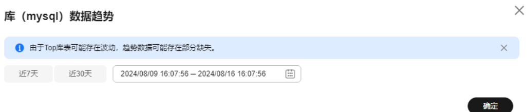
图 3-214 查看趋势
