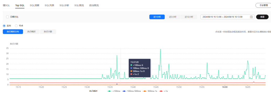
图 12-26 TOP SQL
