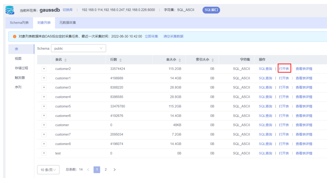
图 10-10 打开表
