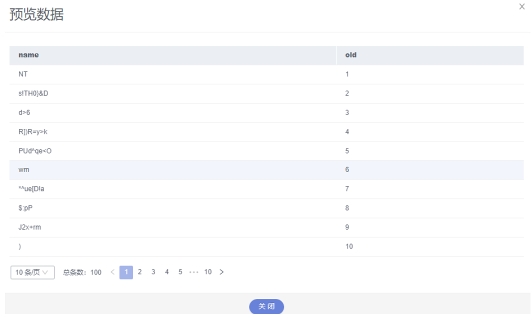
图 6-126 数据预览
