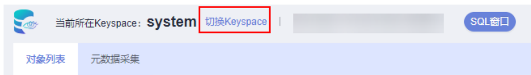
图 9-14 切换 Keyspace
