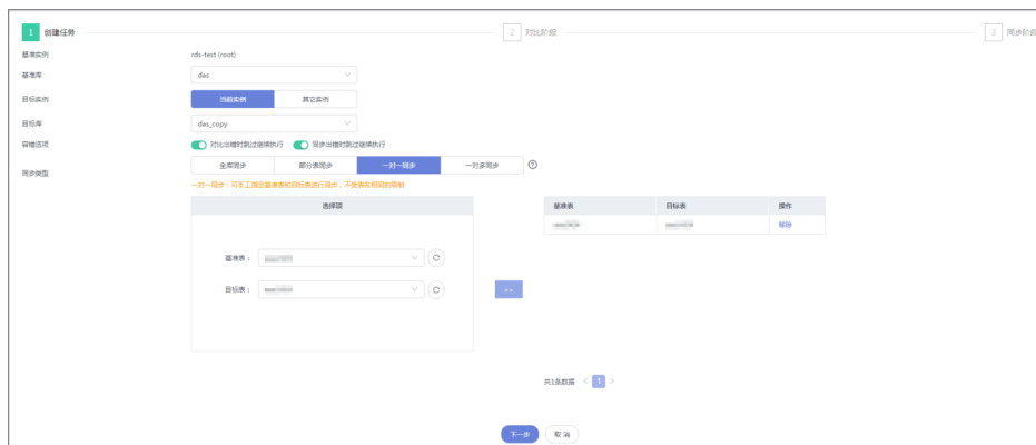
图 8-95 创建任务
