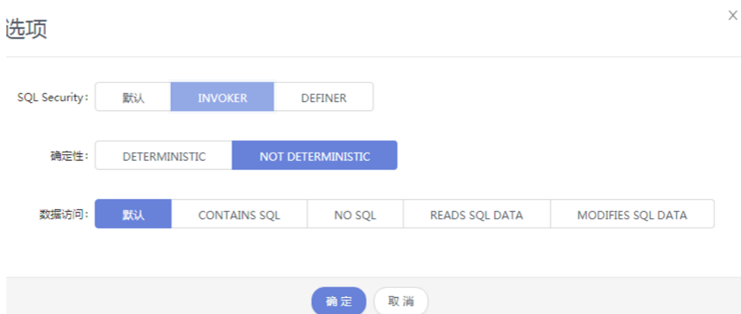
图 8-53 选项界面
