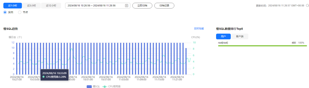
图 5-48 慢日志趋势
