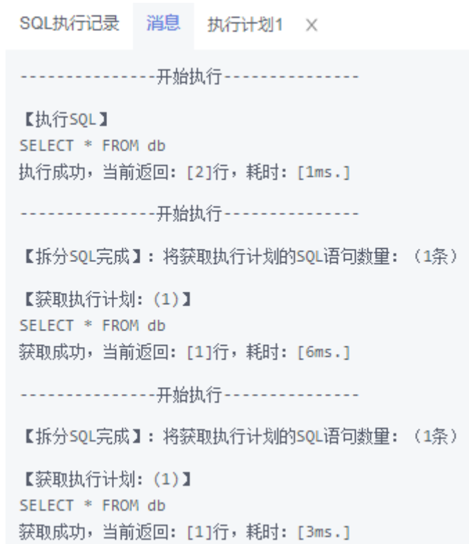
图 6-17 查看消息
