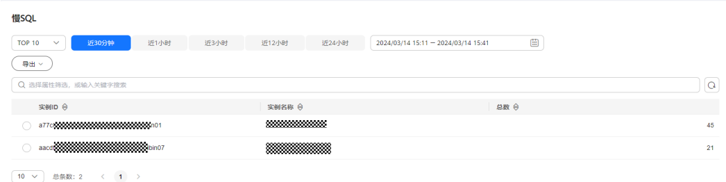
图 6-155 慢 SQL
