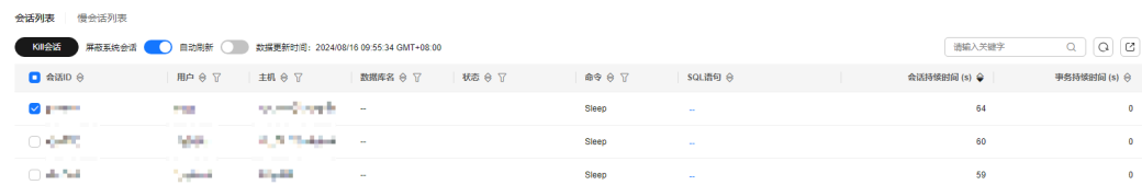
图 8-119 Kill 会话
