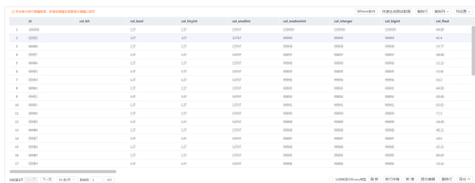
图 8-26 表编辑页面
