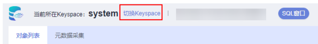
图 9-17 切换 Keyspace
