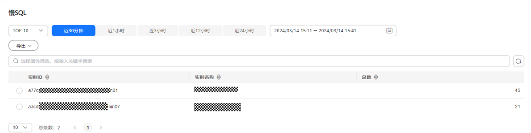
图 8-101 慢 SQL
