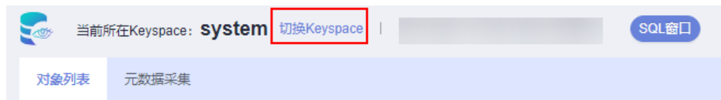
图 9-15 切换 Keyspace
