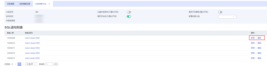
图 3-125 管理 SQL
