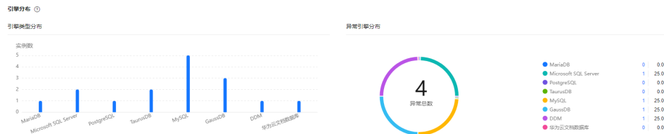
图 12-13 引擎分布
