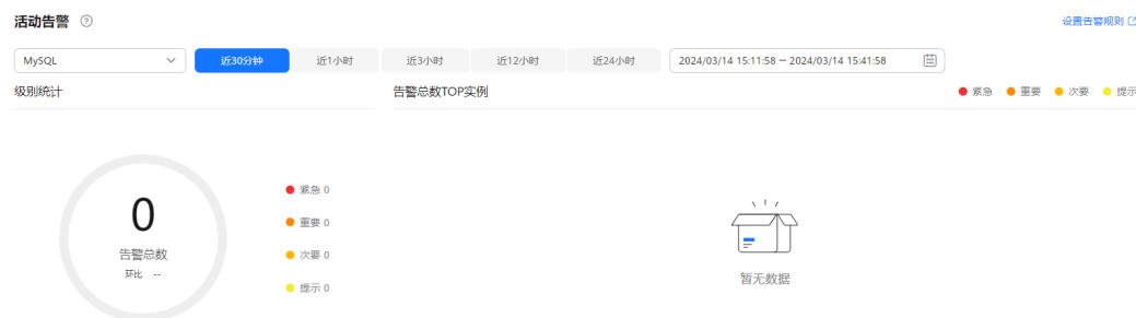
图 3-146 活动告警
