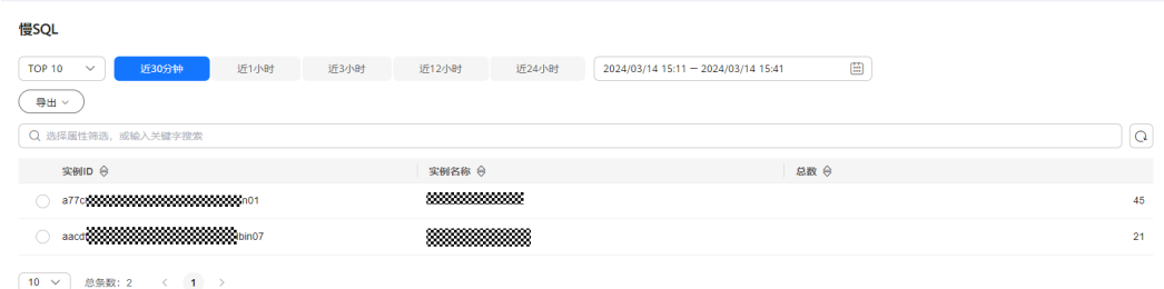
图 7-45 慢 SQL
