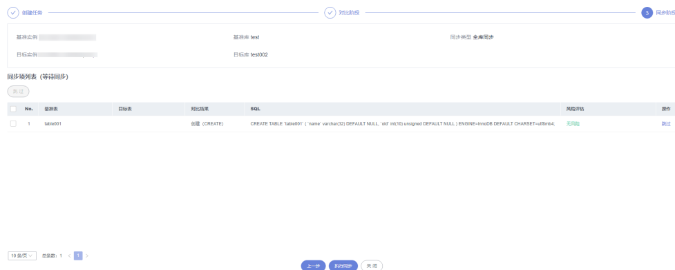
图 3-143 执行同步
