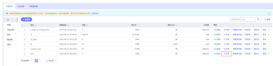
图 8-25 打开表
