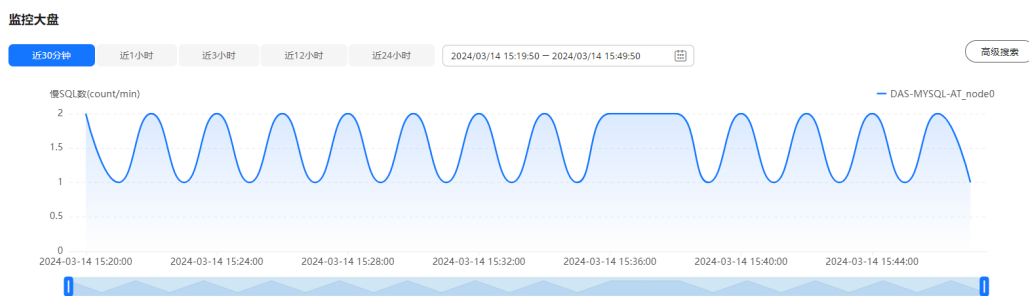
图 7-46 监控大盘
