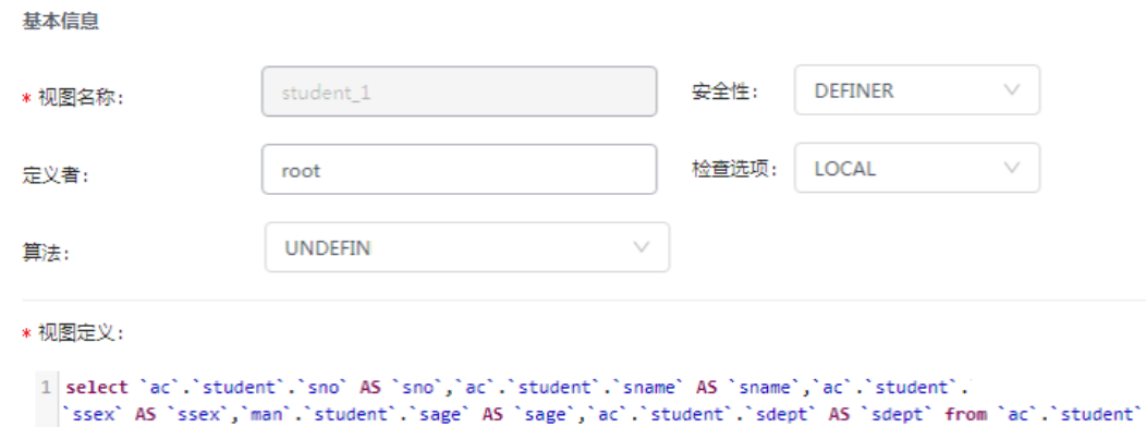
图 8-41 编辑视图
