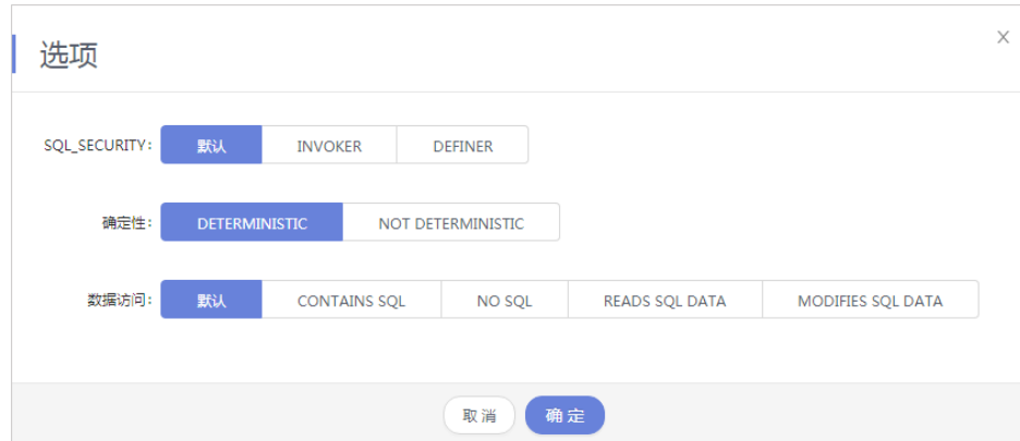
图 3-89 选项
