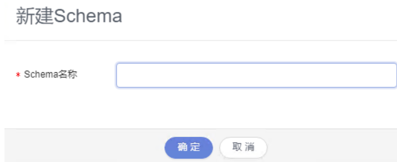
图 7-6 新建 Schema
