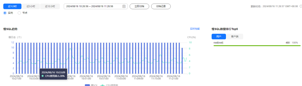
图 3-177 慢日志趋势
