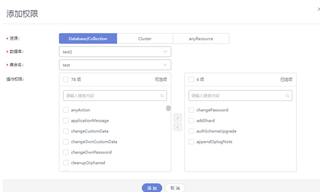
图 11-6 添加权限
