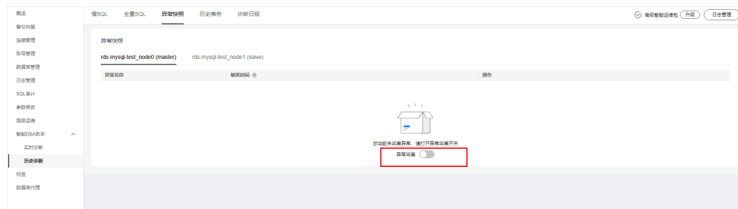
图 3-230 异常快照
