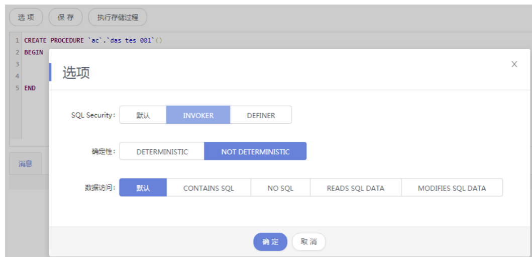
图 6-68 选项页面
