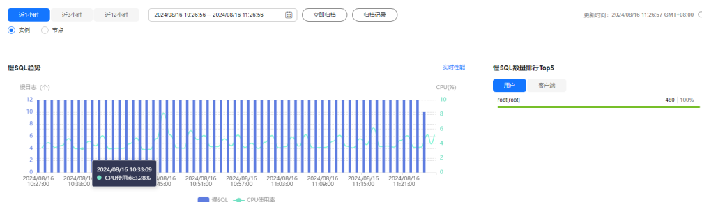
图 6-180 慢日志趋势
