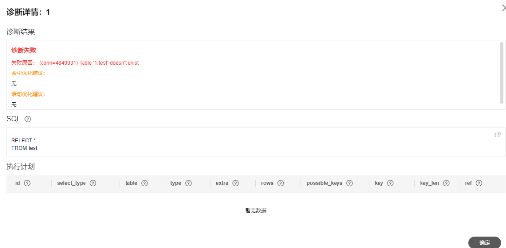
图 3-196 SQL 诊断
