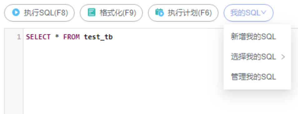
图 4-21 我的 SQL
