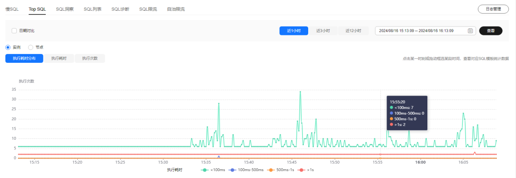
图 7-51 查看特定时间点的 TOP SQL 列表
