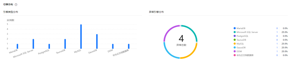
图 8-99 引擎分布
