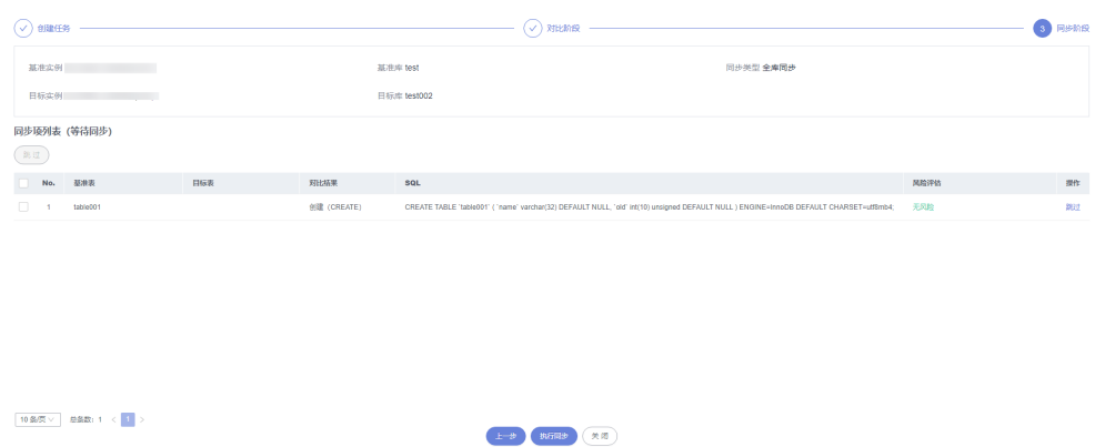
图 3-143 执行同步
