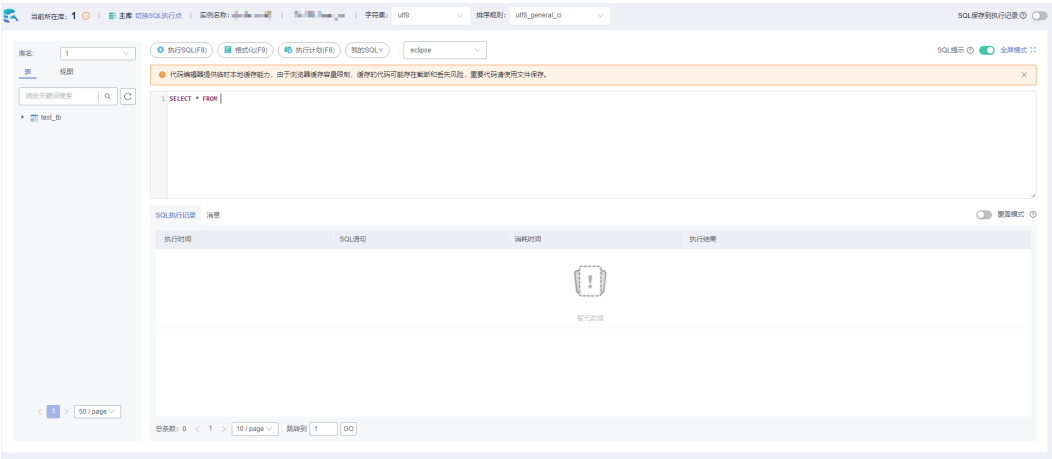
图 3-9 SQL 窗口
