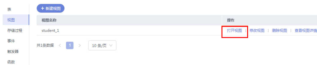
图 8-38 打开视图
