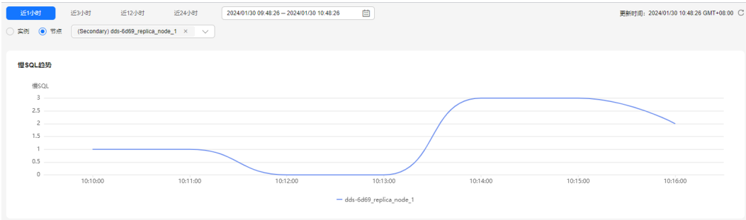
图 11-32 慢 SQL 趋势
