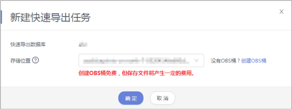
图 5-36 快速导出
