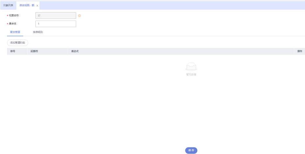
图 11-27 修改视图
