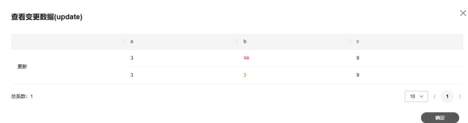
图 3-195 查看数据
