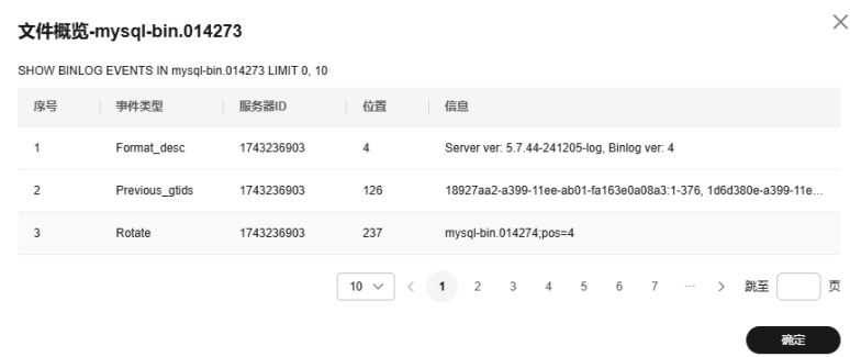
图 3-200 查看概览
