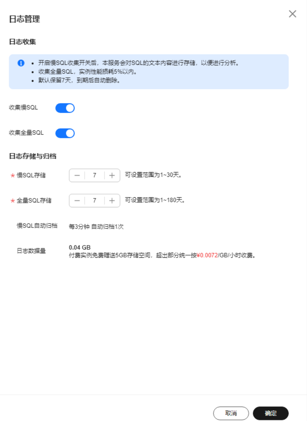
图 3-179 日志管理
