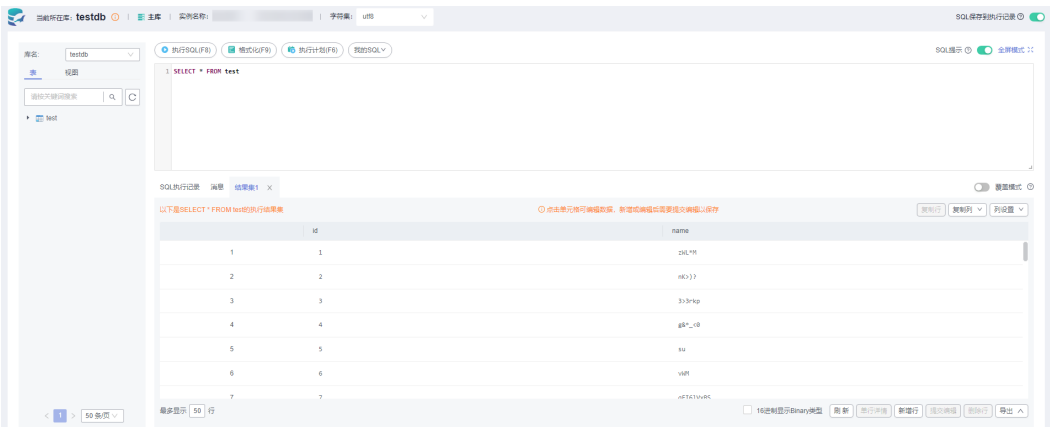
图 6-11 SQL 窗口
