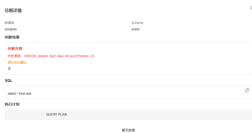
图 5-48 SQL 诊断
