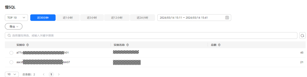
图 4-99 慢 SQL
