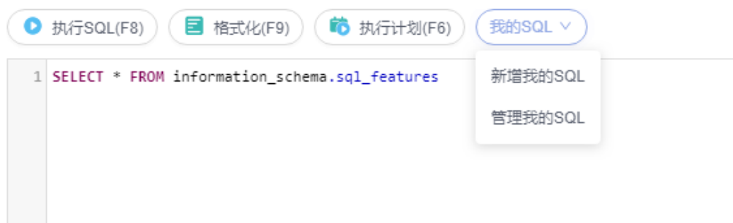
图 5-16 我的 SQL
