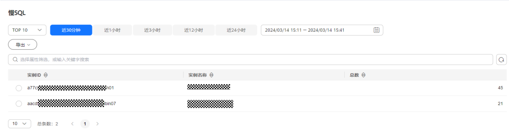
图 12-14 慢 SQL
