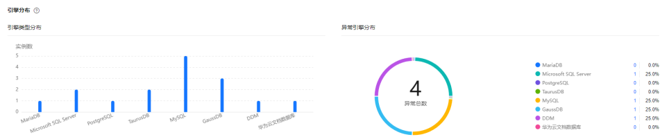
图 4-97 引擎分布
