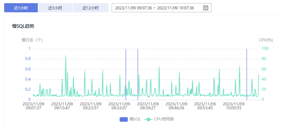
图 4-113 慢 SQL 趋势
