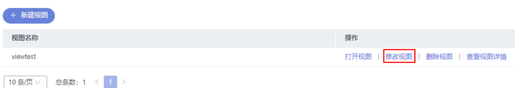
图 6-59 修改视图
