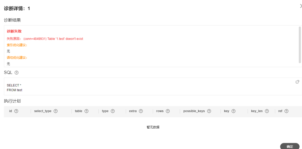
图 3-182 SQL 诊断
