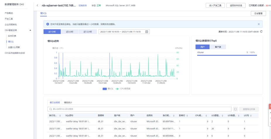
图 4-112 慢 SQL
