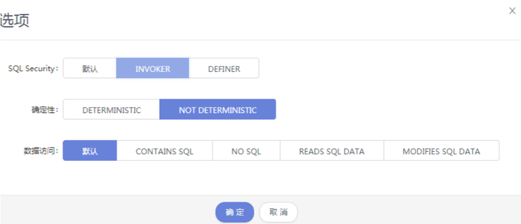
图 8-53 选项界面
