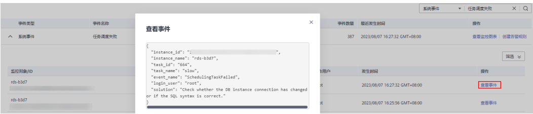
图 14-2 查看事件
