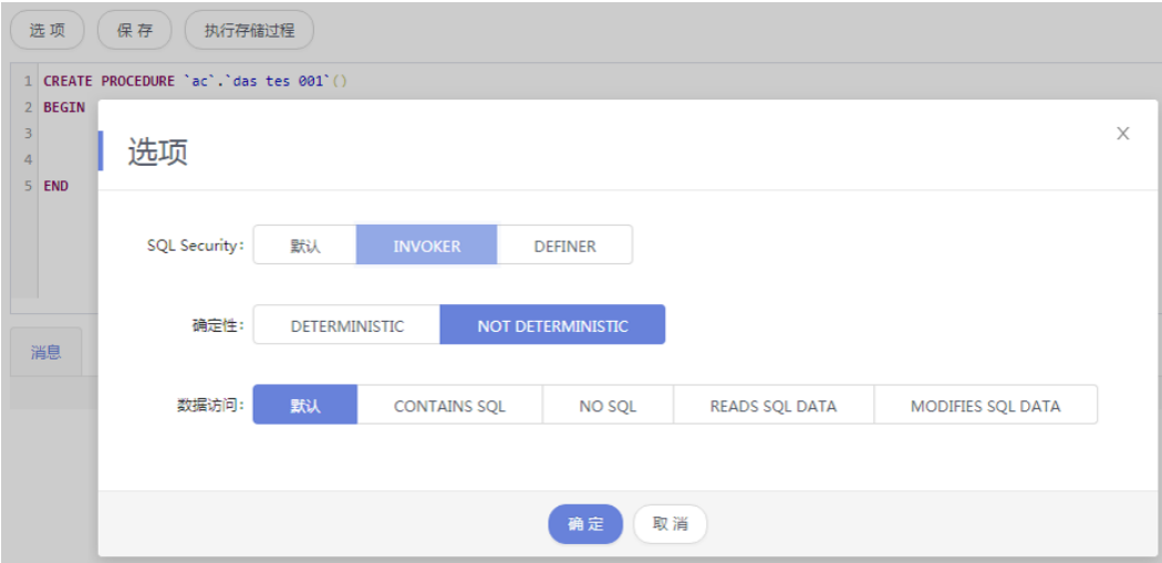
图 6-68 选项页面
