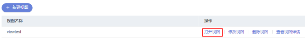
图 6-56 打开视图
