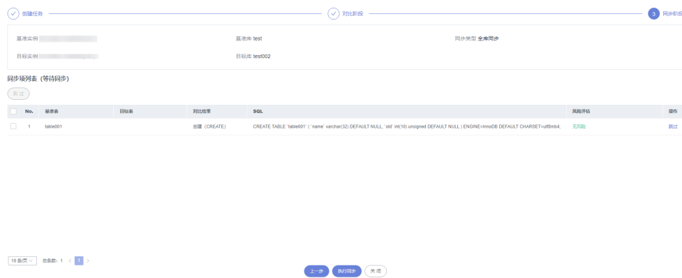
图 6-151 执行同步
