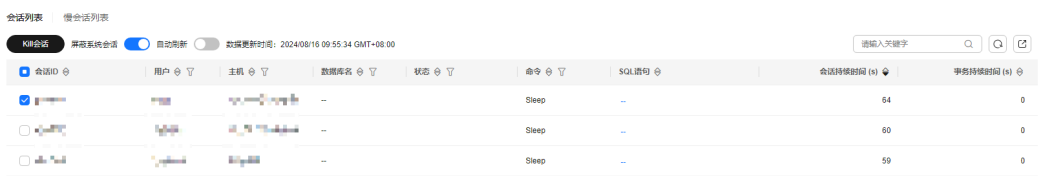
图 8-110 Kill 会话
