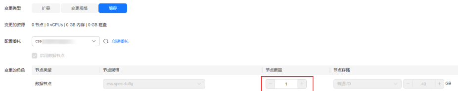
图 2-29 集群缩容
