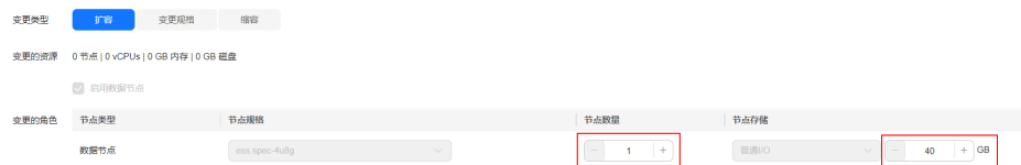
图 3-20 集群扩容
