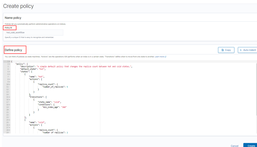
图 3-40 配置策略
