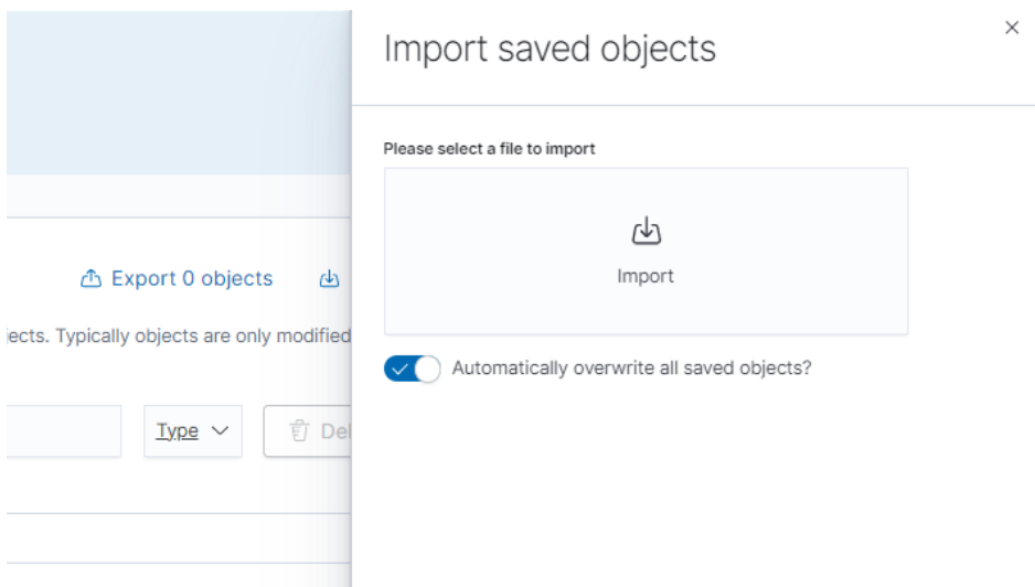
图 2-58 上传文件
