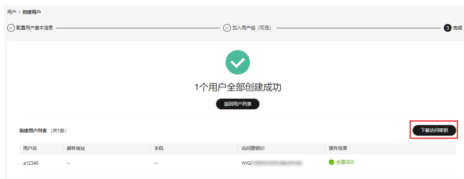
图 1-4 创建成功
