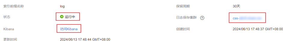
图 3-55 日志采集
