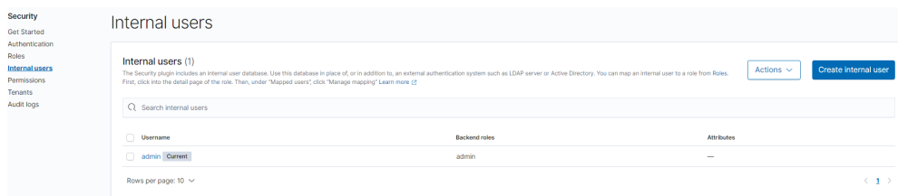
图 3-27 创建用户
