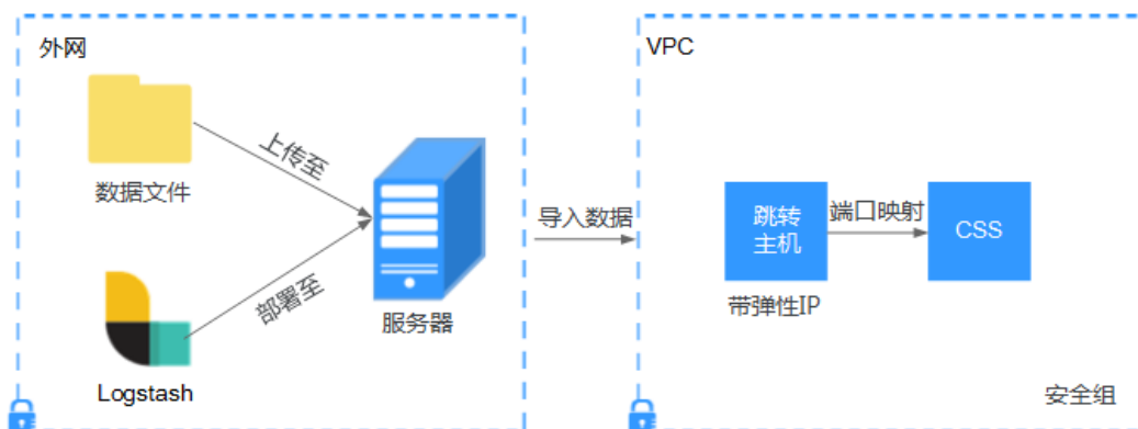
图 2-11 Logstash 部署在外网时导入数据示意图
