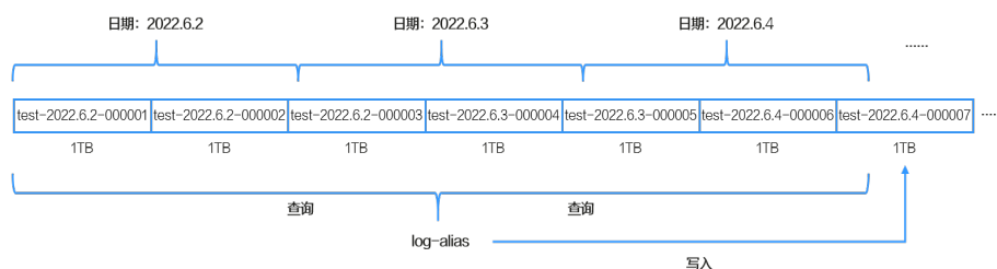
图 2-46 log-alias 的组织形态
