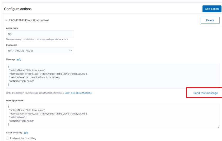
图 2-62 发送验证信息
