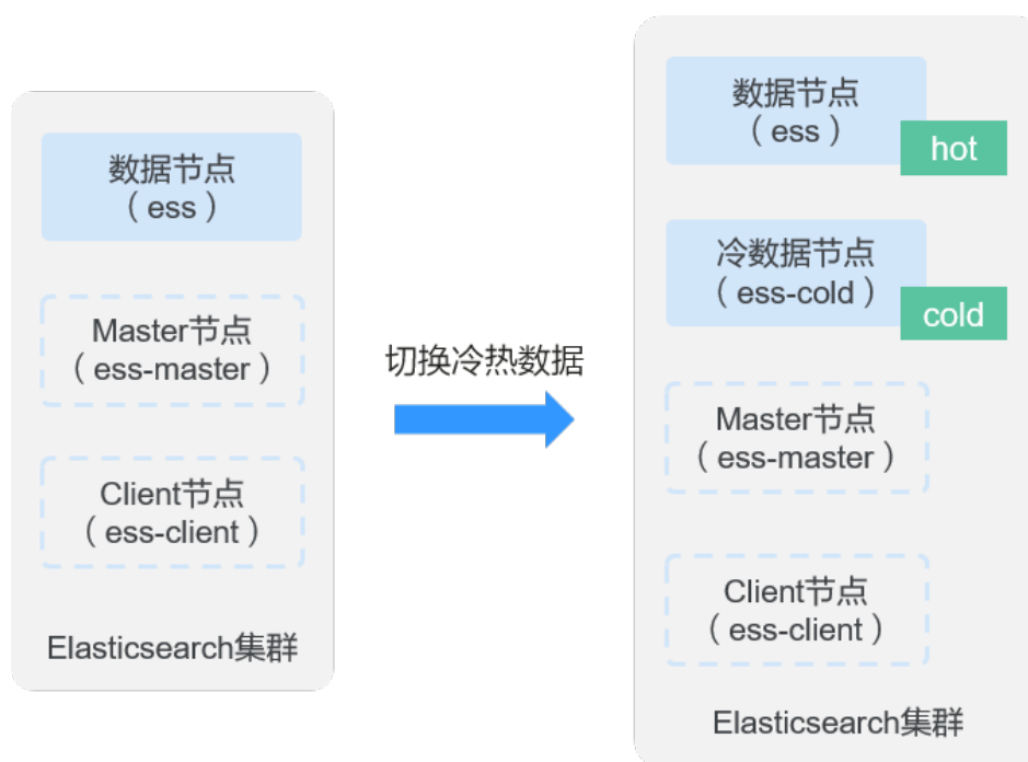
图 3-11 切换冷热数据原理
