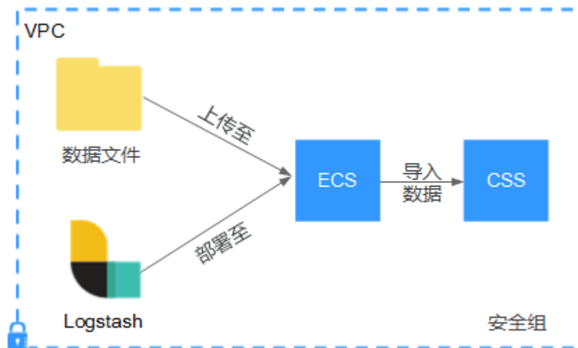
图 3-7 Logstash 部署在弹性云服务器上时导入数据示意图
