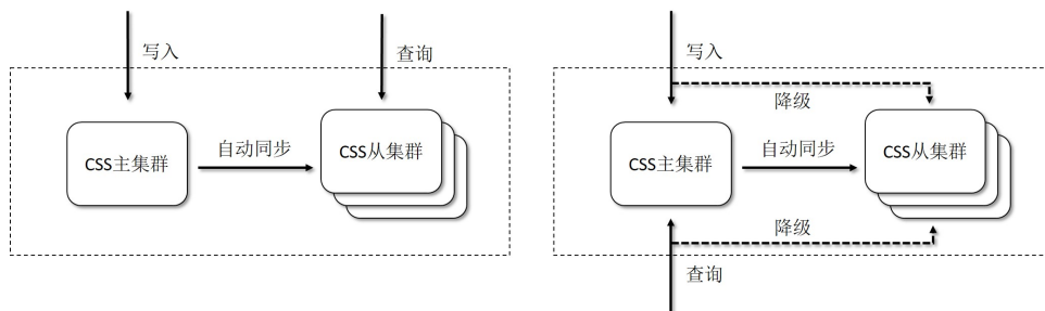
图 2-17 读写分离特性的两种使用场景
