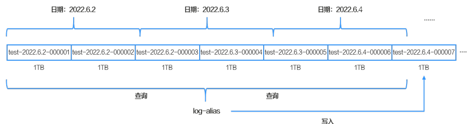
图 3-45 log-alias 的组织形态
