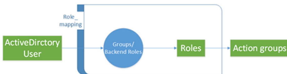
图 3-3 权限映射关系
