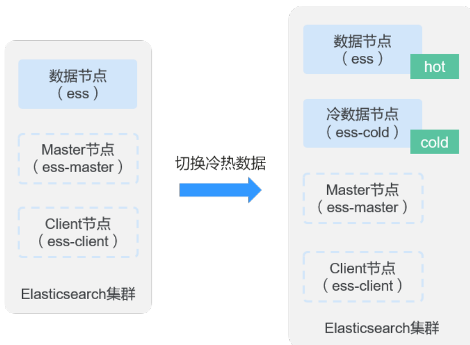
图 2-18 切换冷热数据原理
