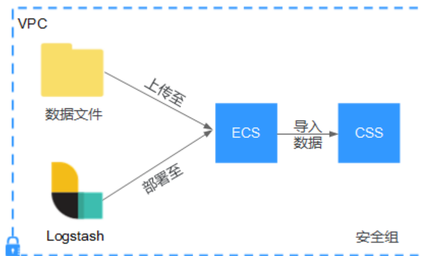
图 2-13 Logstash 部署在弹性云服务器上时导入数据示意图
