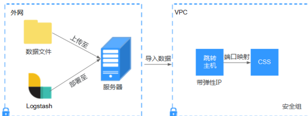
图 3-5 Logstash 部署在外网时导入数据示意图
