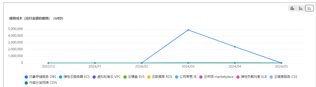
图 6-3 折线图
