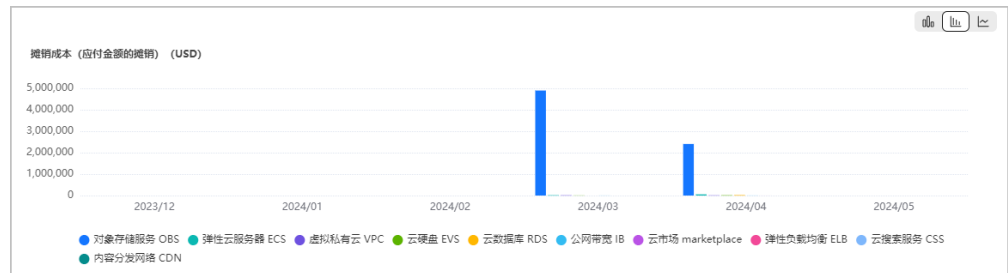
图 6-2 柱状图
