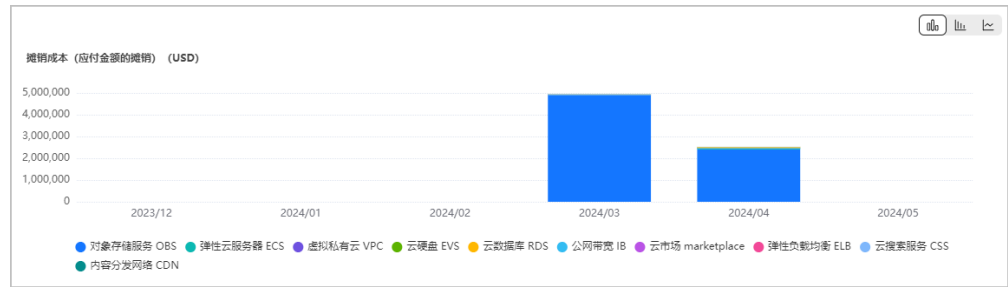
图 6-1 堆叠图
