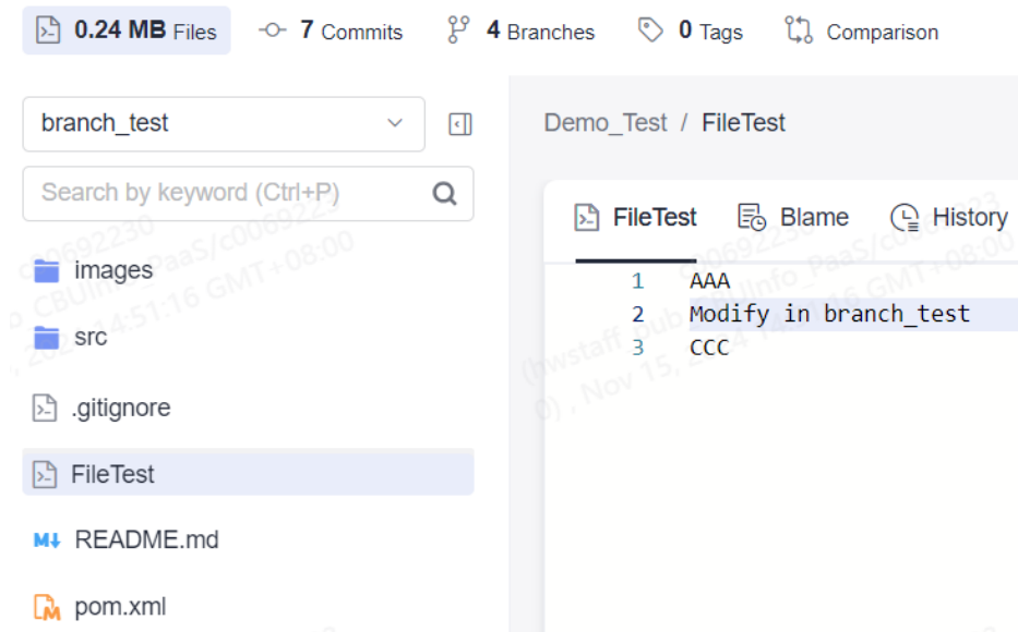
图 18-6 在 “branch_test” 分支修改 FileTest
