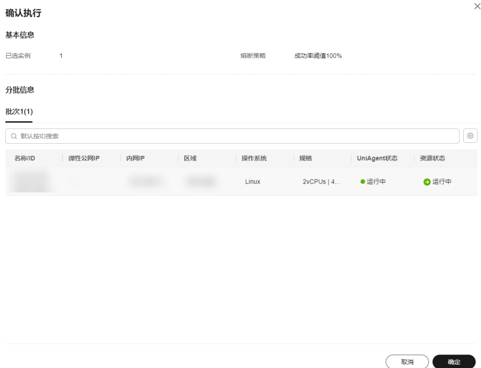
图 4-60 确认执行
