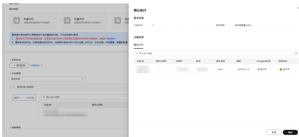
图 4-39 确定执行
