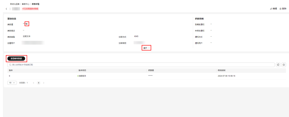
图 5-129 参数详情
