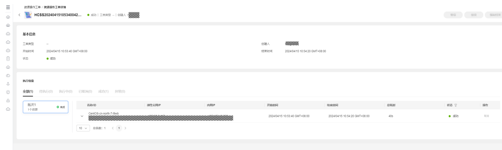
图 4-65 查看结果
