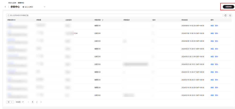
图 5-119 创建参数
