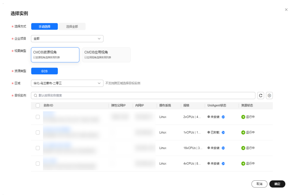
图 4-29 选择实例
