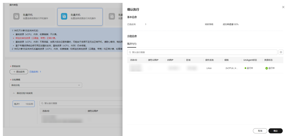
图 4-31 确认执行
