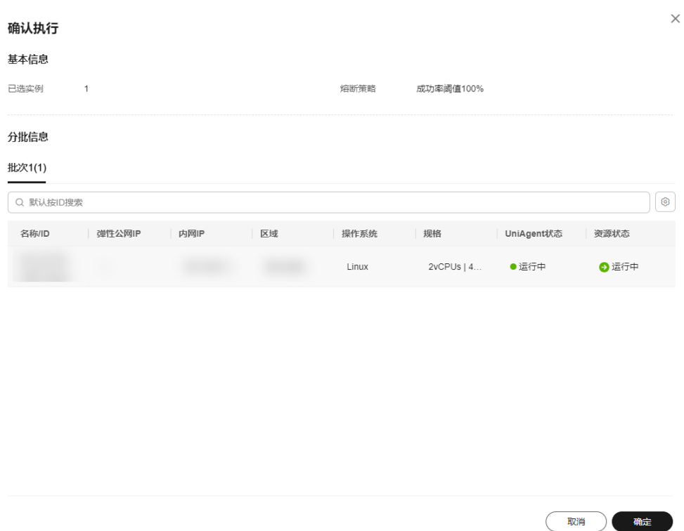
图 4-64 确认执行
