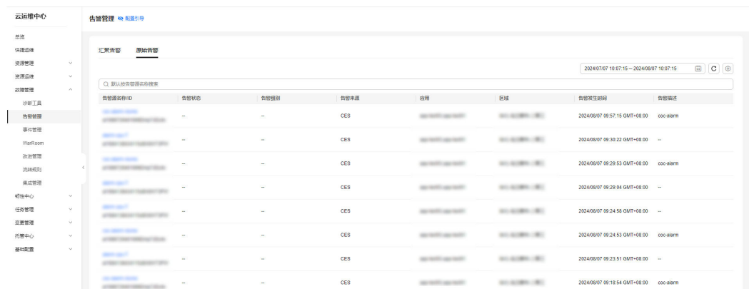
图 6-13 原始告警
