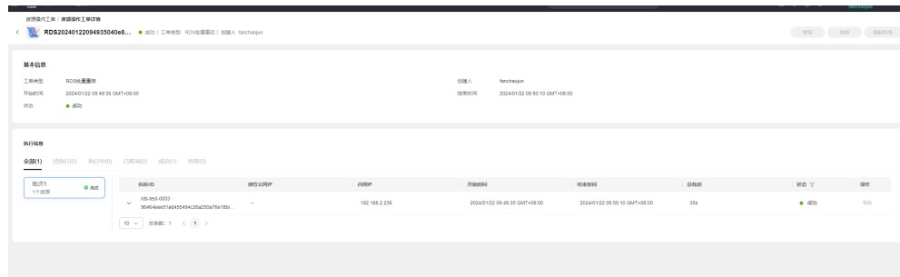
图 4-53 执行结果
