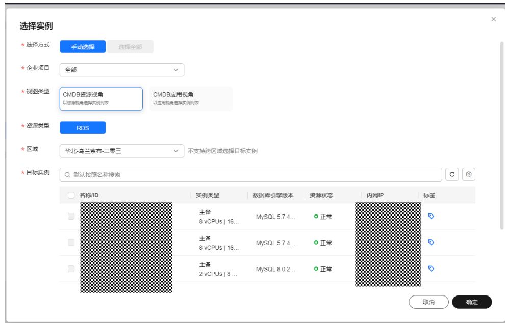
图 4-48 选择实例
