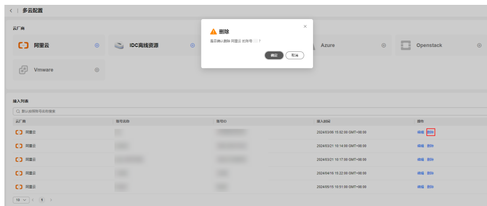
图 3-46 删除账号
