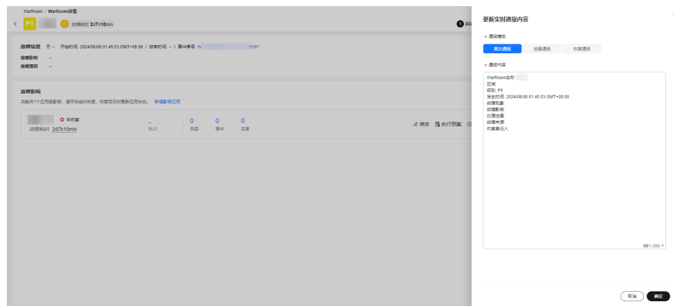
图 6-63 更新通告
