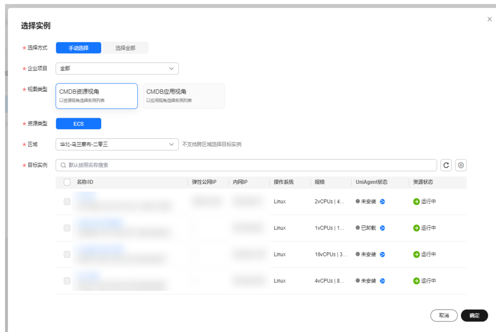
图 4-25 选择实例
