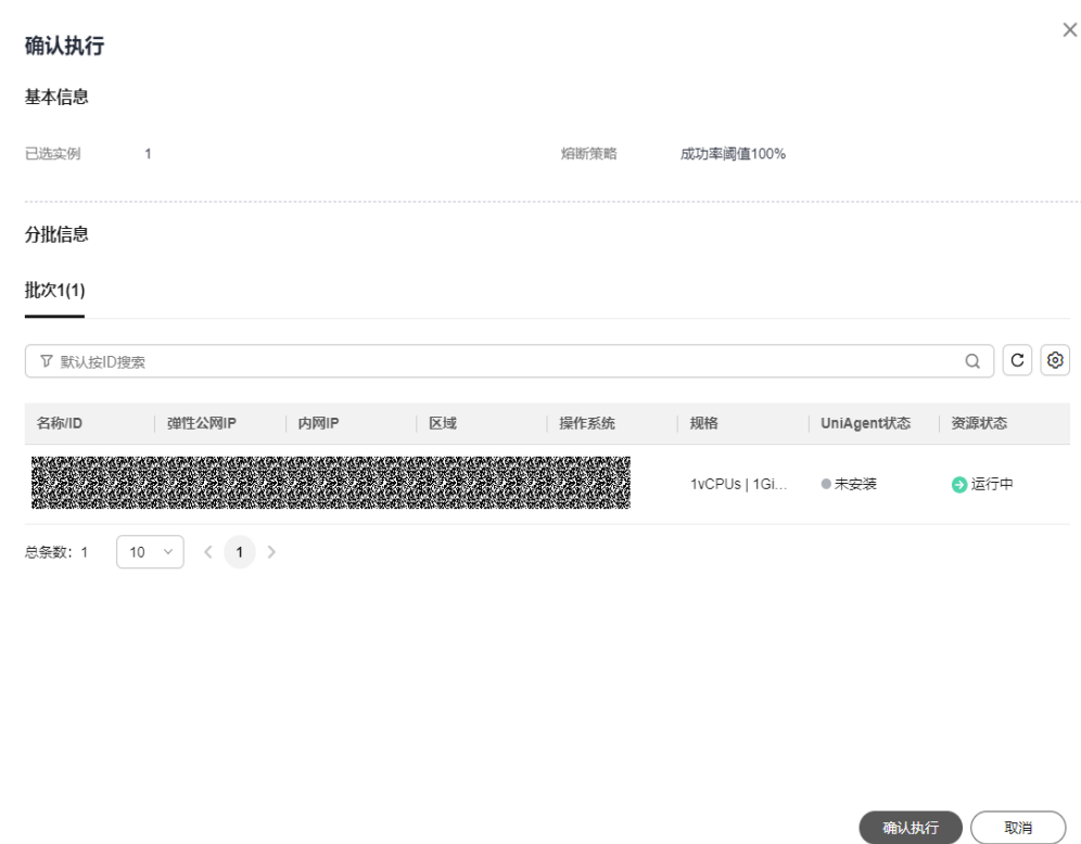
图 4-35 确认执行
