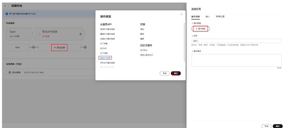
图 5-77 添加任务
