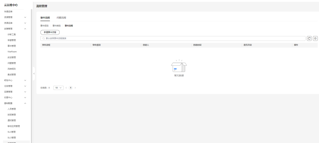
图 10-73 事件流程
