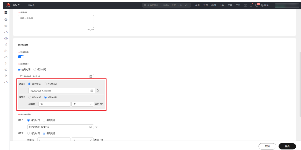
图 5-122 删除前通知
