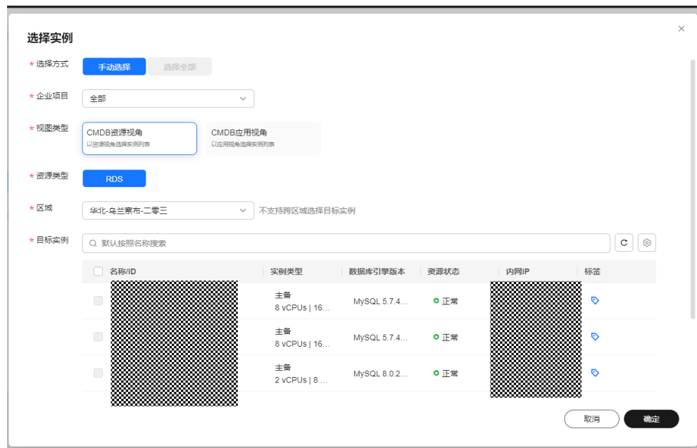
图 4-45 选择实例
