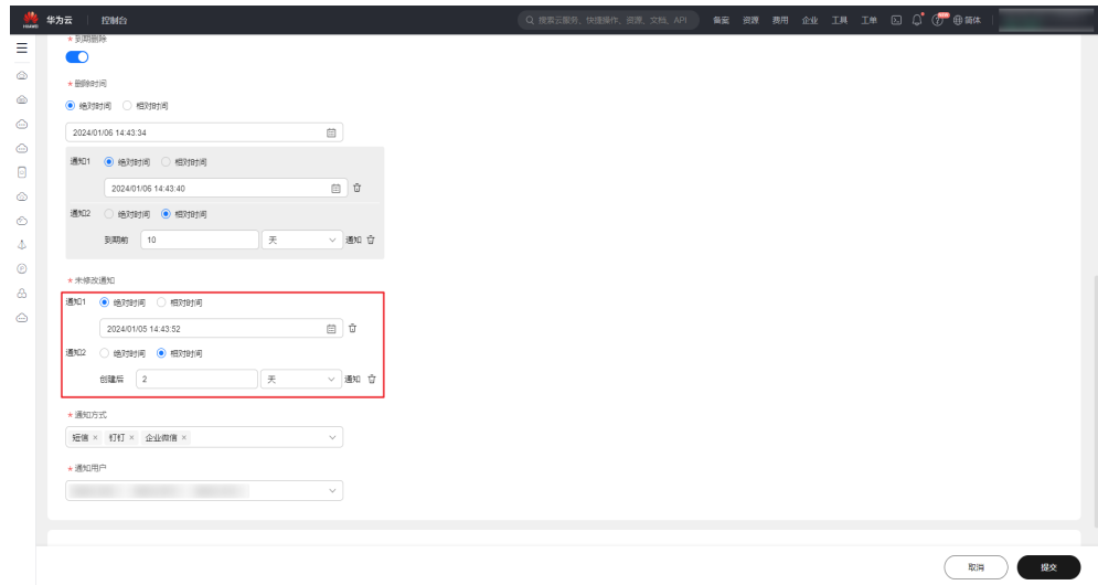
图 5-123 未修改通知
