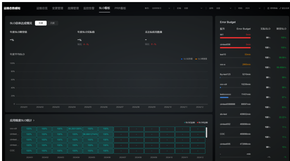
图 2-21 SLO 看板
