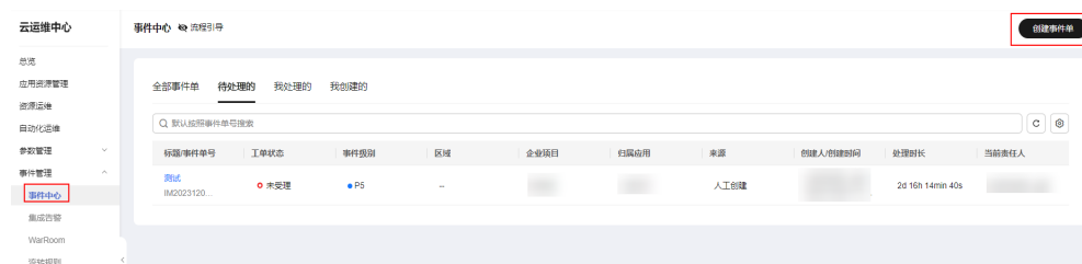
图 6-15 事件单列表
