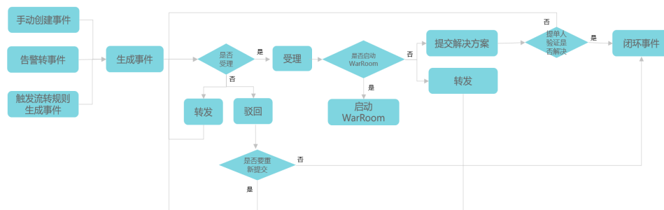
图 6-14 事件流程图
