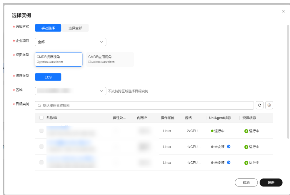
图 4-33 选择实例
