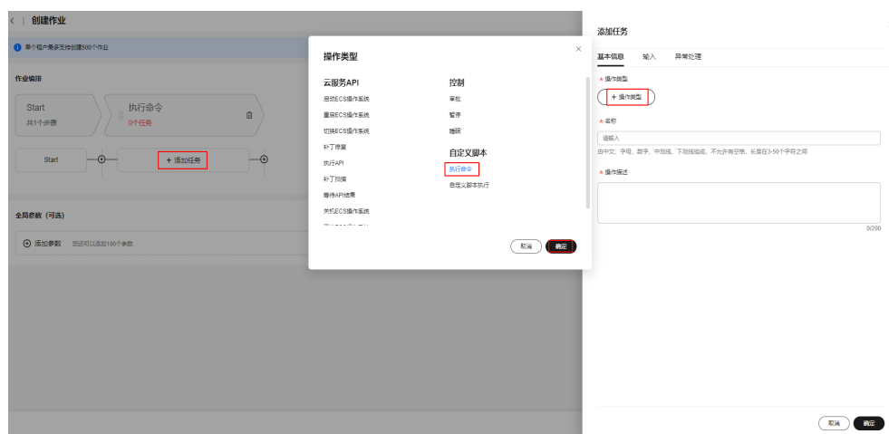
图 5-86 添加任务
