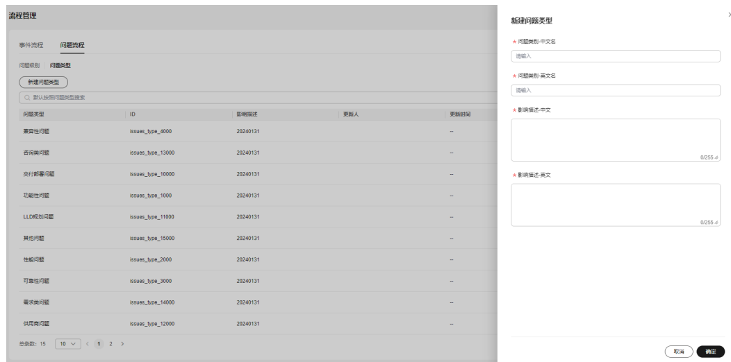
图 10-78 问题类型
