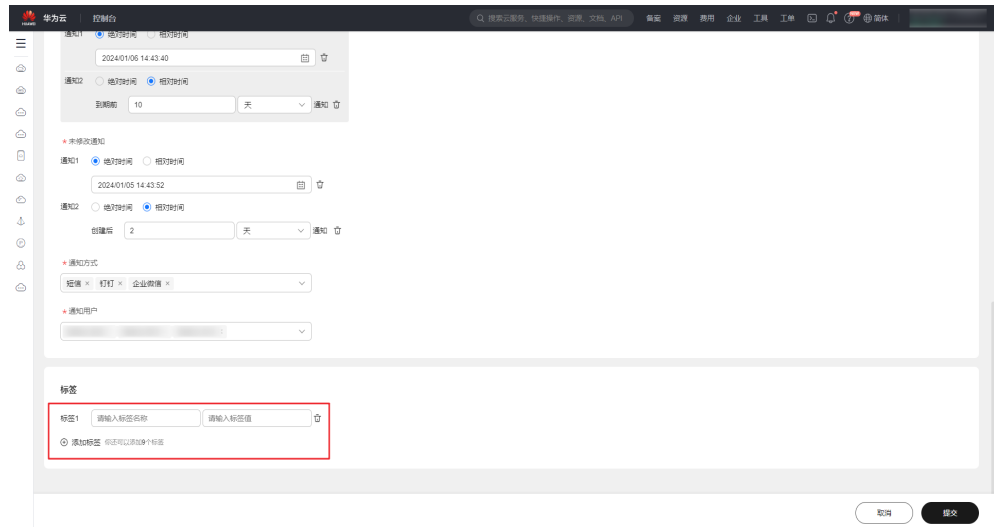
图 5-125 参数标签
