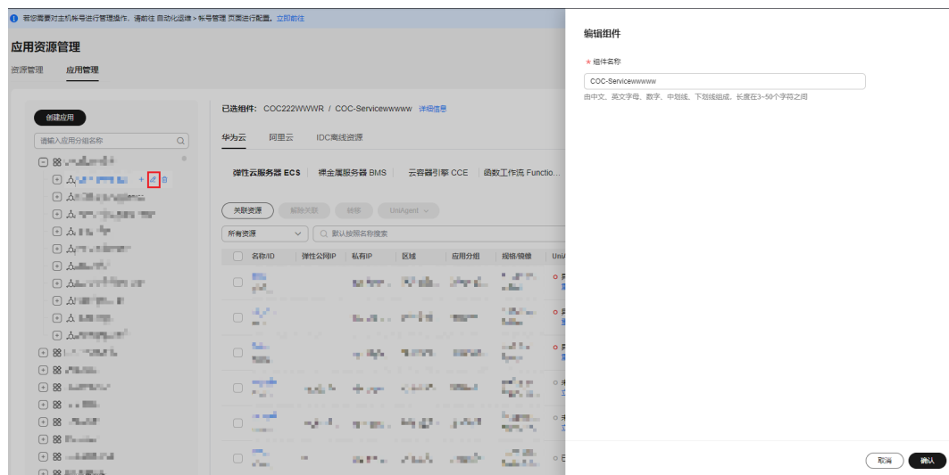
图 3-23 编辑组件
