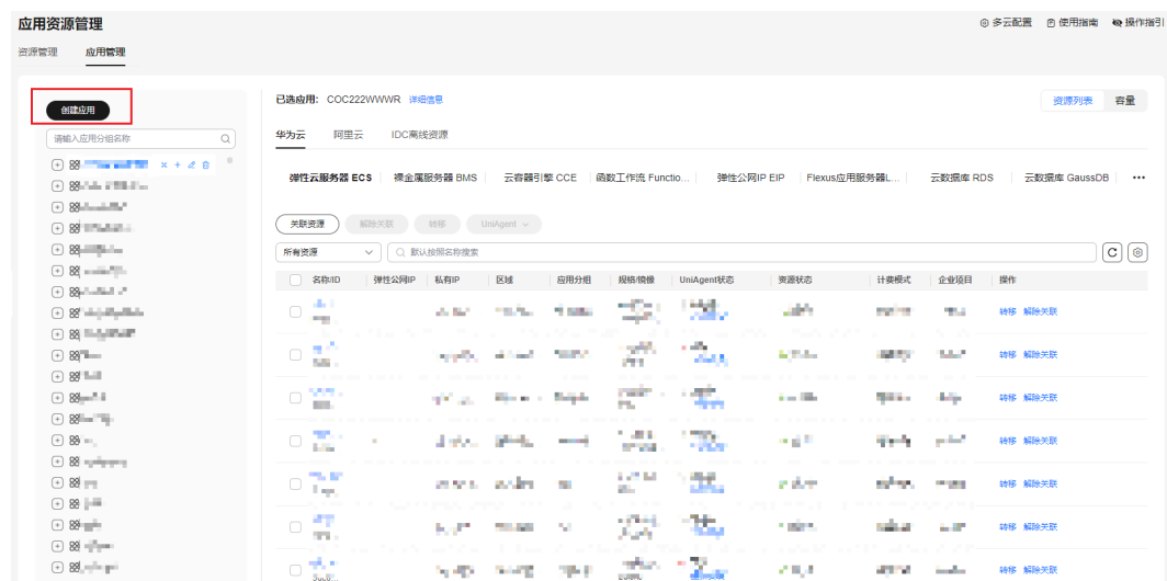
图 3-15 创建应用
