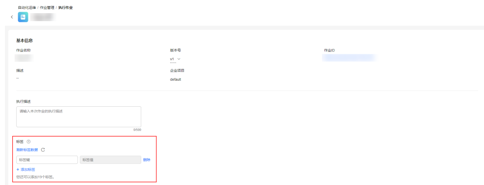
图 5-62 创建标签
