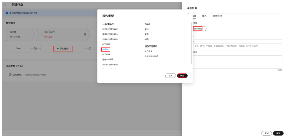
图 5-68 添加任务
