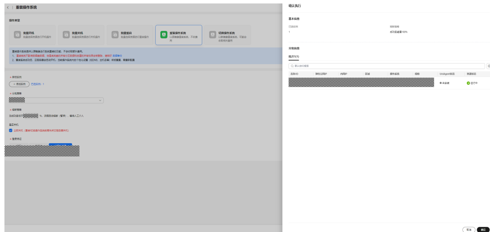
图 4-68 确定执行
