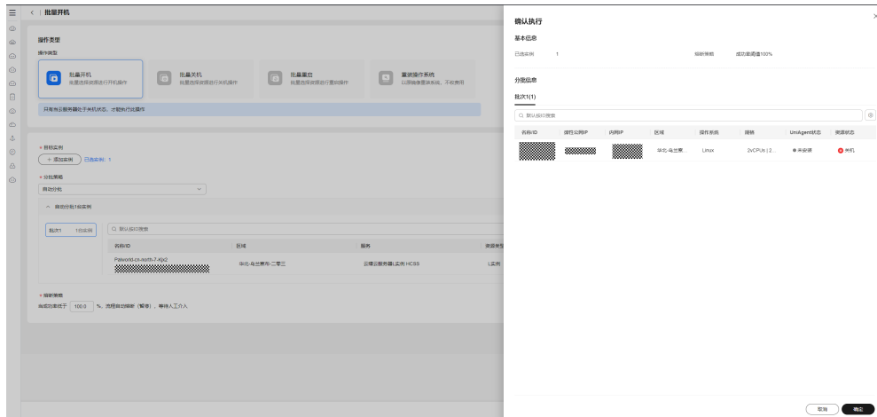
图 4-56 确认执行
