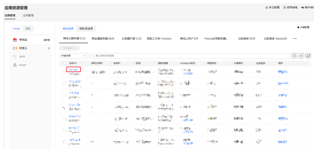
图 3-11 查看详情
