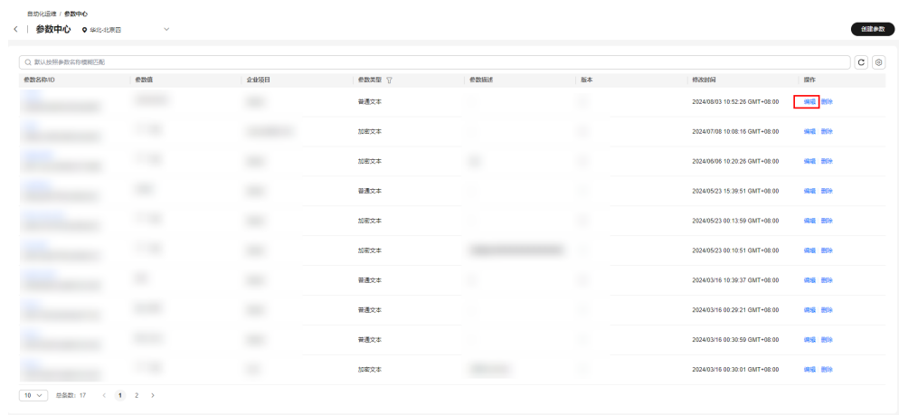
图 5-126 参数列表
