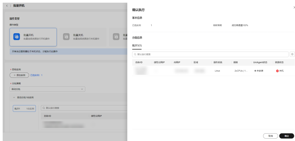
图 4-27 确认执行
