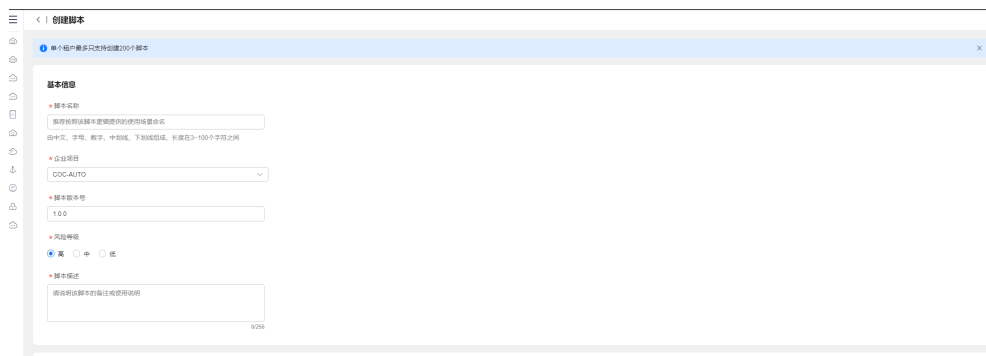
图 5-2 填写信息
