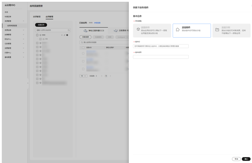
图 3-18 创建组件
