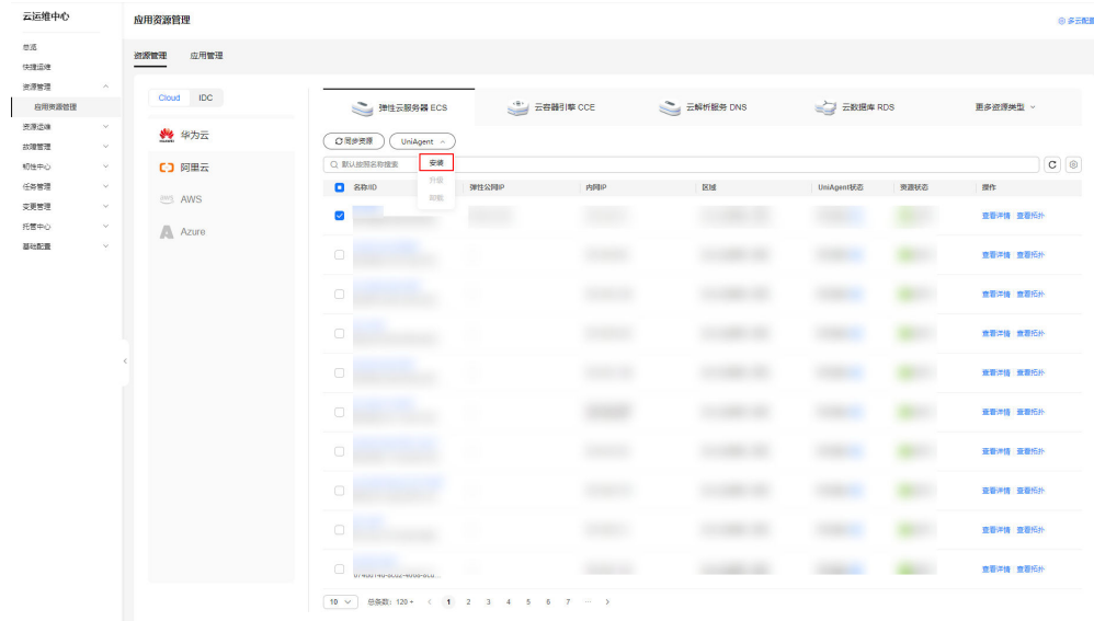
图 3-4 安装 UniAgent
