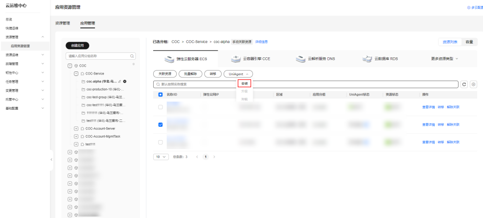
图 3-29 安装 UniAgent
