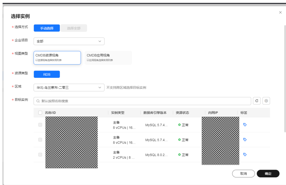
图 4-45 选择实例
