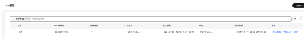
图 11-60 筛选 SLO
