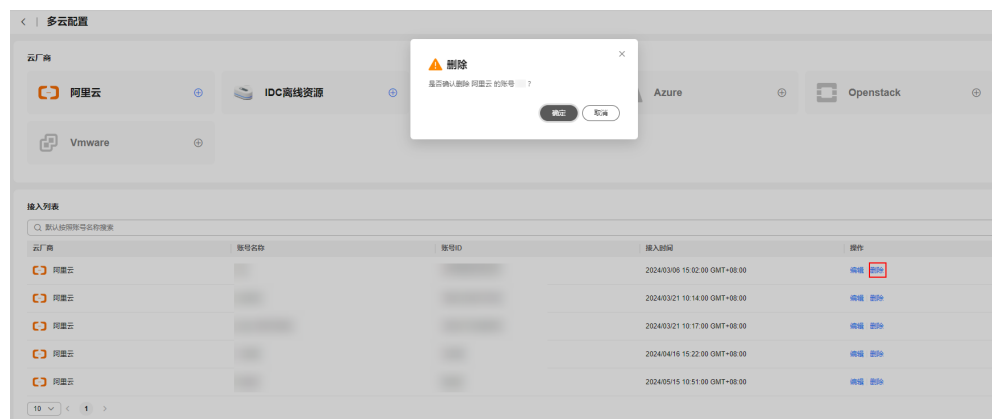
图 3-41 删除账号
