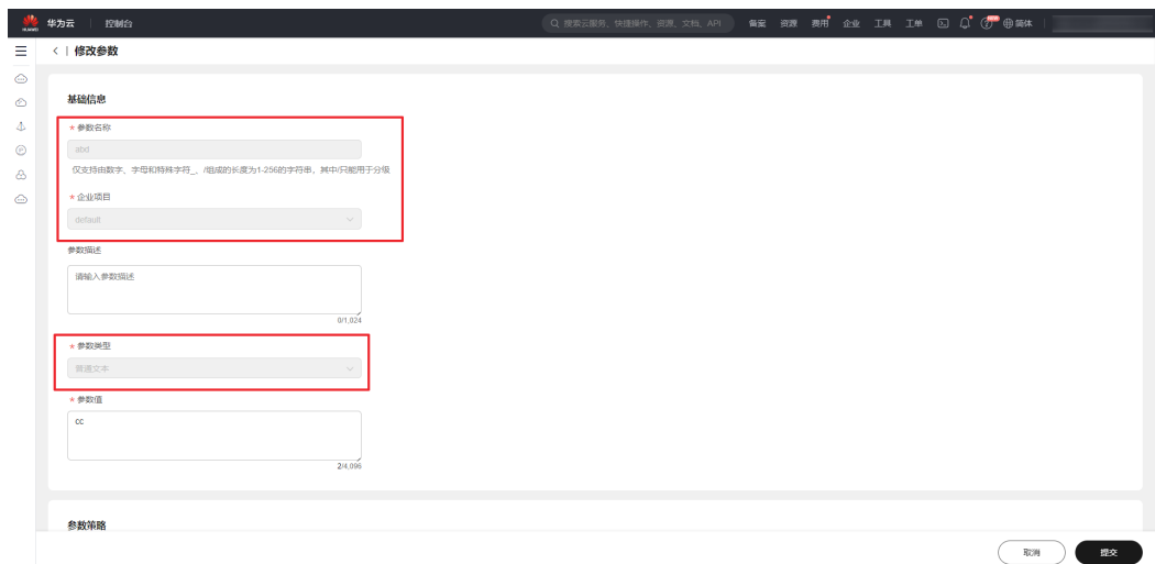
图 6-9 参数详情
