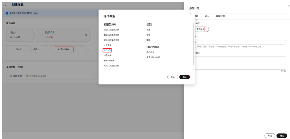
图 5-65 添加任务
