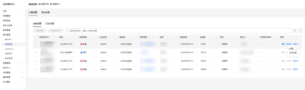
图 7-2 处理告警单
