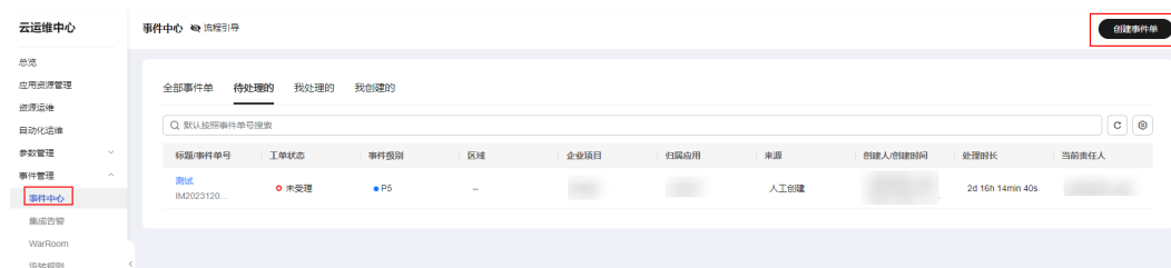
图 7-9 事件单列表
