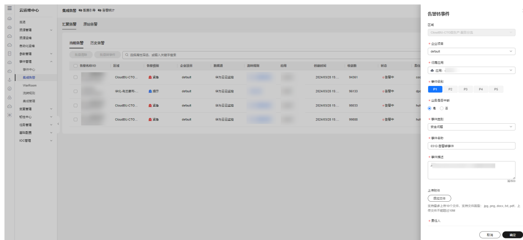
图 7-4 告警转事件
