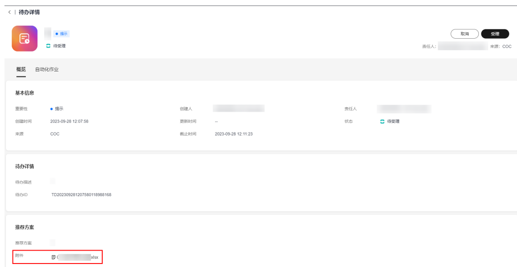
图 10-22 下载附件
