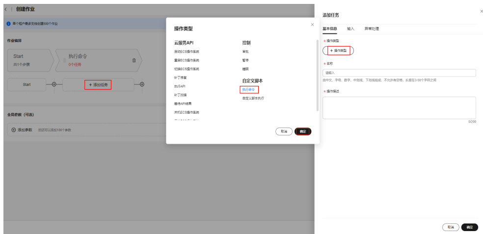
图 5-83 添加任务
