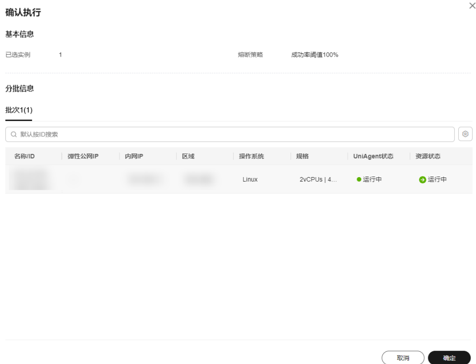
图 4-43 确定执行
