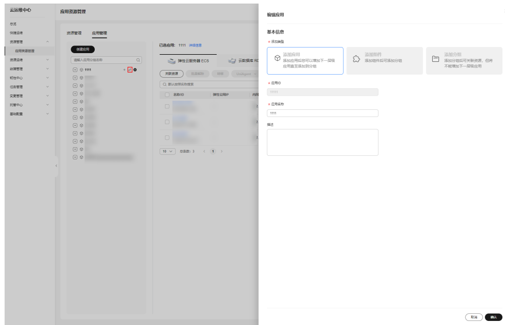
图 3-16 编辑应用
