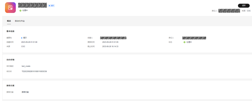
图 10-25 闭环待办
