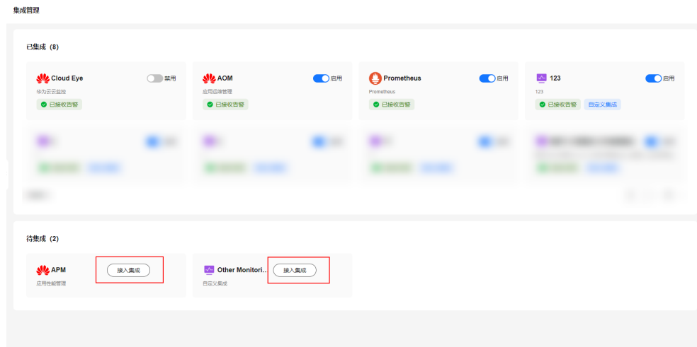
图 7-63 接入集成
