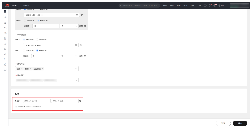
图 6-7 参数标签
