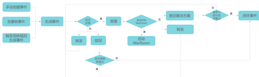
图 7-8 事件流程图
