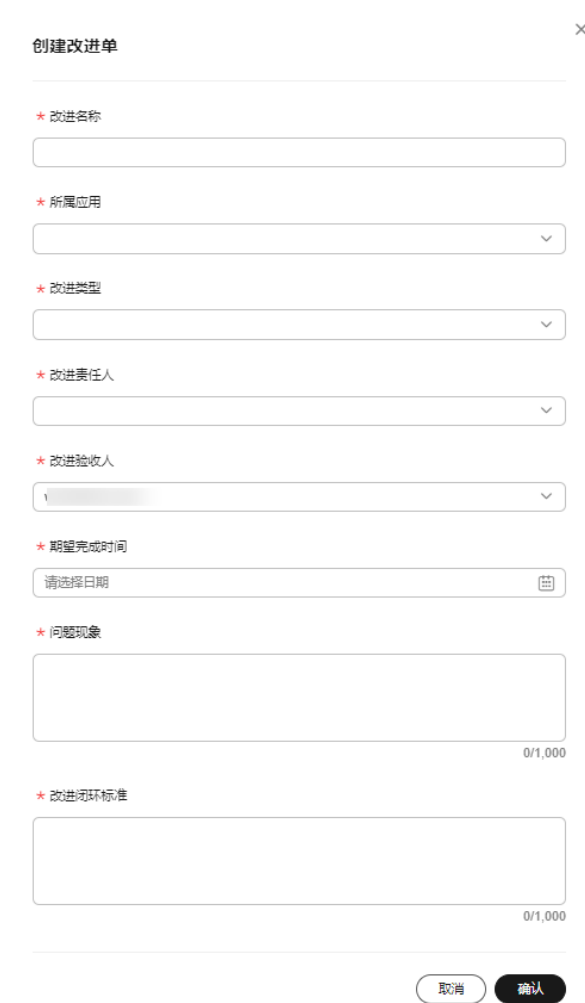
图 7-41 创建改进单
