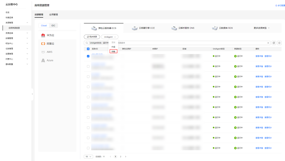
图 3-9 卸载 UniAgent
