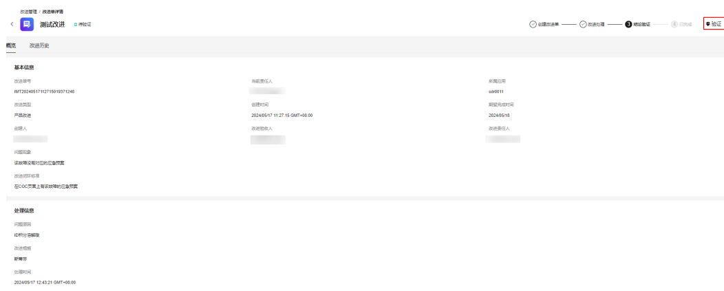
图 7-56 改进单验证
