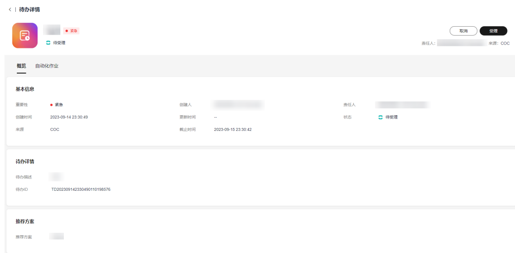
图 10-21 待办详情
