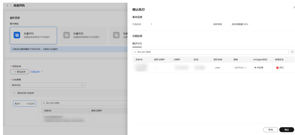
图 4-27 确认执行
