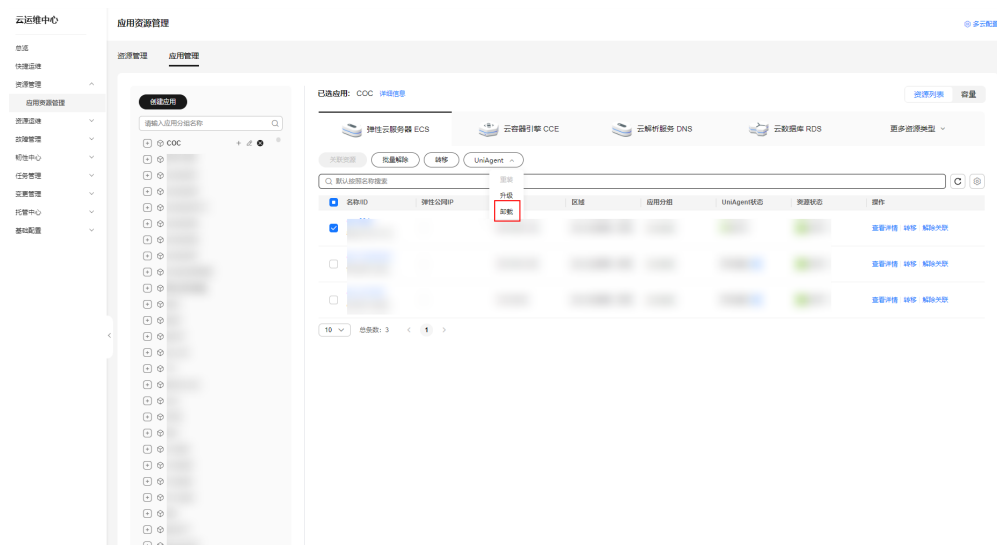
图 3-34 卸载 UniAgent
