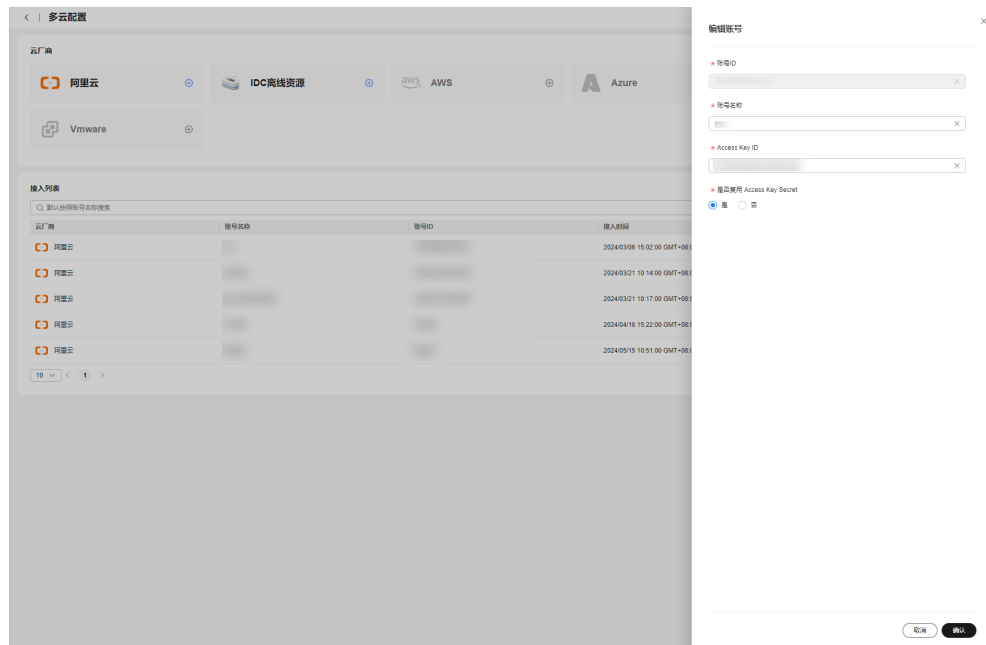
图 3-40 编辑账号
