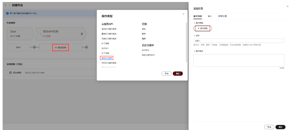
图 5-74 添加任务
