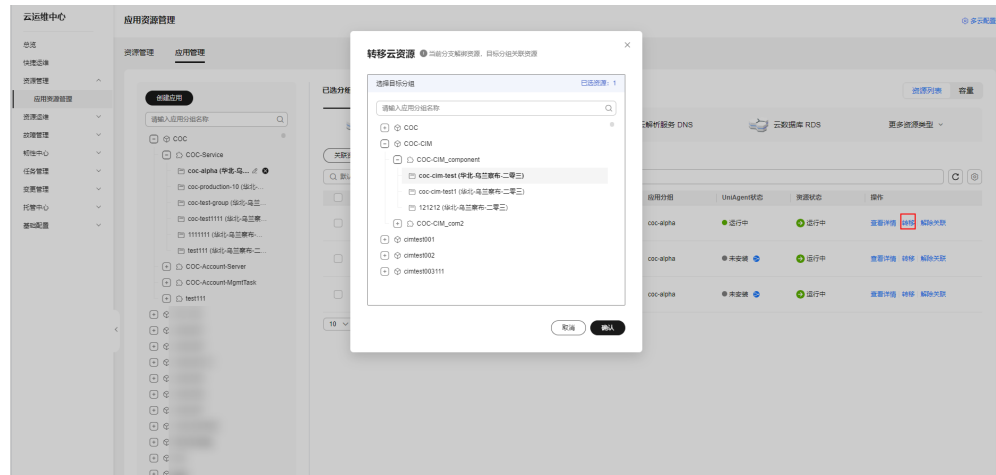
图 3-27 转移资源
