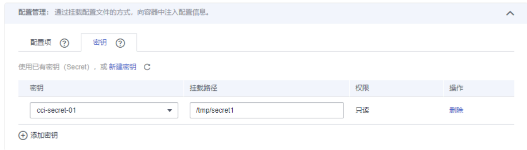
图 7-3 将 Secret 挂载到容器中
