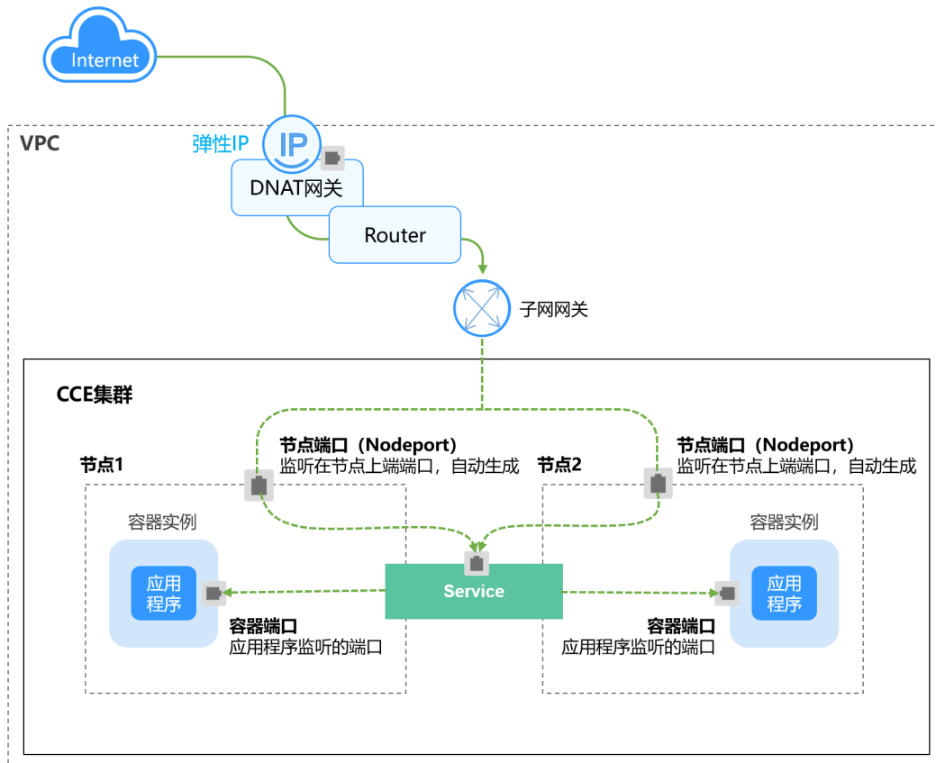
图 3-155 DNAT 网关 ( DNAT )
