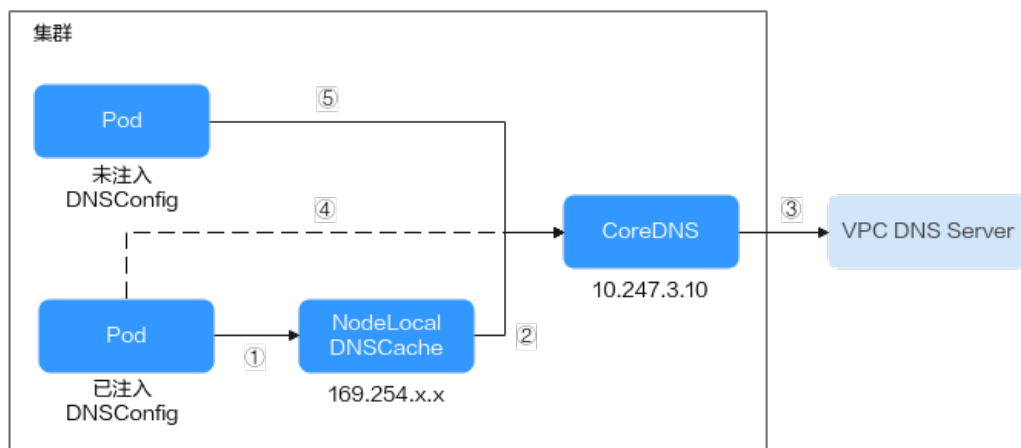
图 3-298 NodeLocal DNSCache 查询路径
