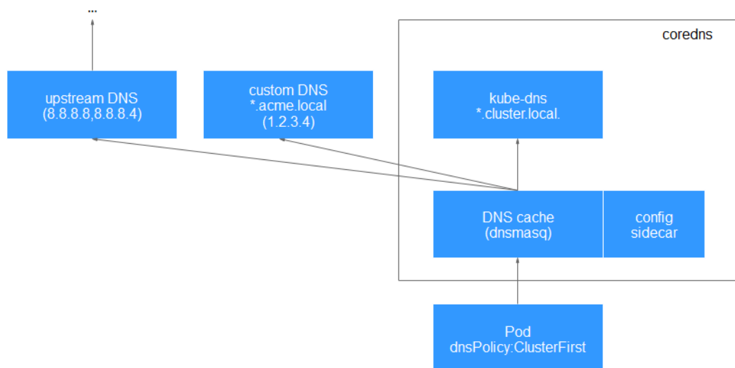
图 3-166 路由请求流程
