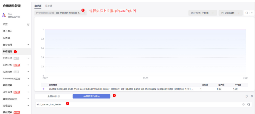
图 3-258 查看指标
