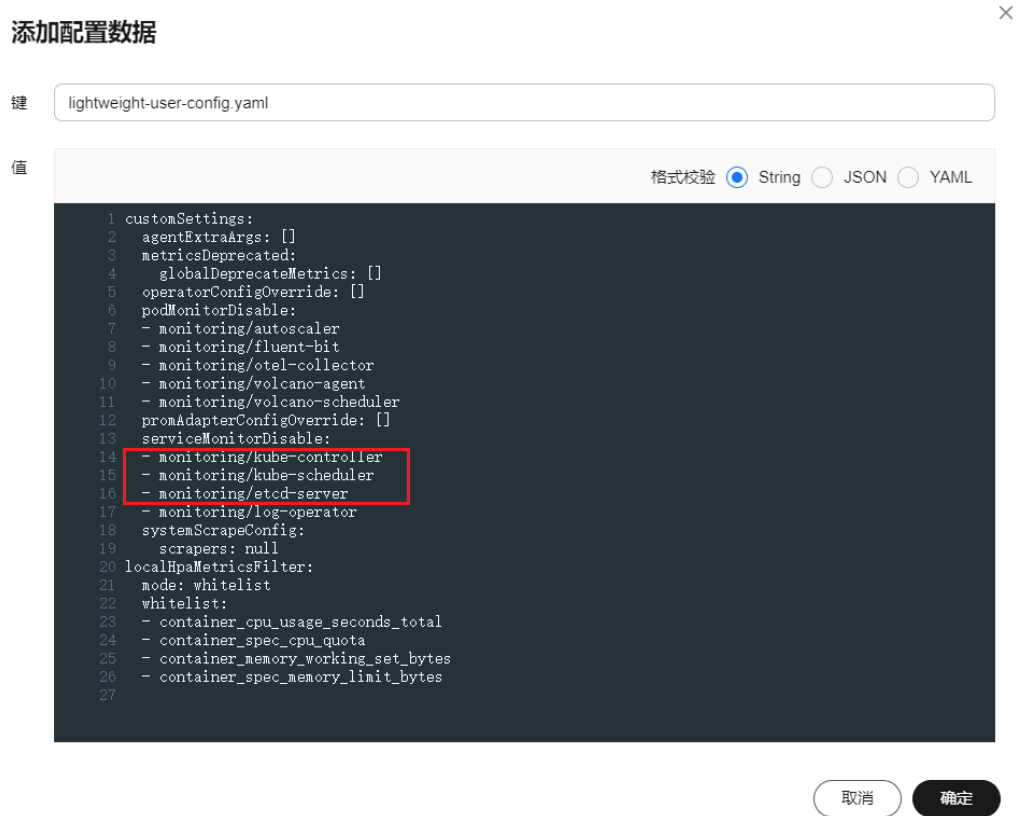
图 3-257 删除配置
