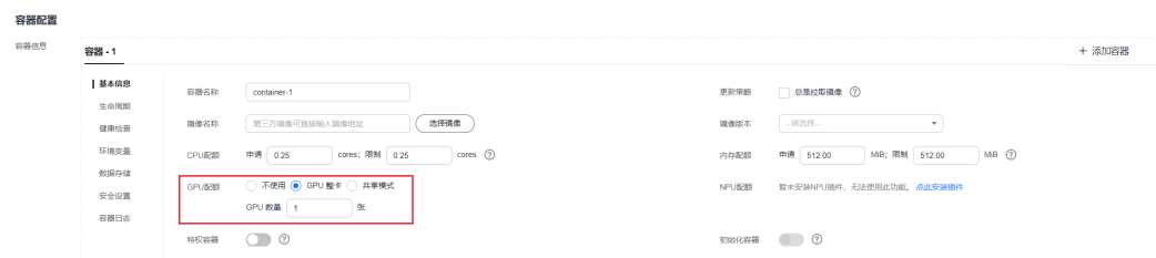
图 3-92 使用 GPU
