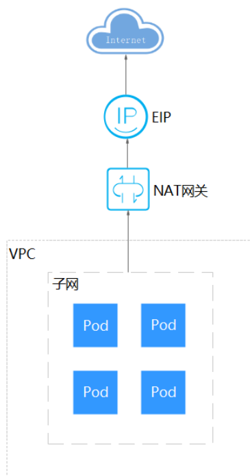
图 3-182 SNAT
