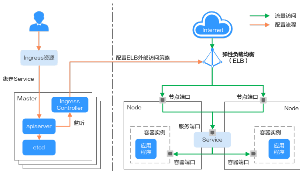
图 3-157 ELB Ingress 工作原理（CCE Standard 集群以及 CCE Turbo 集群使用共享型 ELB 场景）
