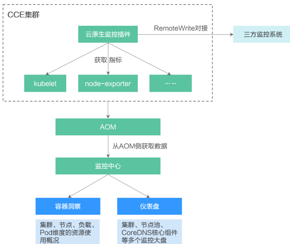
图 3-193 监控中心架构
