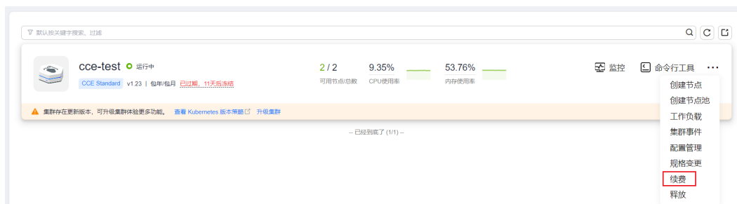
图 3-42 续费集群
