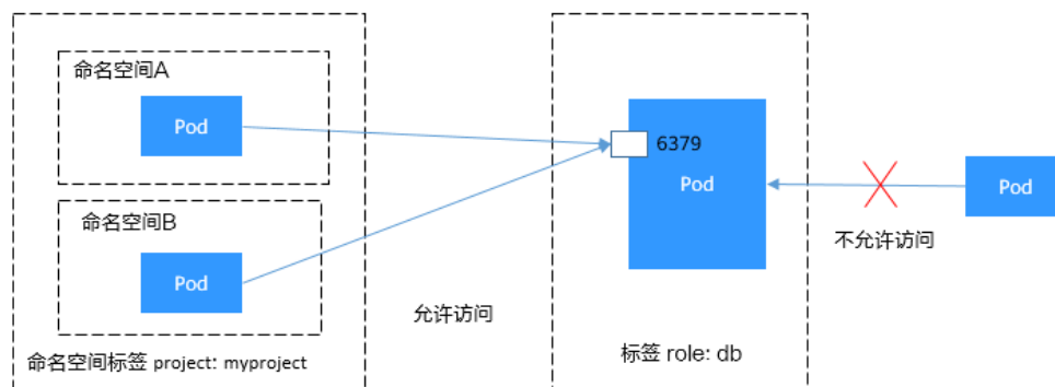
图 3-170 namespaceSelector
