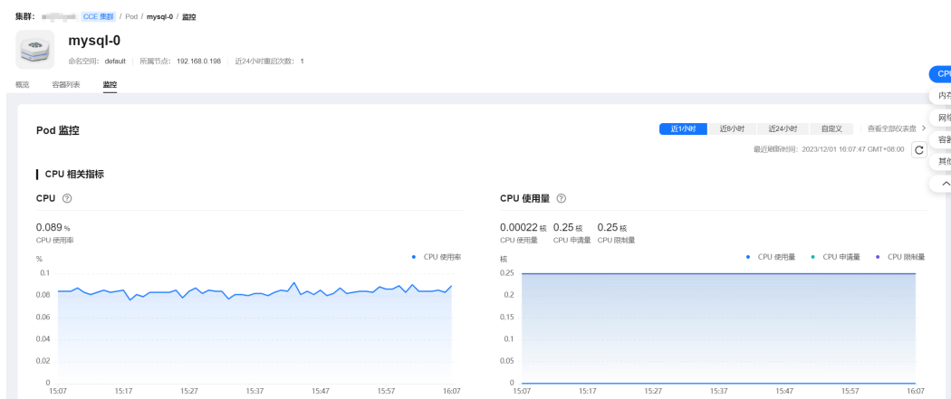
图 3-213 Pod 监控
