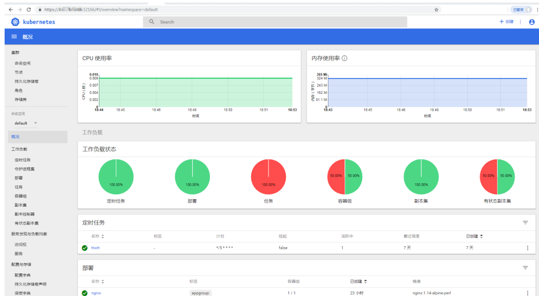
图 3-286 Dashboard 概览页
