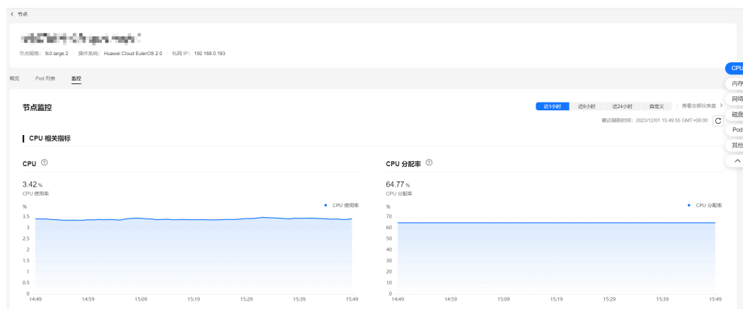
图 3-204 节点监控
