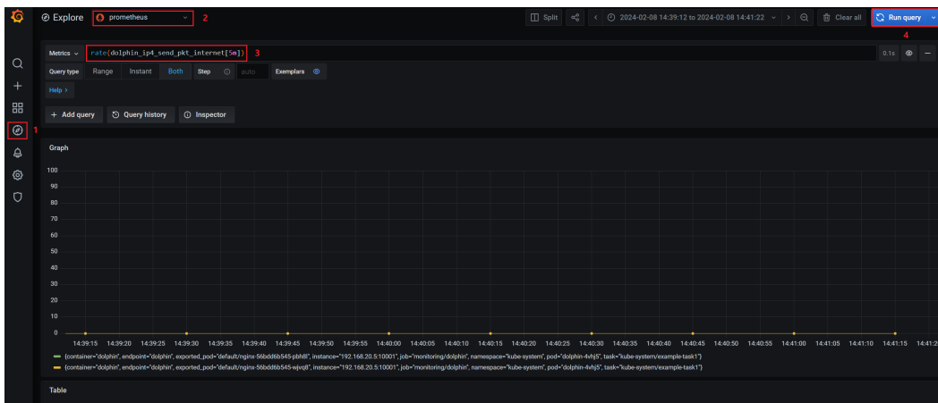
图 3-263 Grafana 图表
