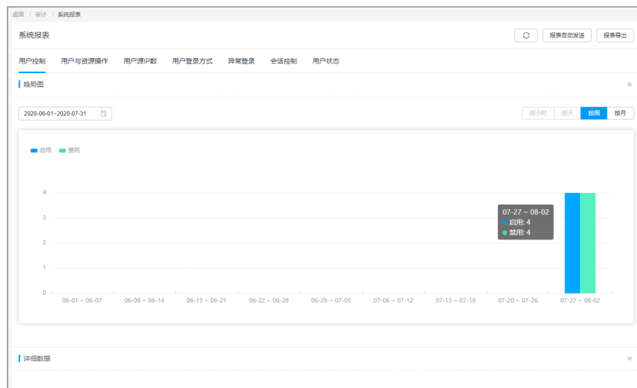
图 10-31 系统报表
