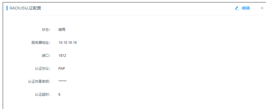
图 5-46 RADIUS 域认证
