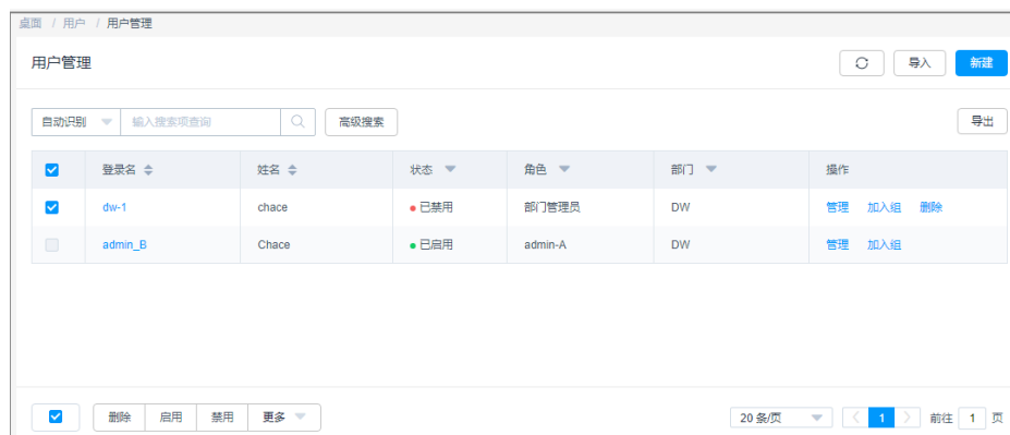
图 5-7 删除用户
