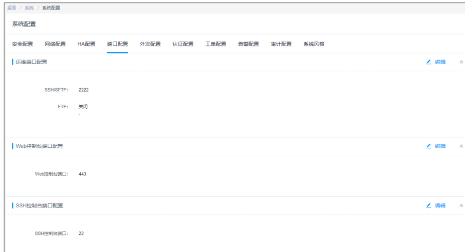
图 11-11 端口配置
