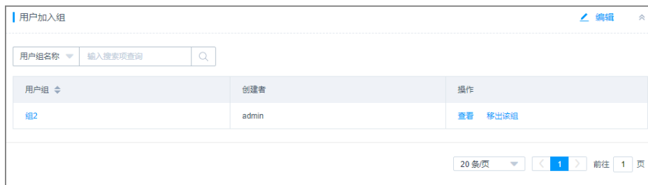
图 5-18 用户加入组
