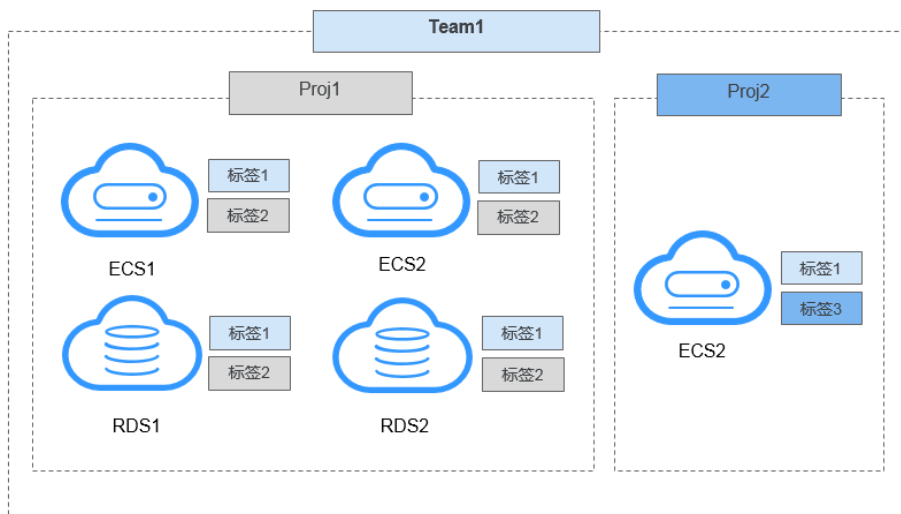
图 6-58 标签示例
