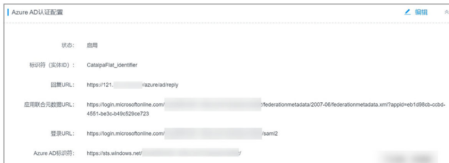
图 5-49 Azure AD 认证
