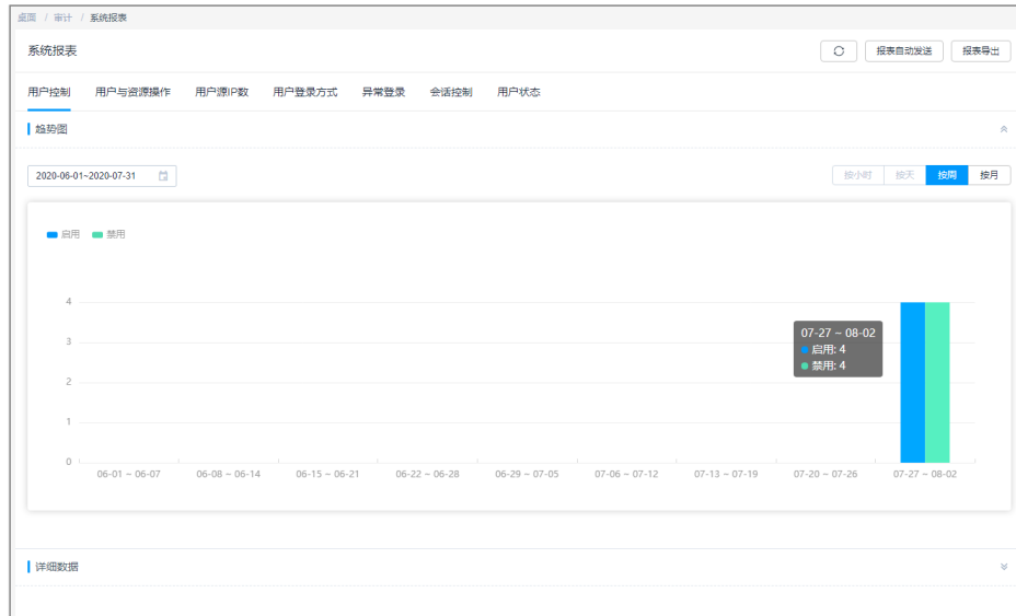
图 10-39 系统报表
