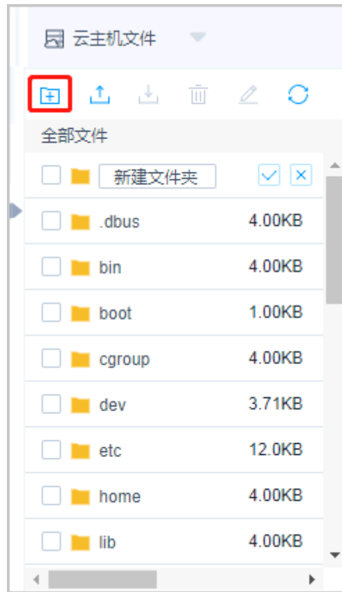
图 9-48 新建文件夹
