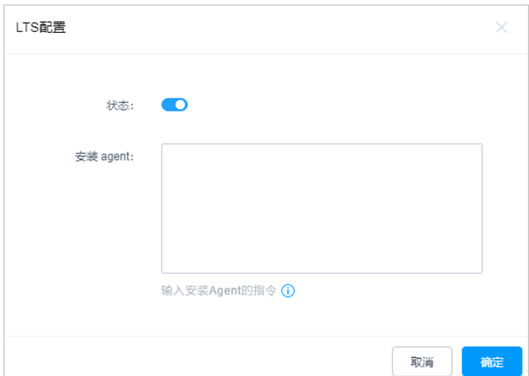
图 11-26 LTS 配置
