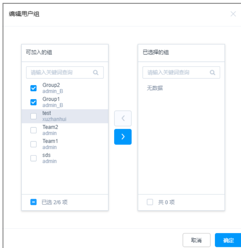
图 5-26 用户加入组
