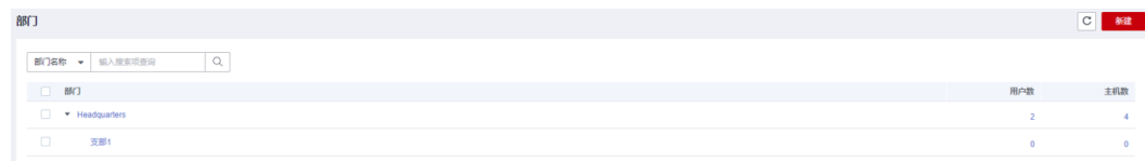
图 4-1 部门管理
