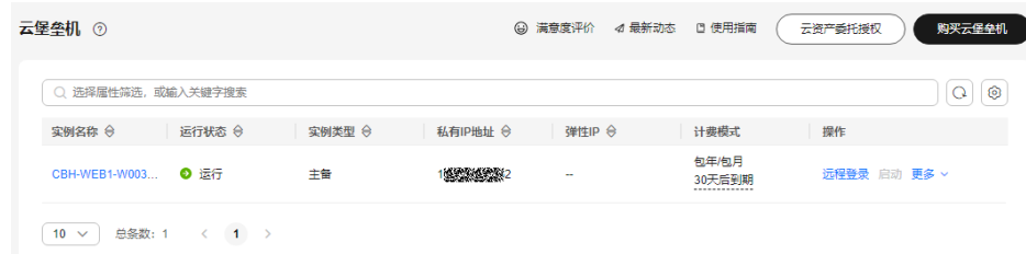
图 1-19 实例列表
