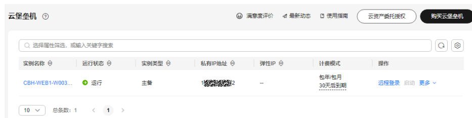
图 1-10 实例列表
