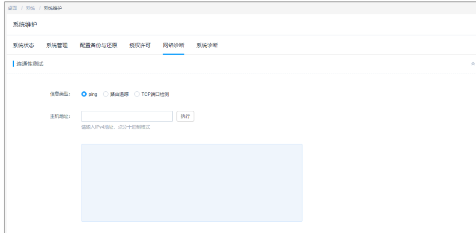
图 11-64 网络诊断
