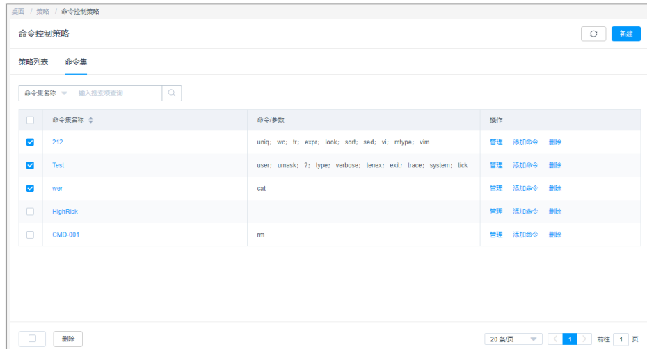
图 7-32 命令集列表
