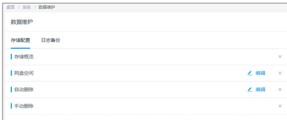
图 11-36 存储配置
