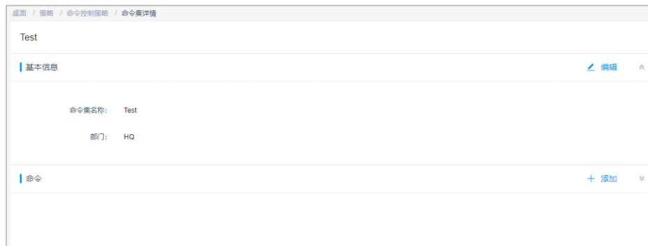
图 7-33 命令集详情
