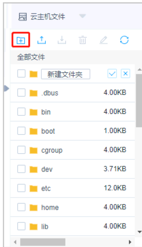
图 9-8 新建文件夹
