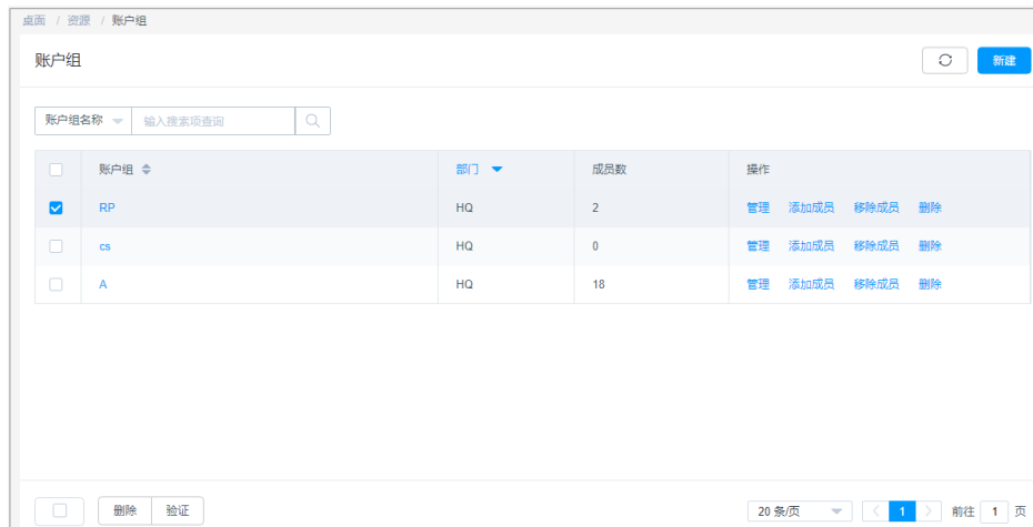
图 6-56 删除账户组
