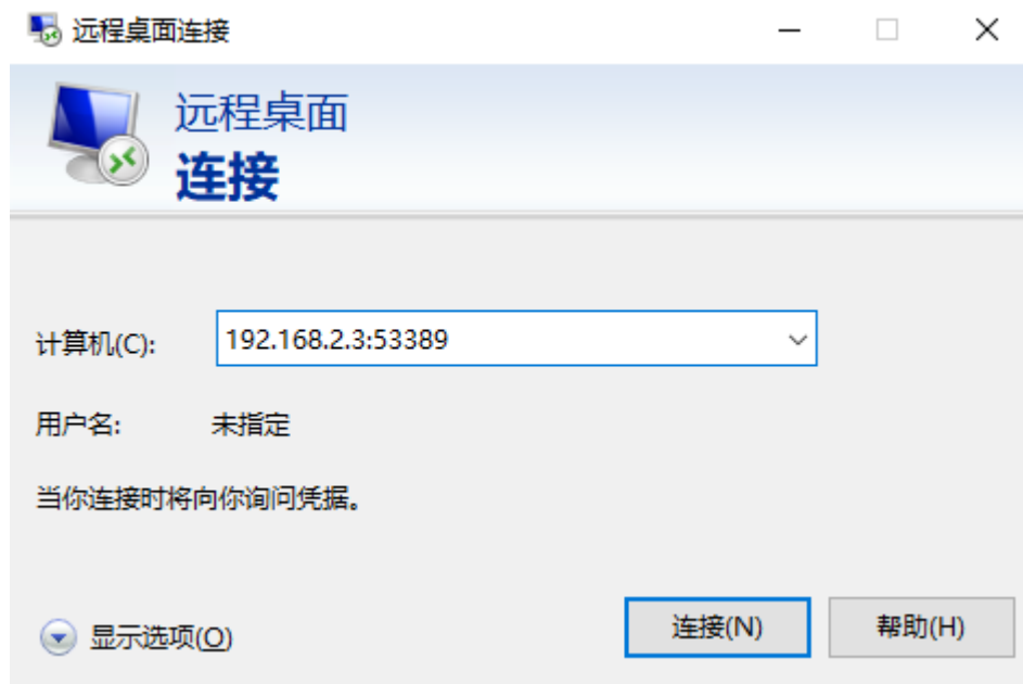
图 2-7 配置计算机
