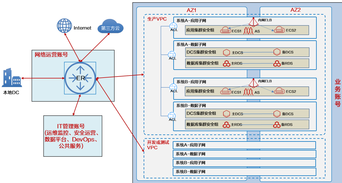
图 3-19 业务账号内的网络规划：多个业务系统共用一个子账号
