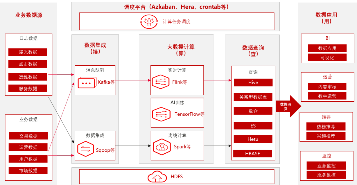
图 5-20 大数据参考架构
