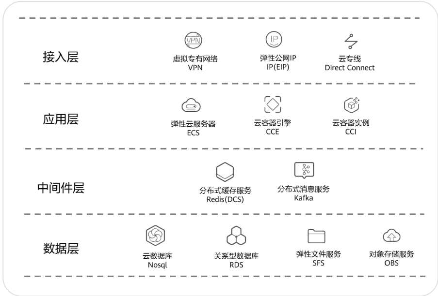
图 5-2 应用的四层部署架构设计
