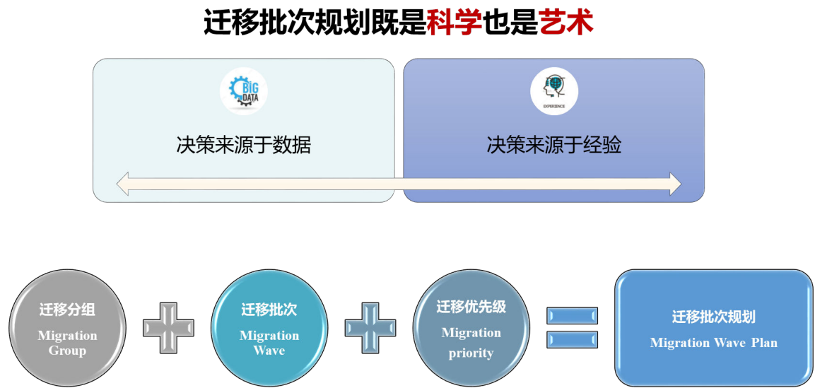
图 5-25 批次规划
