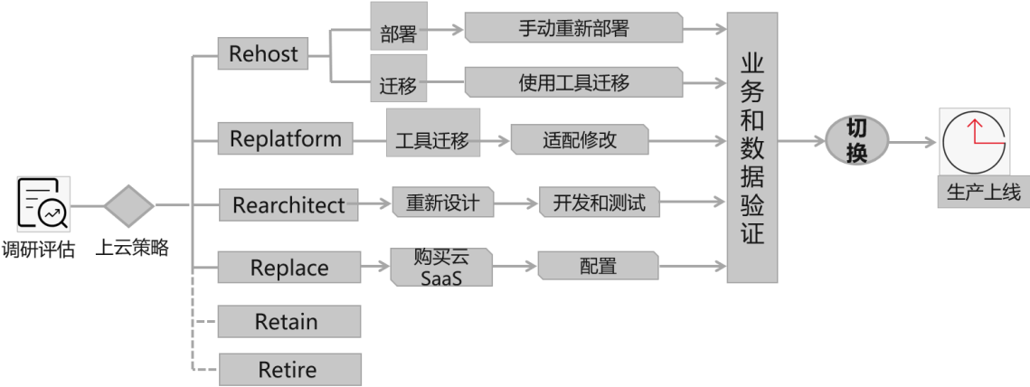
图 5-21 6R 策略
