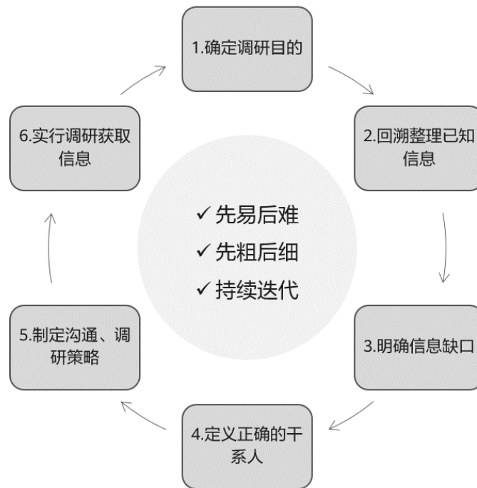
图 4-1 调研方法
