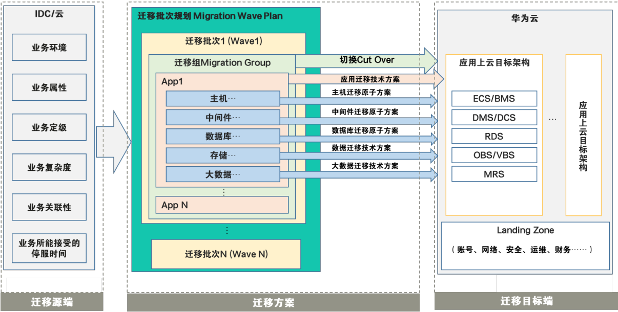
图 5-24 迁移概览图
