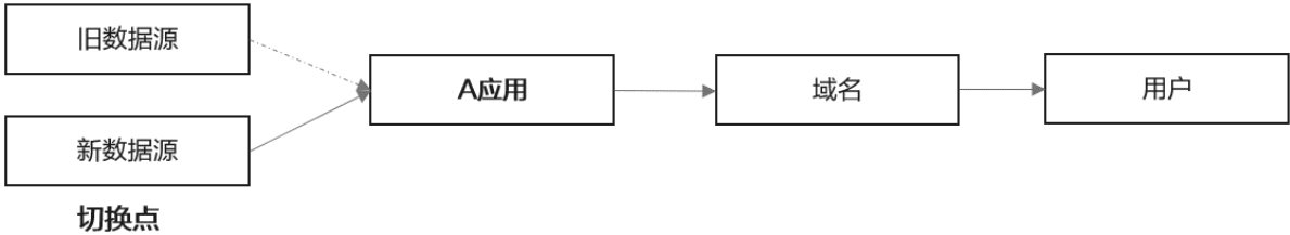
图 6-49 推数场景
