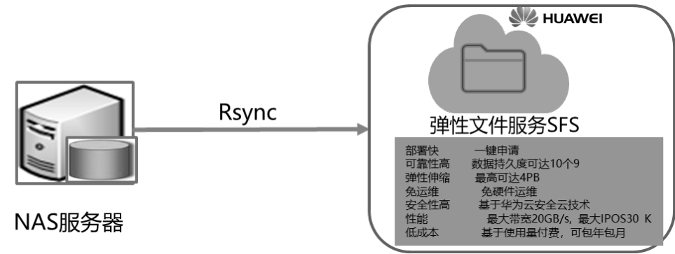
图 6-30 Rsync 迁移
