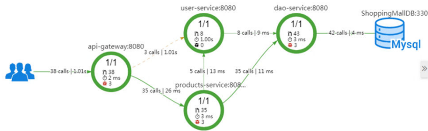
图 4-8 CMDB 法
