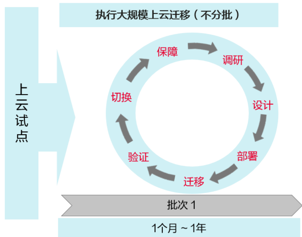
图 6-2 整体迁移
