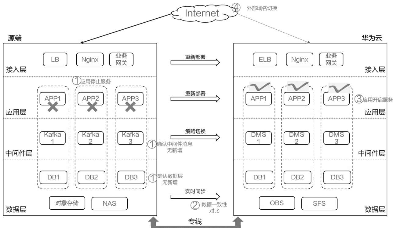
图 6-10 一把切方案
