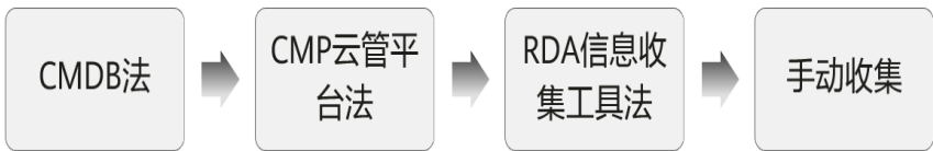
图 4-4 调研方式图
