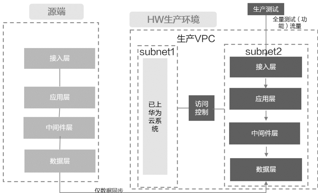
图 6-37 演练环境
