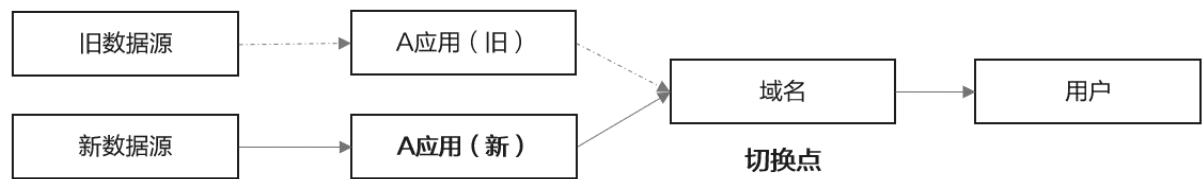
图 6-48 双跑场景
