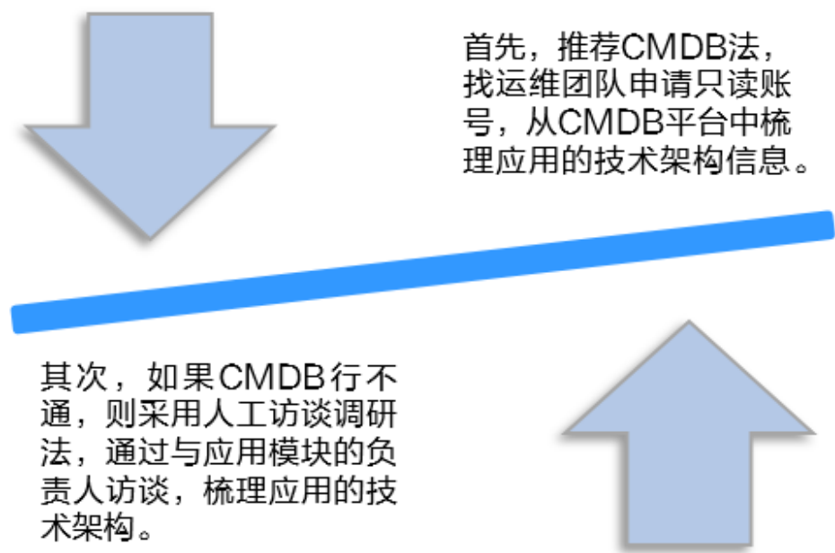
图 4-3 调研方式
