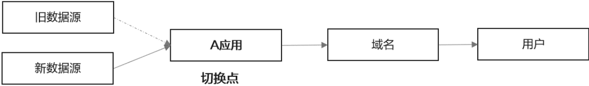
图 6-50 抽数场景
