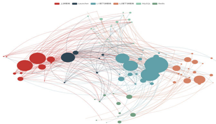
图 4-9 CMDB 法示例
