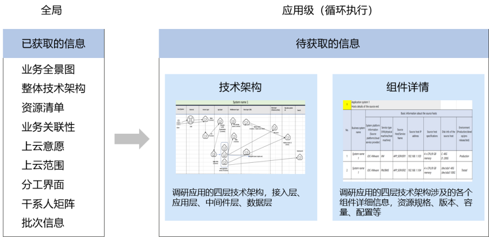
图 6-6 应用调研
