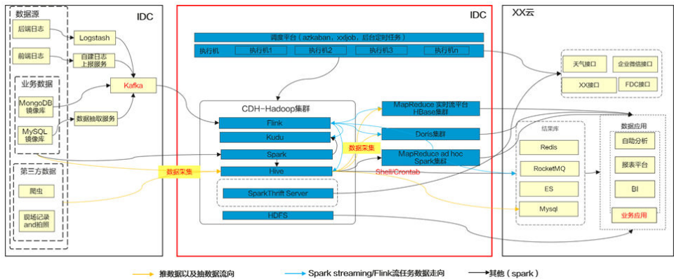
图 4-12 数据流示例
