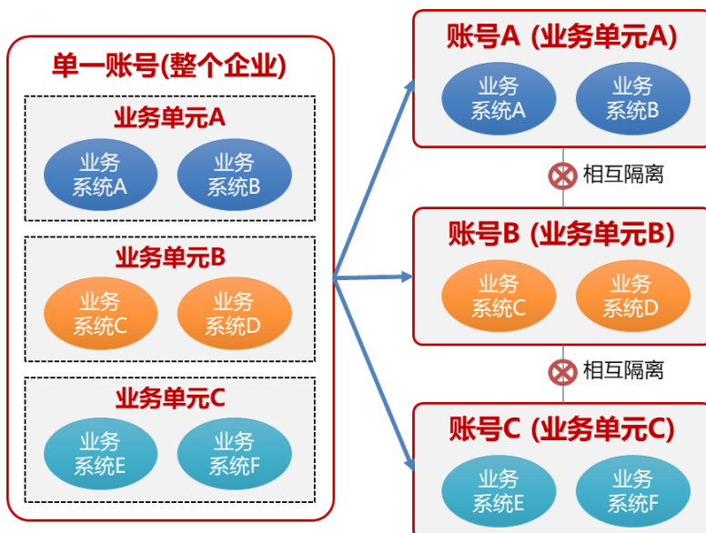
图 3-5 多账号部署
