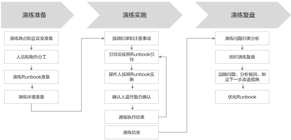
图 6-35 演练流程
