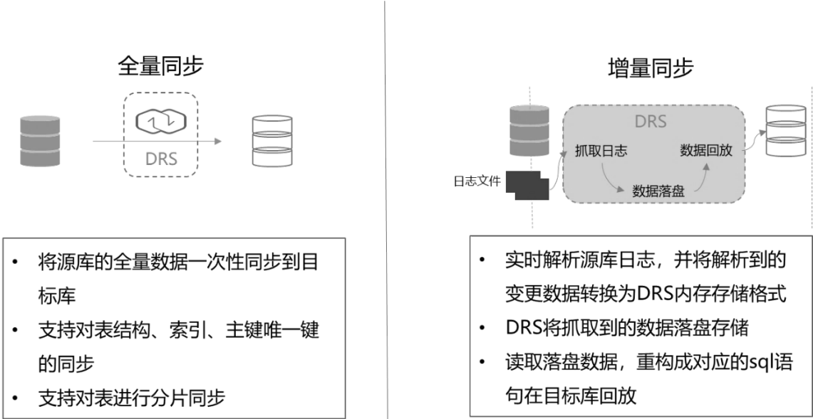
图 6-31 DRS 迁移
