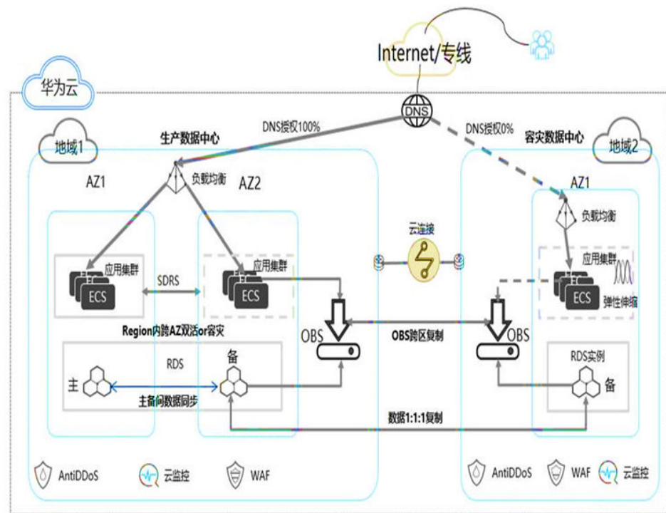
图 5-5 三 AZ 高可用设计
