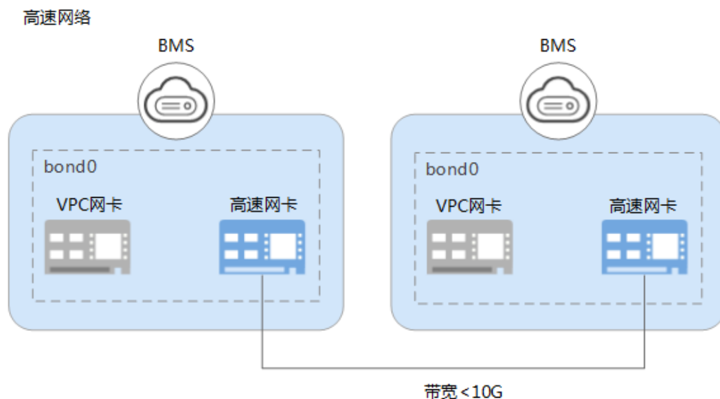
图 6-9 上一代高速网络架构
