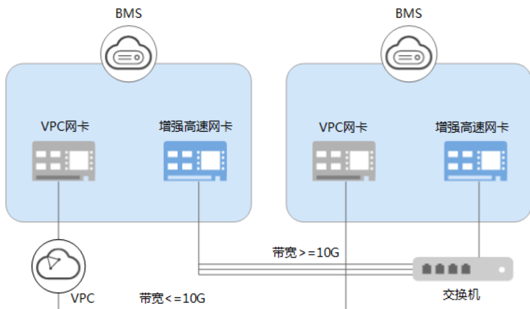
图 6-8 增强高速网络架构
