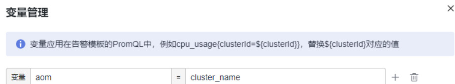
图 6-16 变量管理
