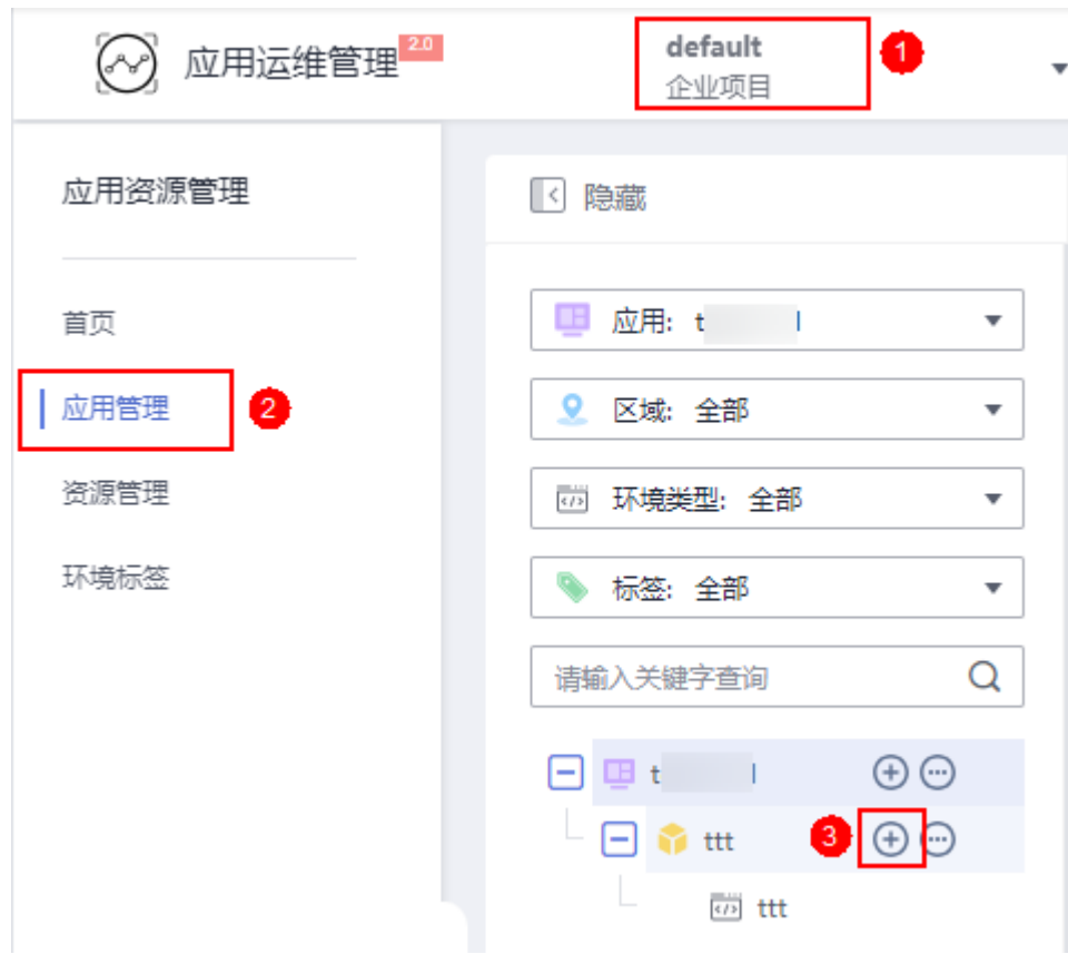
图 11-12 添加环境
