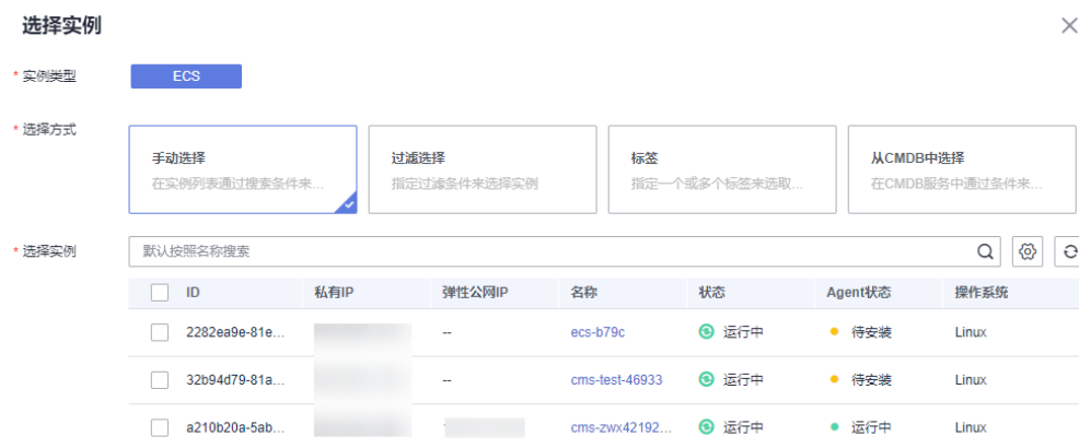
图 12-36 添加实例
