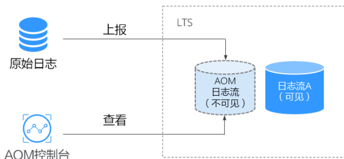
图 8-4 删除映射
