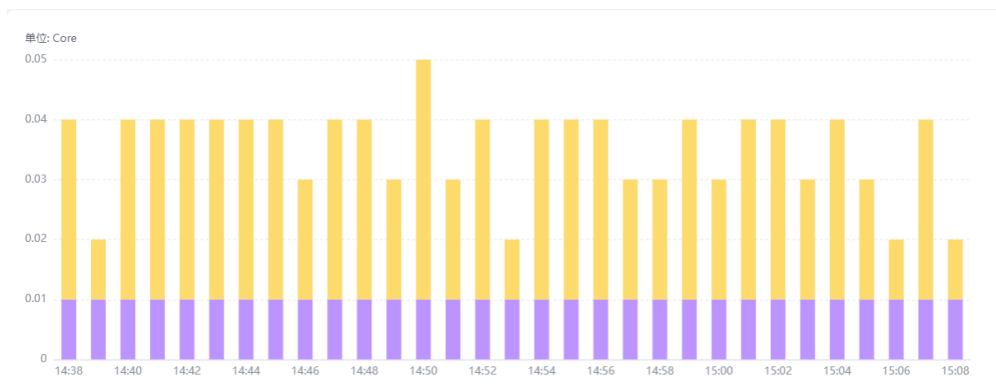
图 5-12 柱状图
