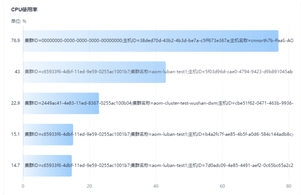
图 5-21 TopN 图
