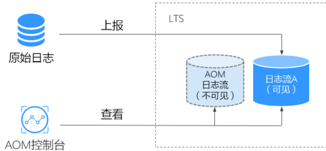
图 8-2 已创建映射
