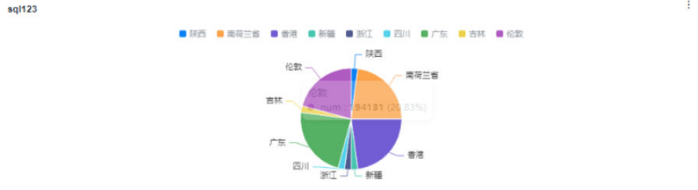
图 5-14 饼状图
