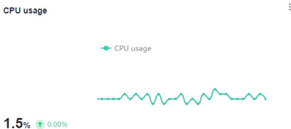
图 5-29 数字折线图
