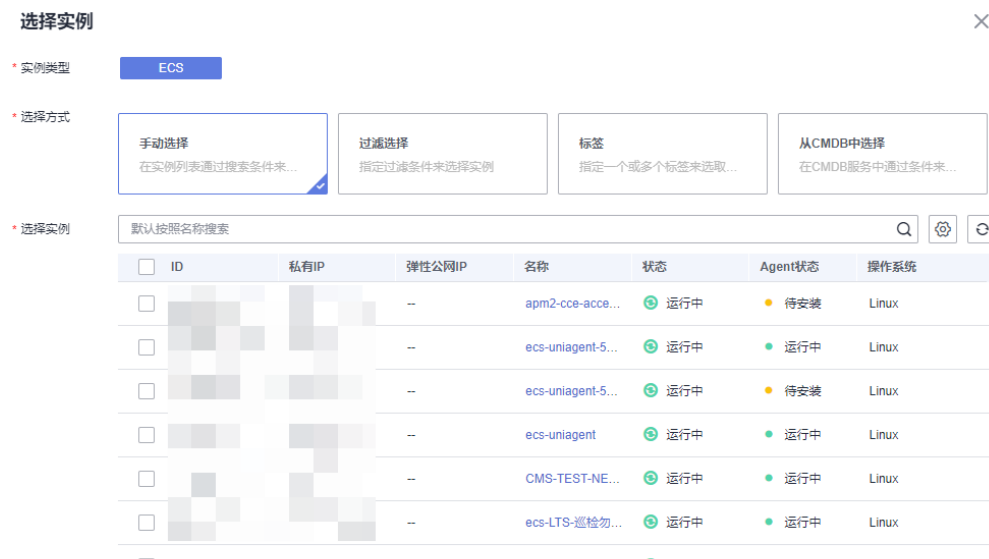
图 12-13 选择实例
