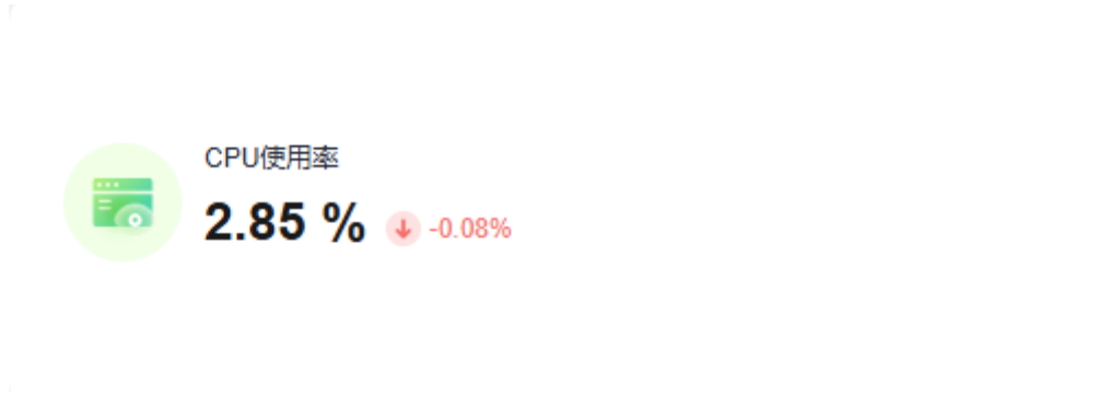
图 5-6 数字图
