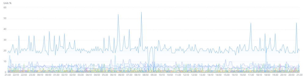
图 5-25 折线图
