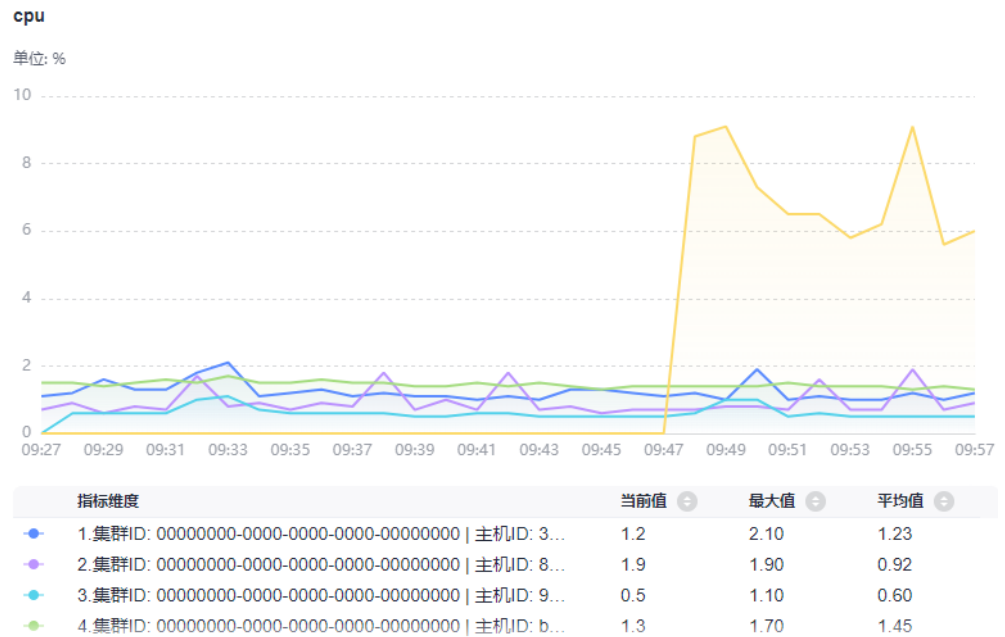
图 5-5 折线图
