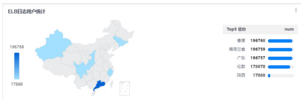
图 5-31 地图
