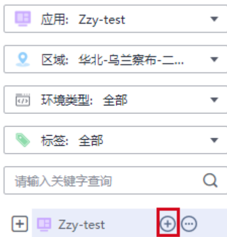
图 11-10 应用树
