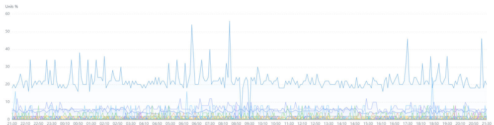
图 5-13 折线图
