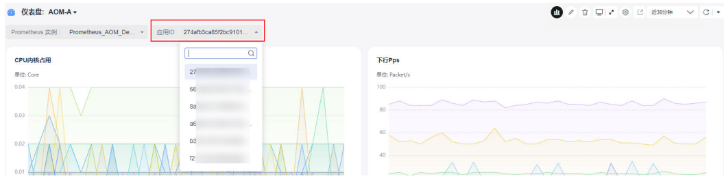
图 5-4 查看过滤器
