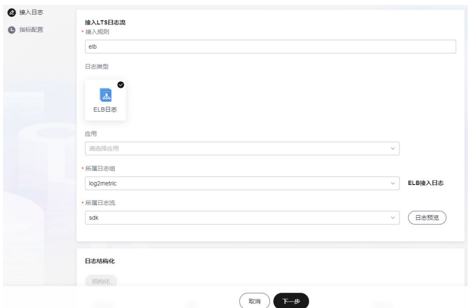
图 2-12 接入日志
