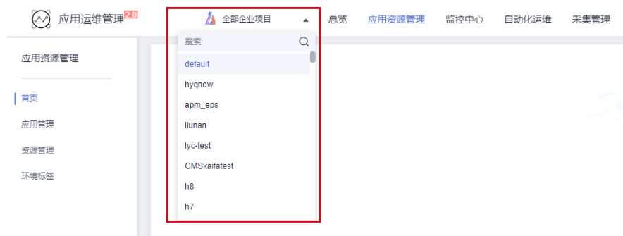
图 11-7 企业项目
