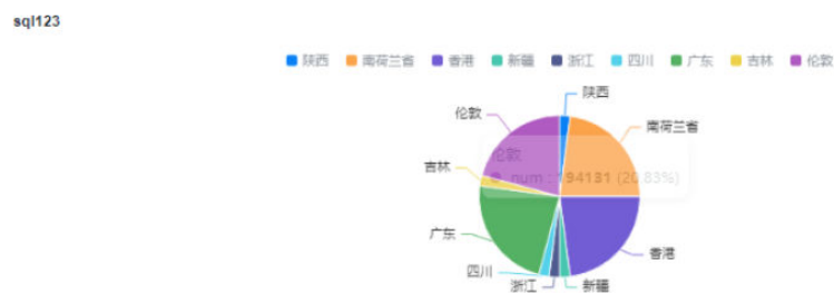
图 5-30 饼状图
