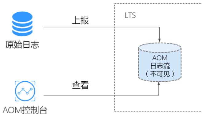
图 8-1 未创建映射
