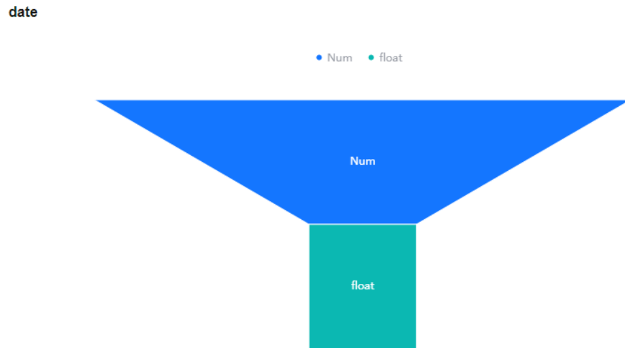
图 5-18 漏斗图
