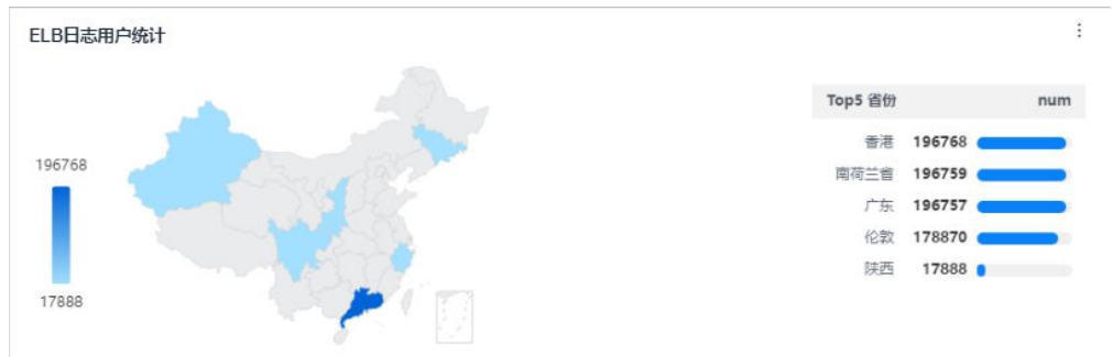
图 5-17 地图
