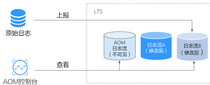
图 8-3 修改映射
