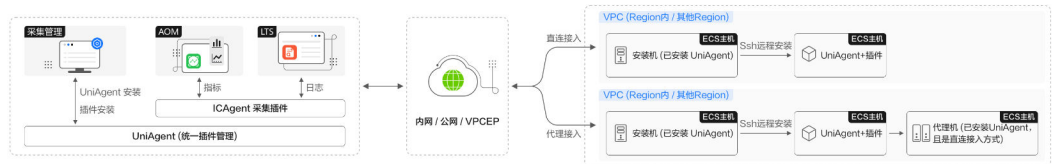
图 3-3 新手介绍
