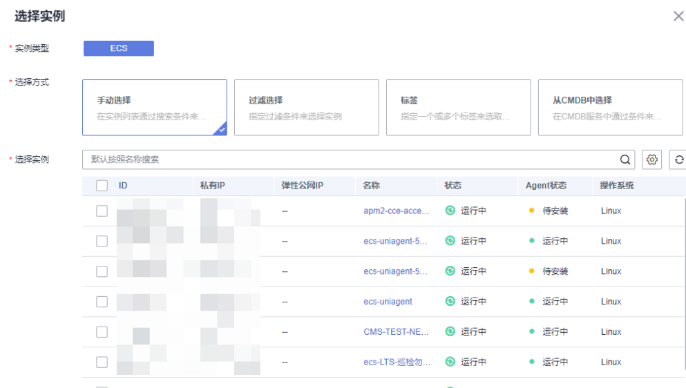
图 12-9 选择实例
