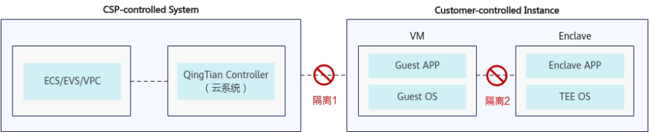
图 1-4 QingTian 机密计算
