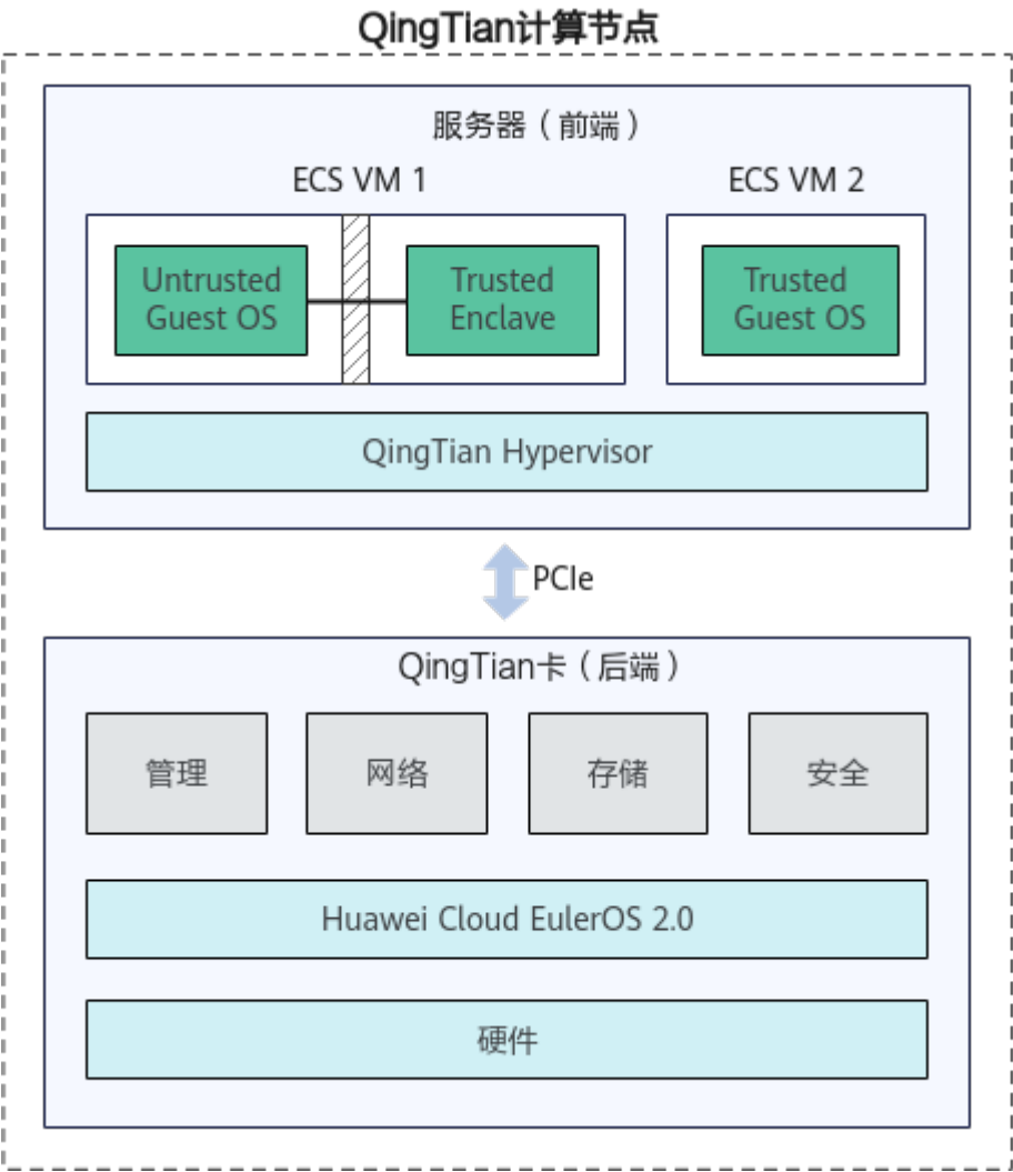
图 1-6 隔离维度 2
