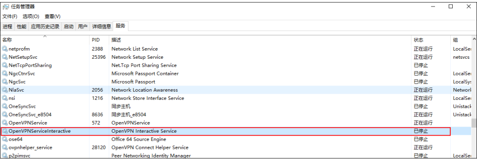
图 3-8 任务管理器
