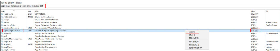
图 3-7 任务管理器
