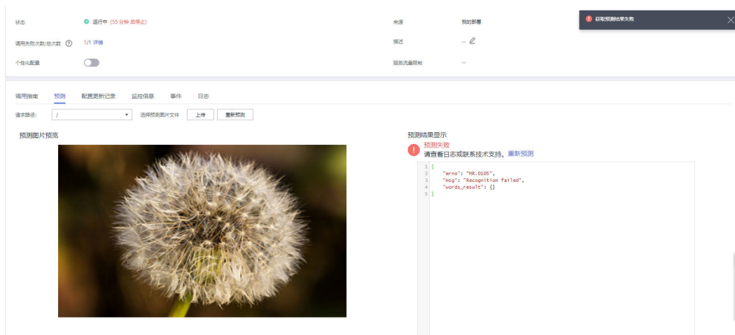
图 5-26 预测报错
