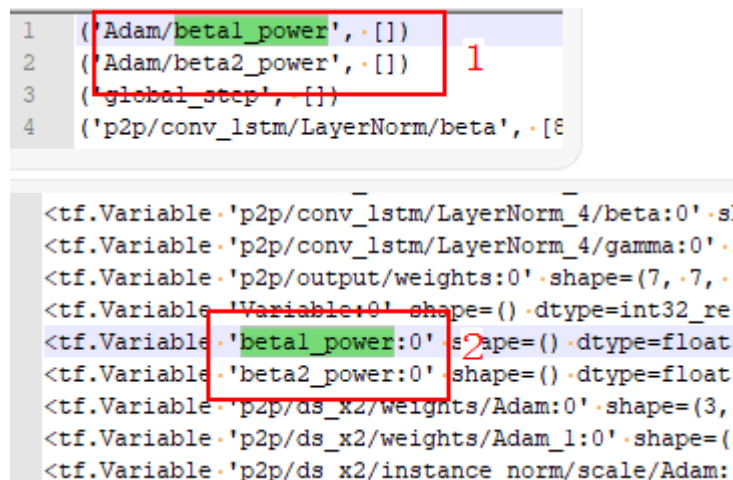
图 6-1 代码示例
