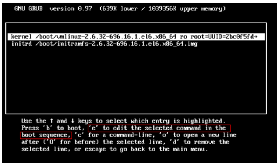
图 11-11 移动至 kernel 行
