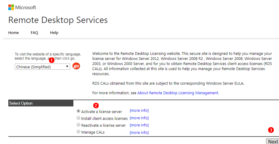
图 10-28 启用许可证服务器
