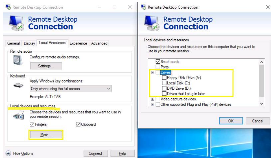
图 13-5 禁用 redirect local drives 功能
