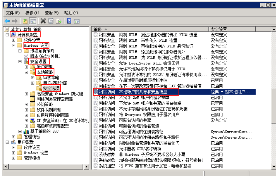
图 4-42 打开网络访问策略
