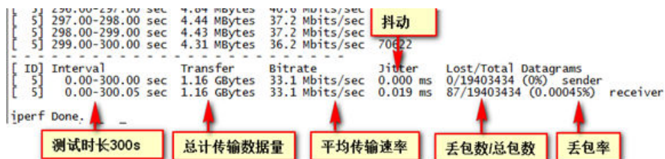
图 14-149 UDP PPS 测试结果
