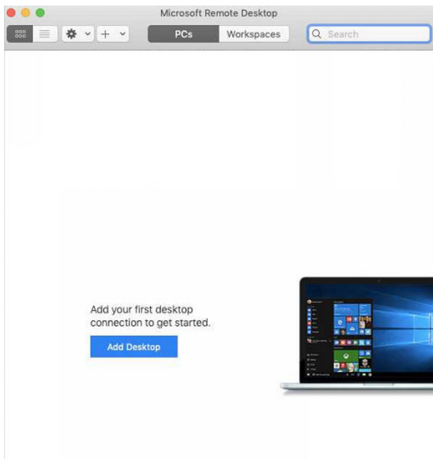
图 14-81 Add Desktop
