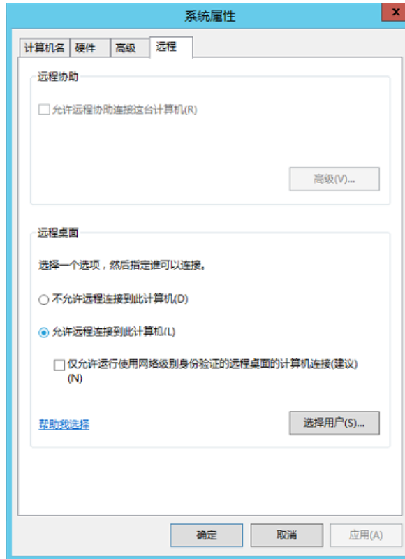
图 3-8 系统属性
