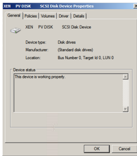
图 14-109 磁盘属性
