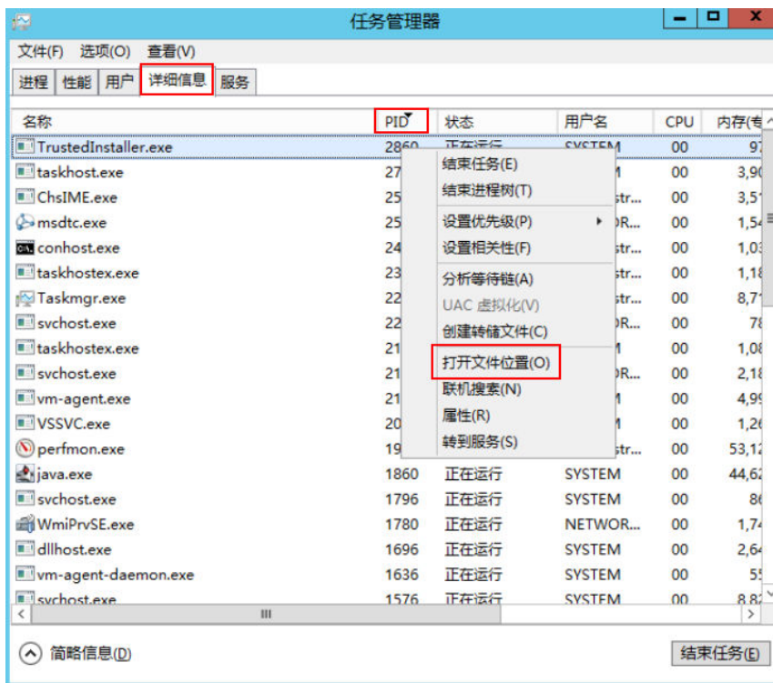
图 14-155 检查进程
