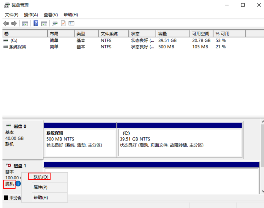
图 14-96 磁盘联机
