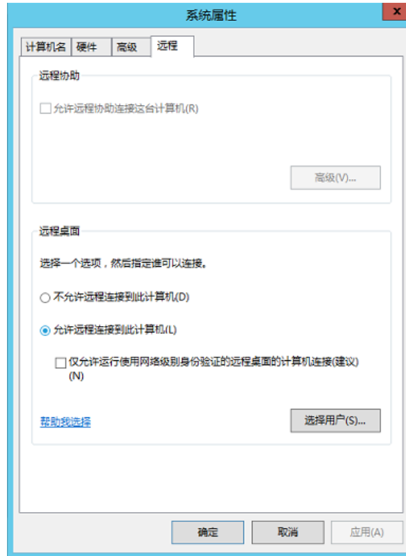
图 3-7 系统属性
