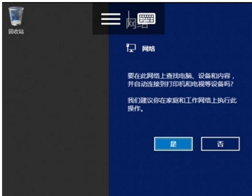
图 3-14 登录成功
