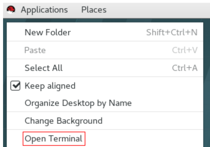
图 14-111 open terminal
