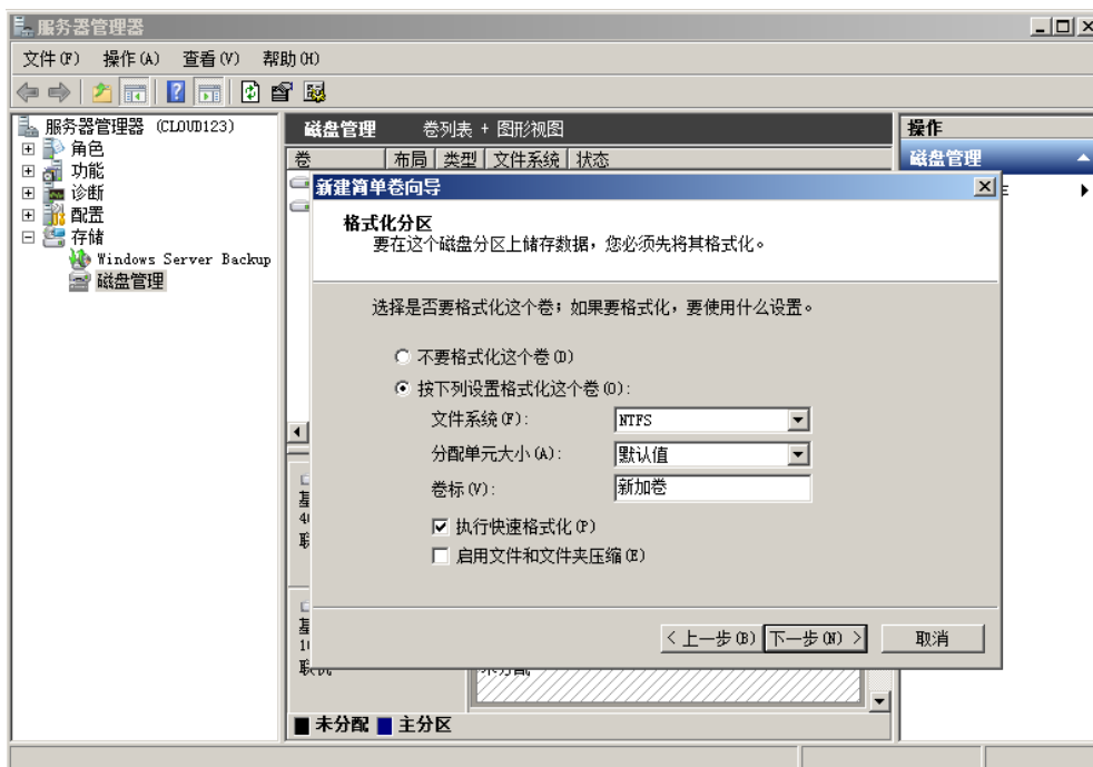
图 2-9 格式化分区
