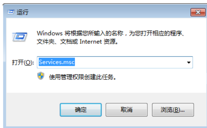
图 14-125 运行
