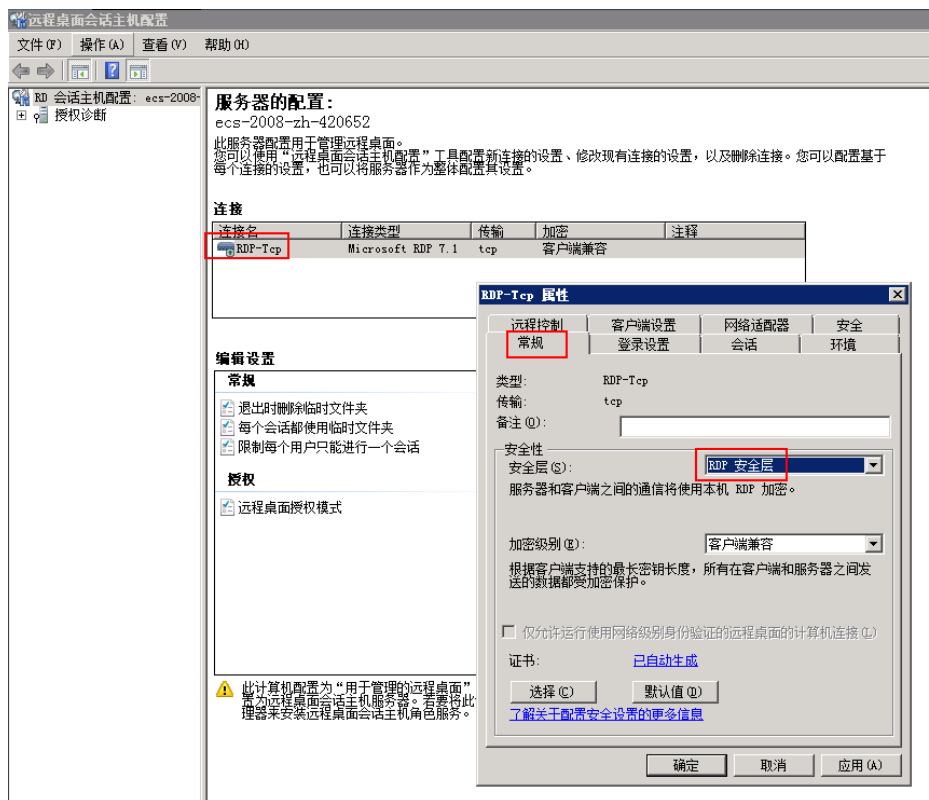
图 14-46 RDP-TCP 属性
