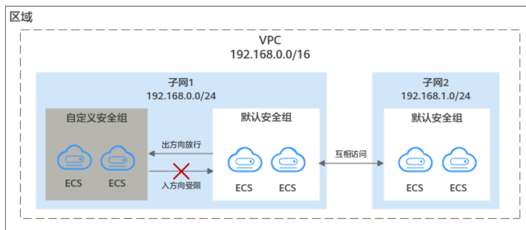
图 1-2 默认安全组
