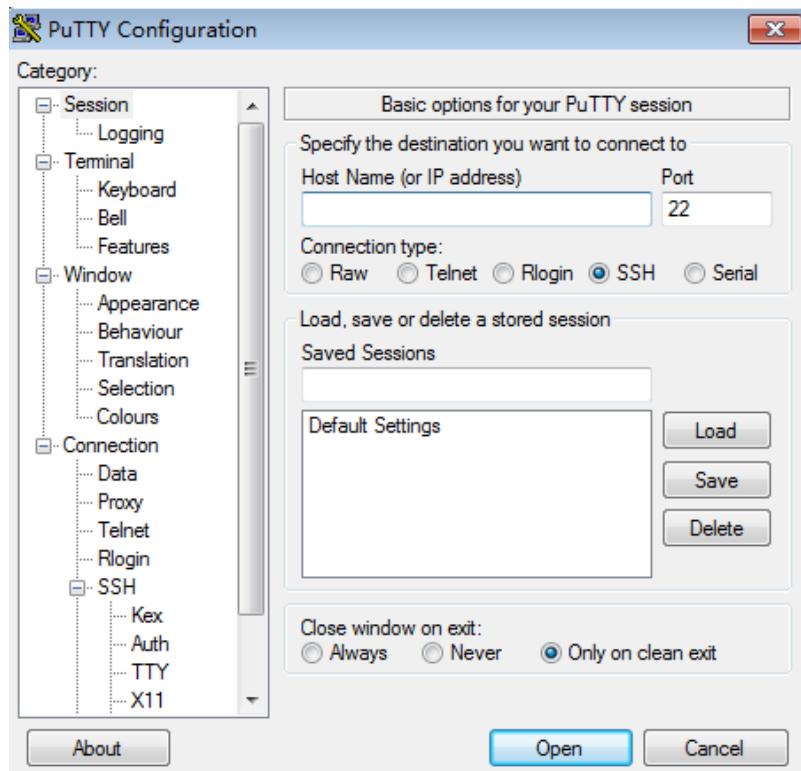
图 3-21 单击“Session”
