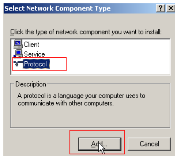
图 7-14 添加协议
