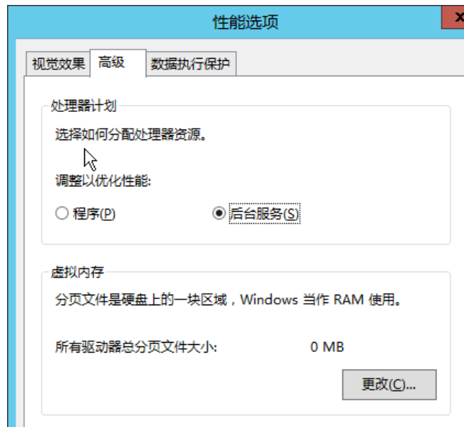
图 14-113 性能选项
