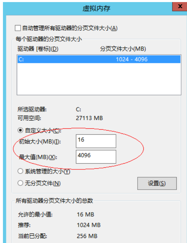
图 14-114 虚拟内存
