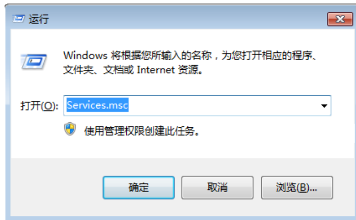
图 14-122 运行
