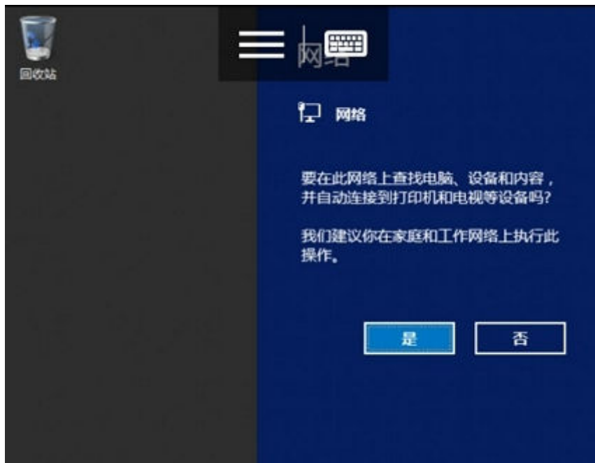
图 3-19 登录成功
