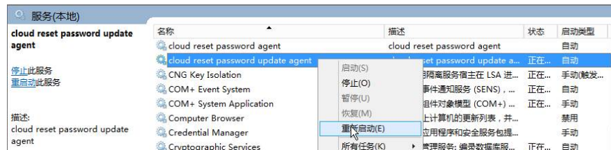
图 14-123 服务（本地）
