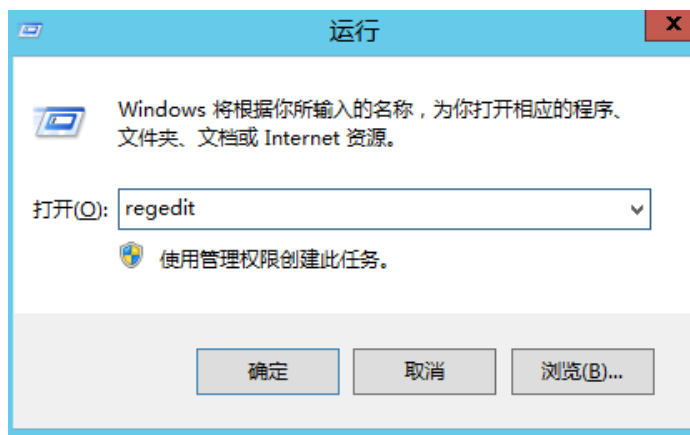
图 14-43 打开注册表
