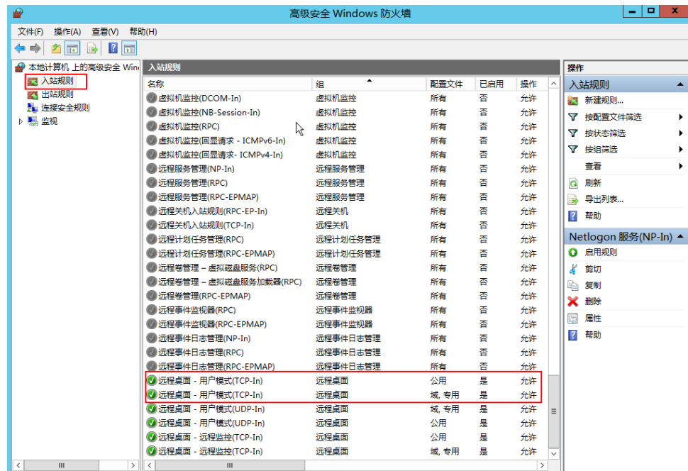
图 14-12 进站规则
