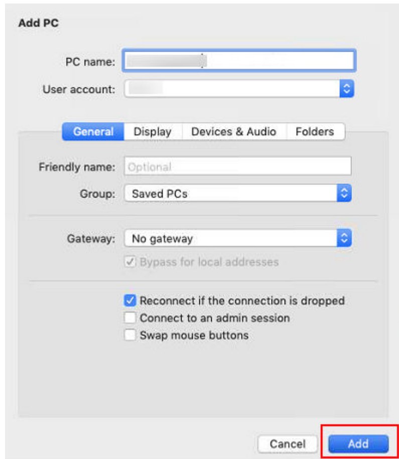
图 3-17 Add PC
