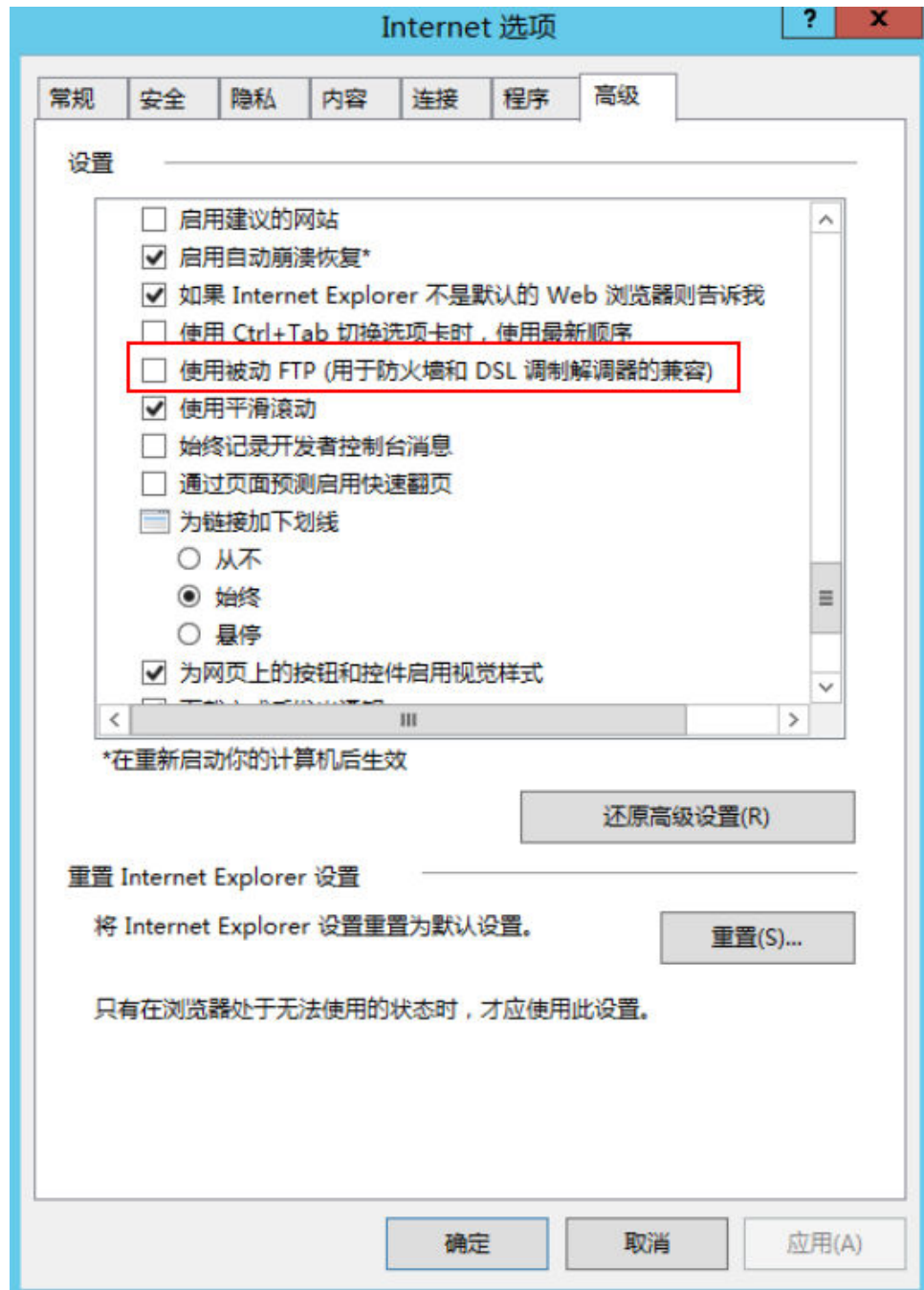
图 14-93 Internet 选项
