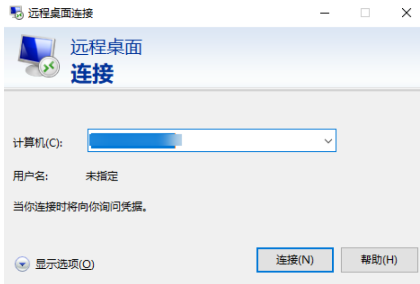
图 3-2 显示选项
