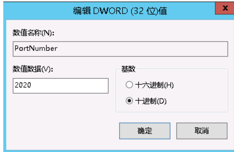
图 14-4 修改为 2020 端口
