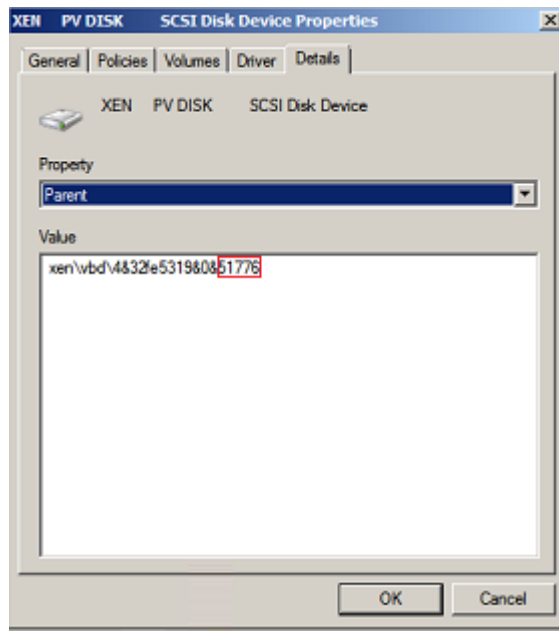
图 14-110 详细信息
