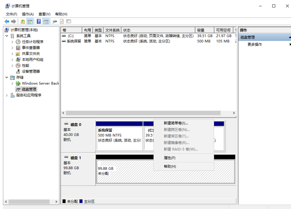
图 2-15 计算机管理
