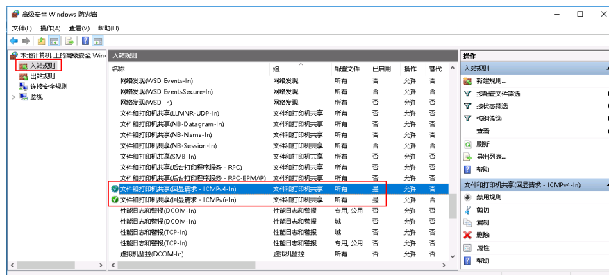
图 14-138 进站规则
