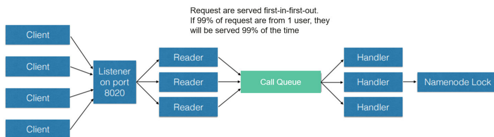
图 10-4 基于 FIFO 调用队列的 NameNode 请求处理
