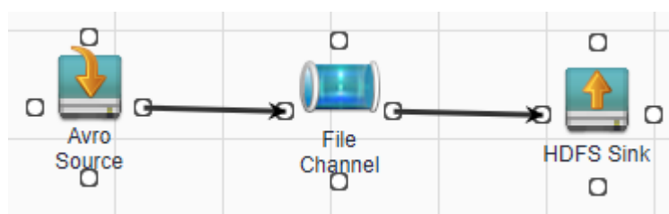
图 6-17 Flume 配置工具示例
