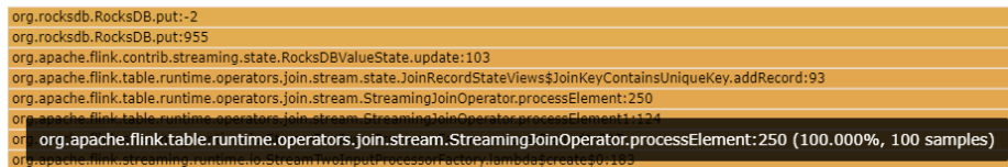
图 5-4 通过火焰图查看算子热点
