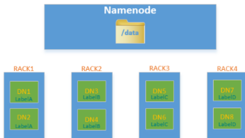
图 10-7 场景样例
