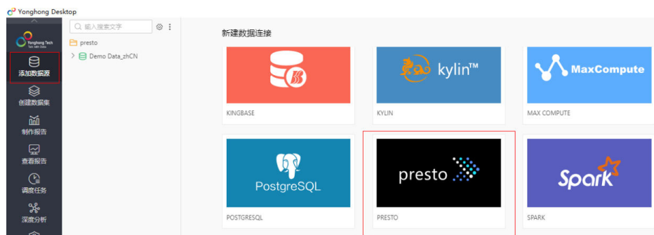
图 9-40 打开 presto
