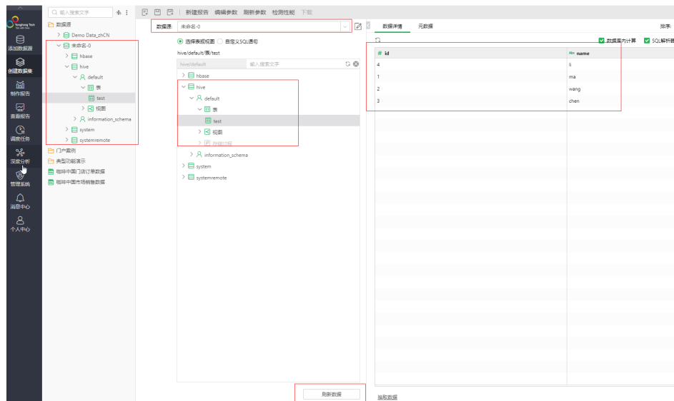
图 9-45 查看表信息
