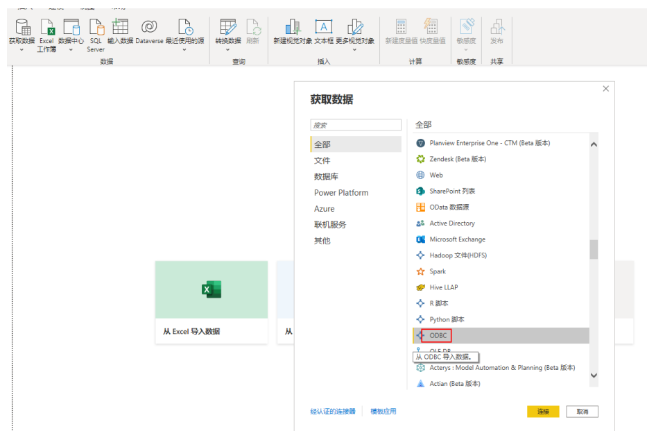
图 9-36 选择 ODBC
