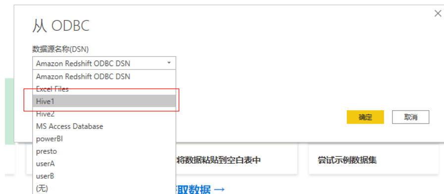
图 9-37 添加数据源
