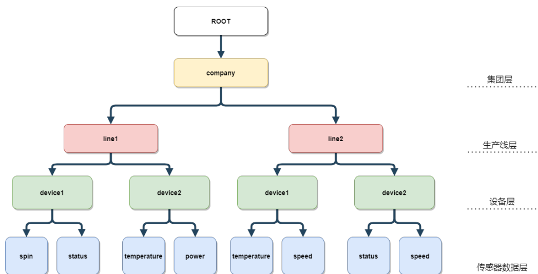
图 13-1 数据结构
