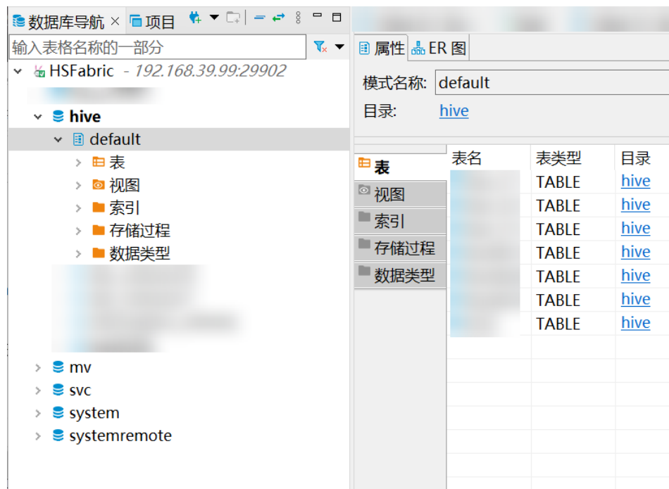
图 9-15 连接成功
