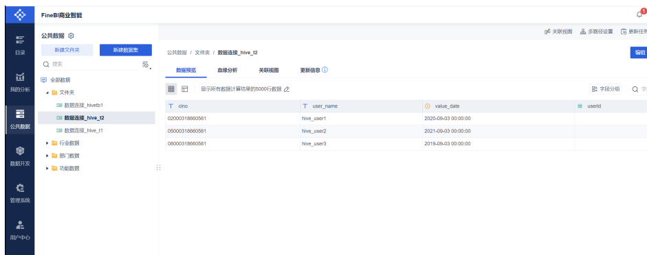
图 9-19 数据预览
