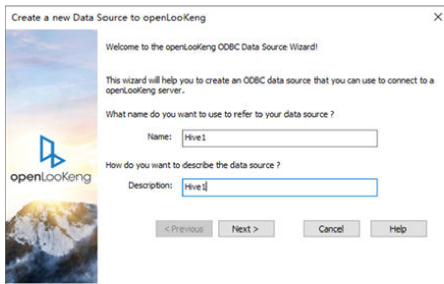
图 9-31 填写名称
