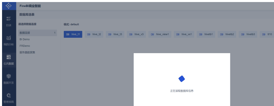
图 9-18 选择数据库
