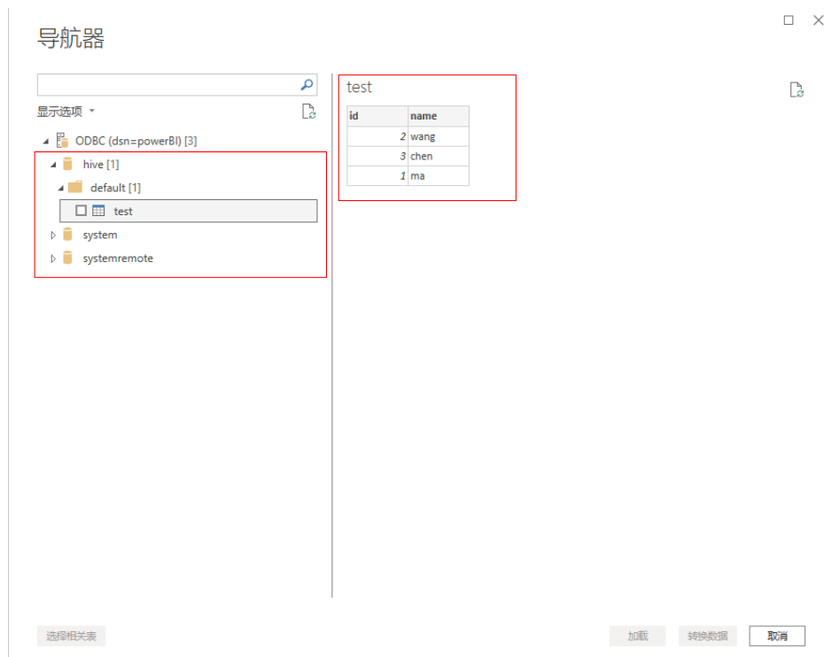
图 9-39 连接成功
