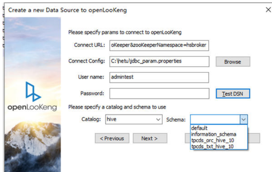
图 9-34 查看内容
