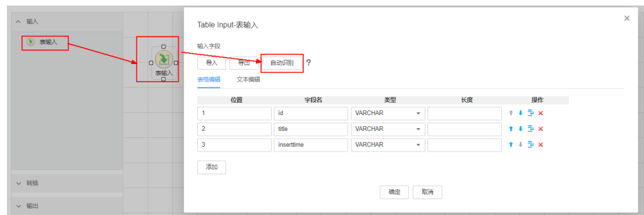
图 16-30 算子输入
