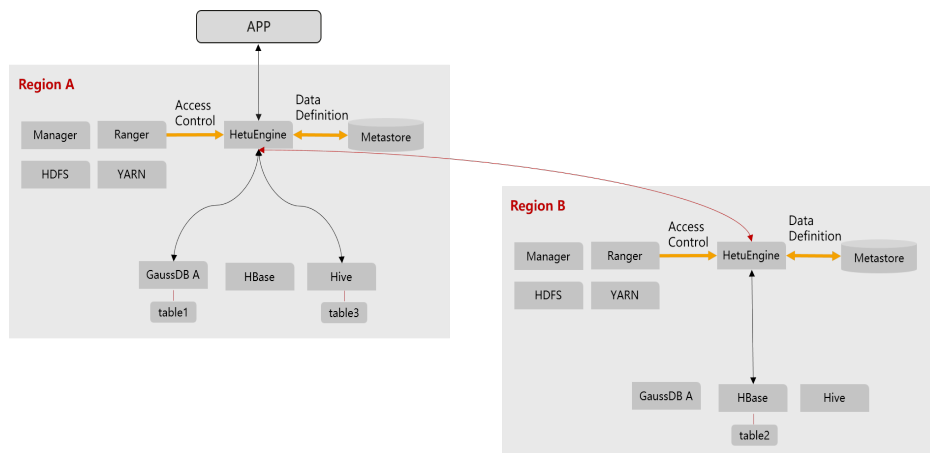
图 9-9 HetuEngine 跨域功能示意
