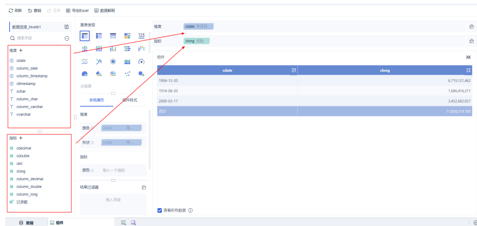
图 9-25 分析表
