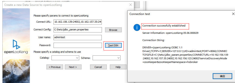
图 9-33 测试连接
