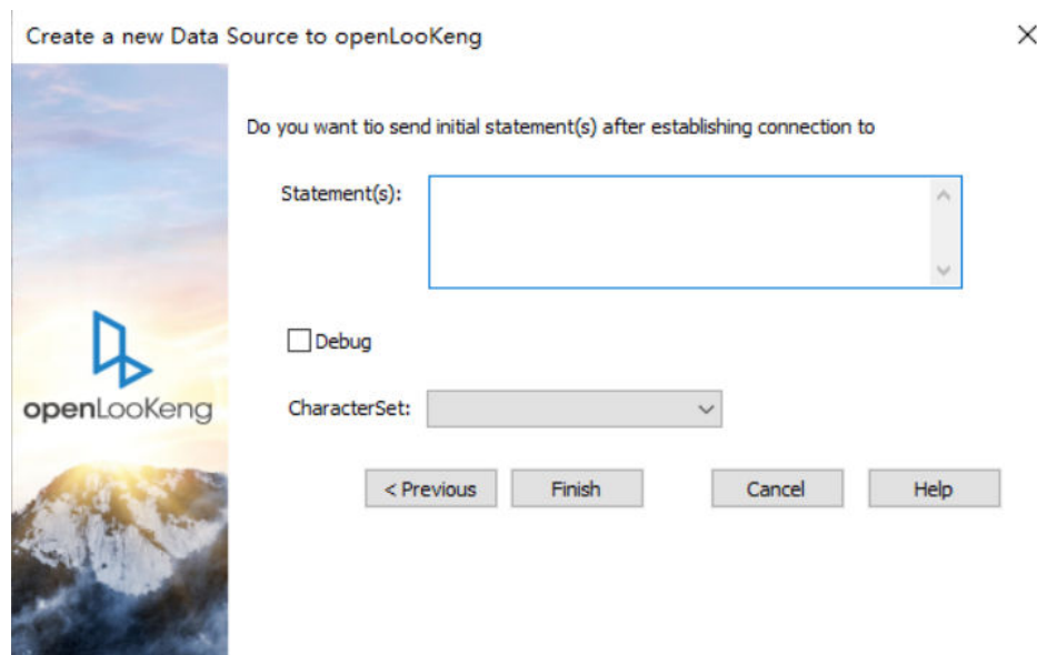
图 9-35 完成连接
