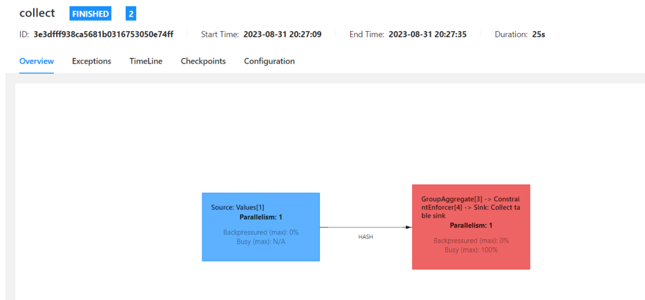
图 5-7 作业任务
