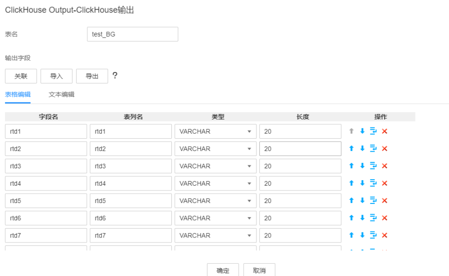
图 16-31 算子输出
