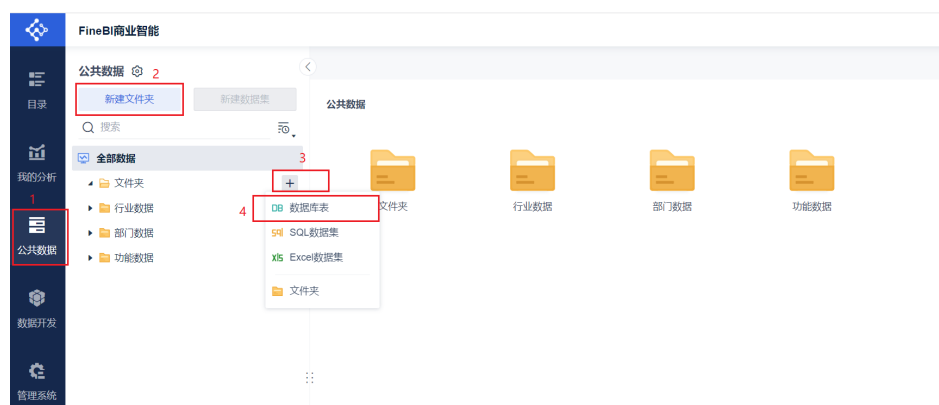
图 9-16 配置数据
