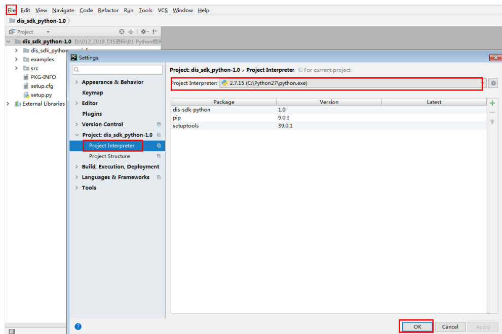
图 6-4 添加 python
