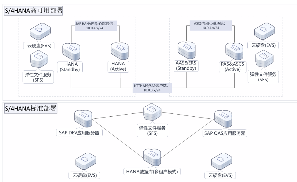
图 1-1 方案架构
