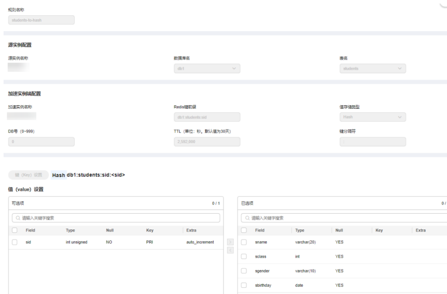
图 6-171 配置映射规则
