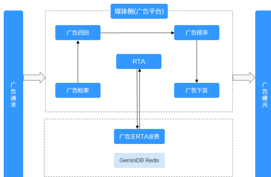
图 9-1 RTA 广告流程
