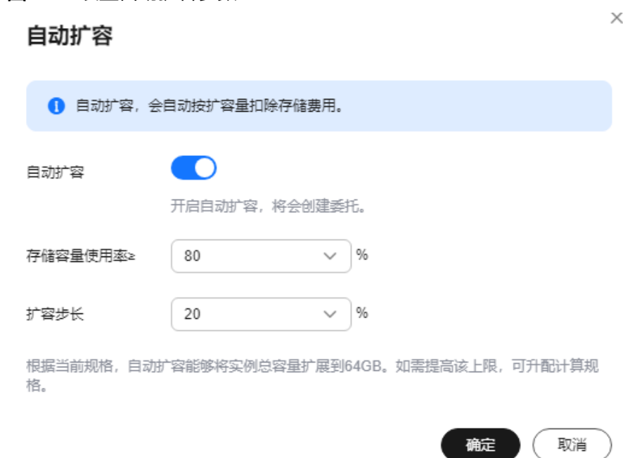
图 6-26 设置自动扩容参数
