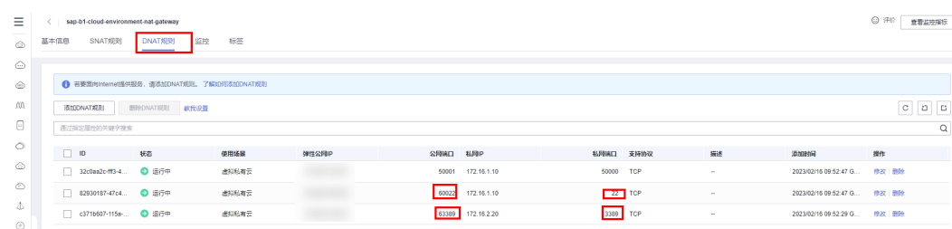
图 3-19 DNAT 映射
