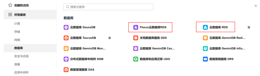
图 1-5 选择服务
