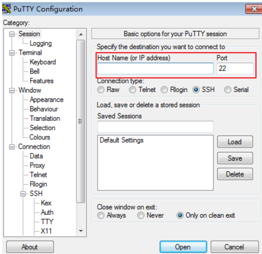
图 2-9 PuTTY 配置
