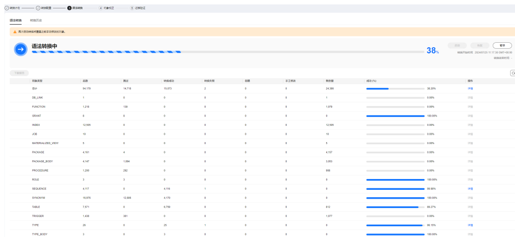
图 2-6 语法转换
