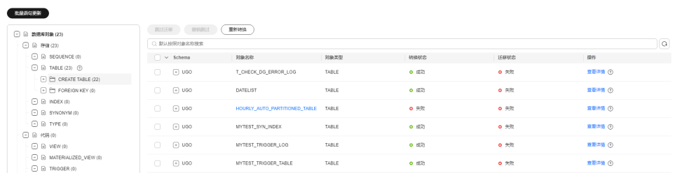
图 2-7 对象校正
