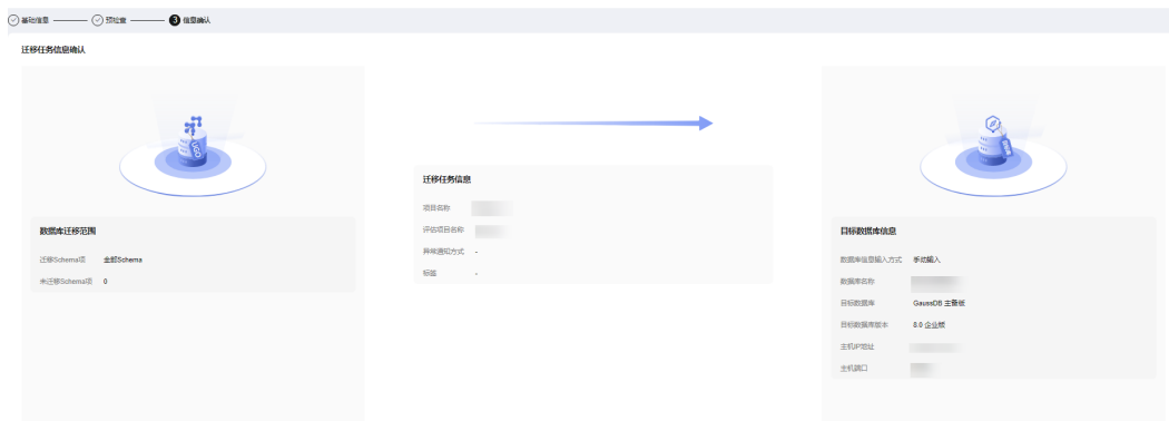
图 2-3 信息确认
