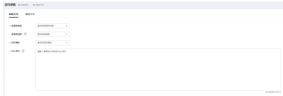
图 3-5 审核文本
