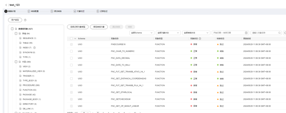
图 2-4 转换计划
