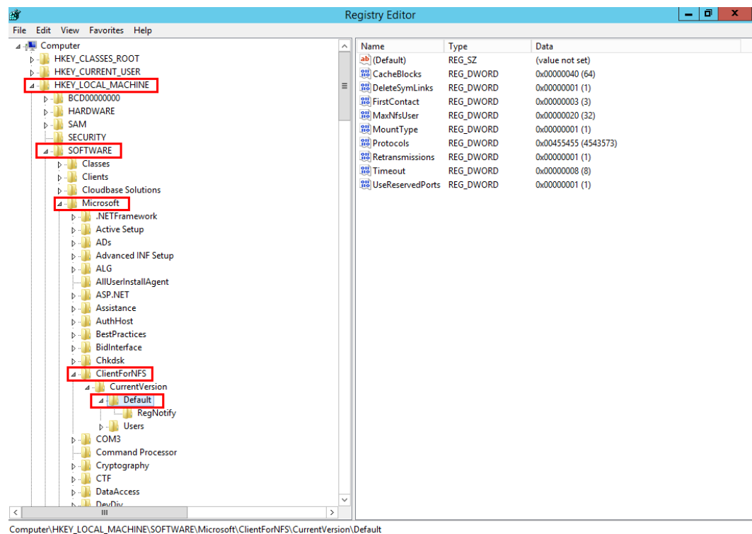
图 4-12 进入目录
