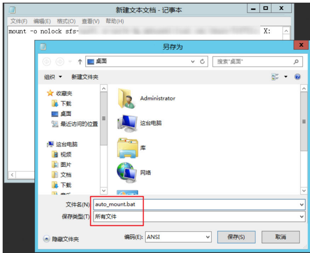
图 4-16 保存脚本
