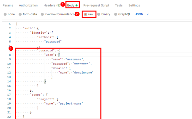
图 3-2 Token 认证鉴权
