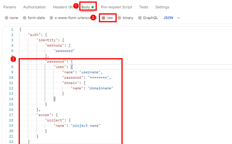
图 3-5 Token 认证鉴权
