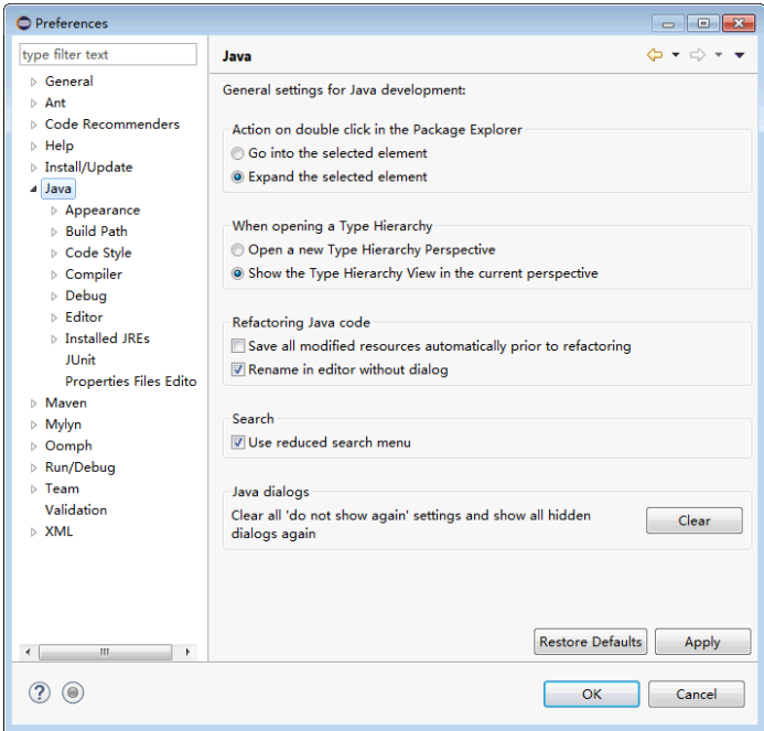
图 3-1 Preferences
