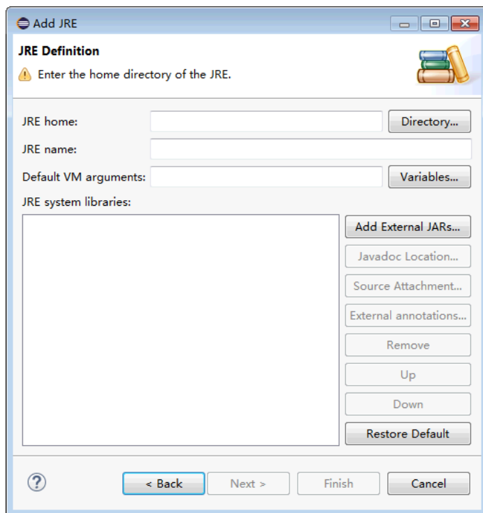
图 3-4 JRE Definition
