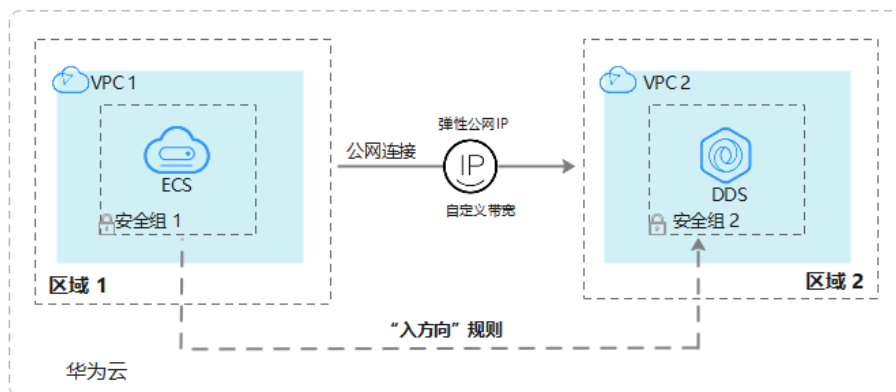
图 3-30 不同区域 ECS 访问 DDS
