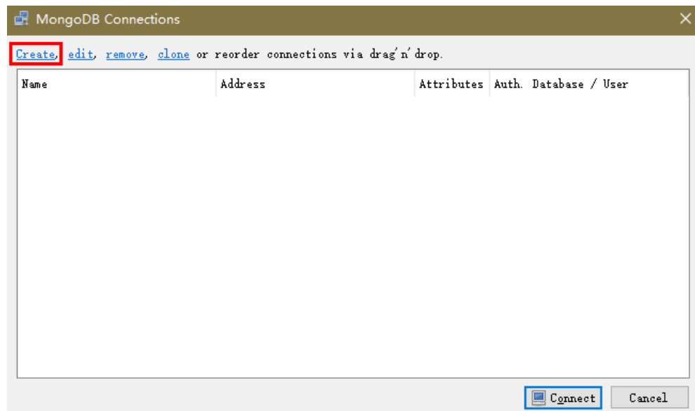
图 3-37 连接信息
