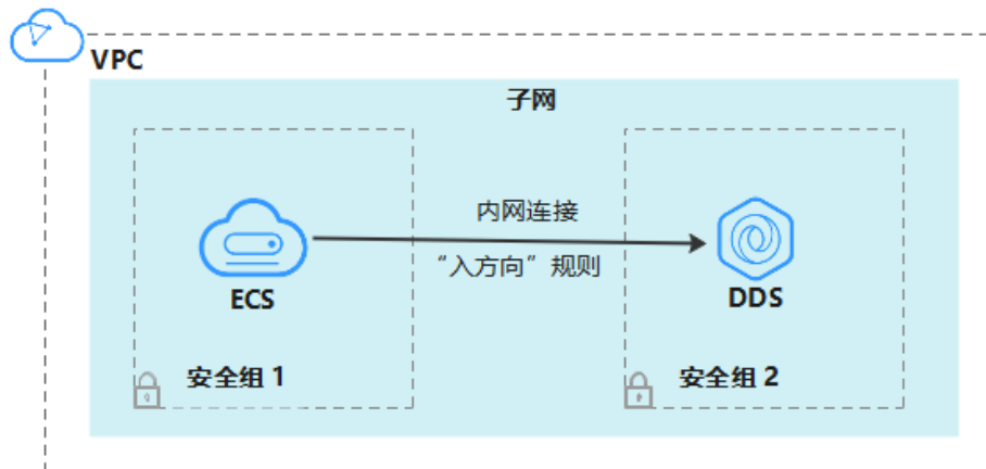
图 2-8 不同安全组
