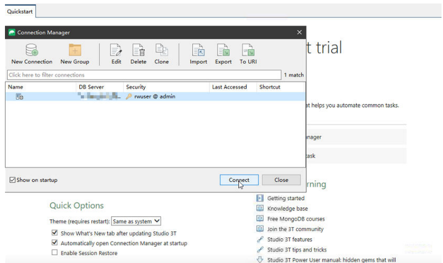
图 6-41 连接信息
