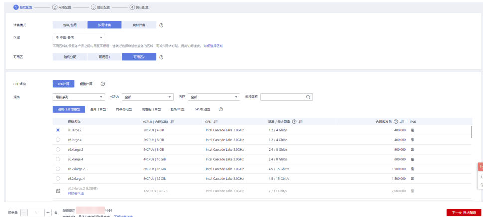
图 6-5 基础配置
