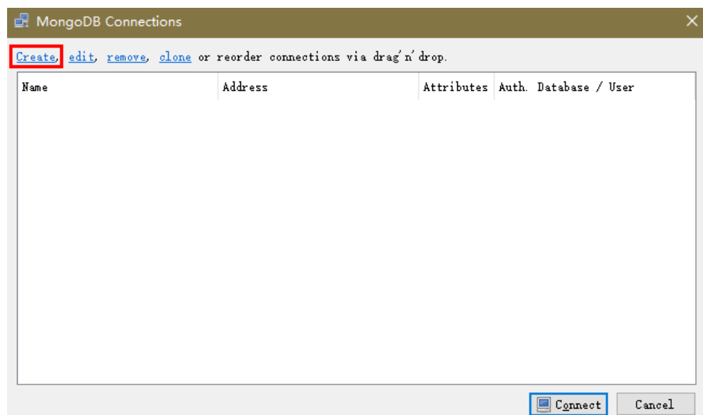
图 2-45 连接信息
