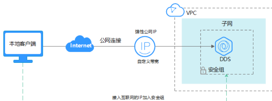
图 4-22 连接示意图
