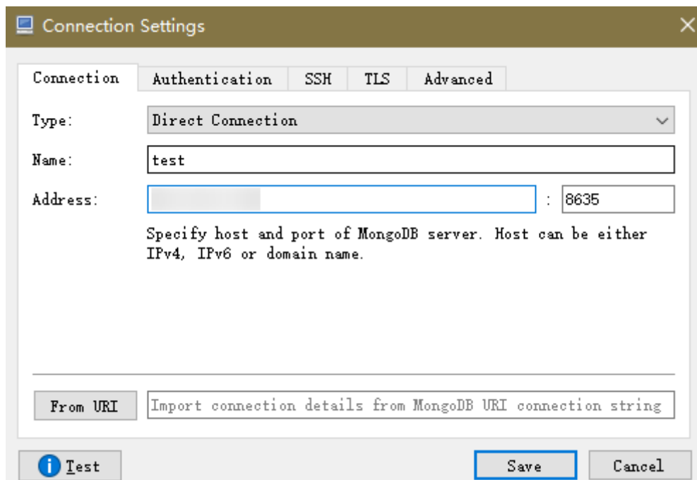
图 4-30 Connection
