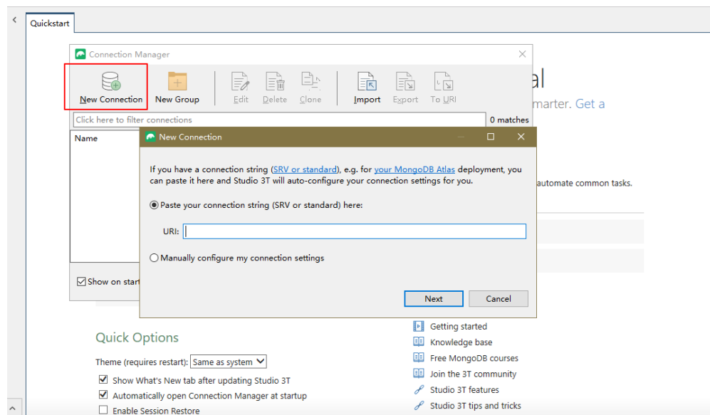
图 6-33 连接管理器
