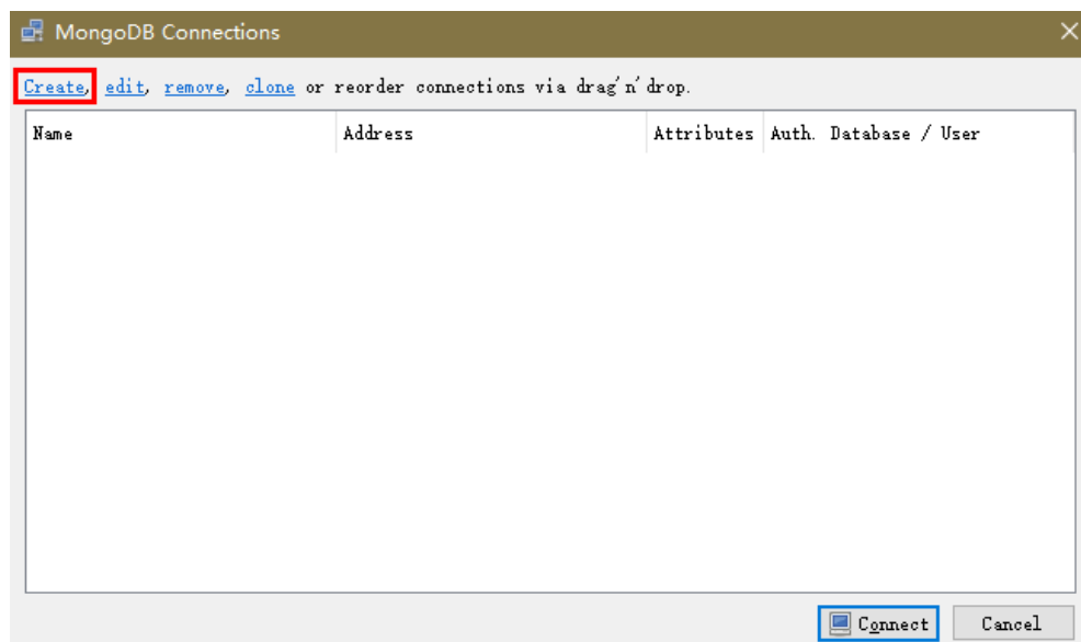
图 2-39 连接信息
