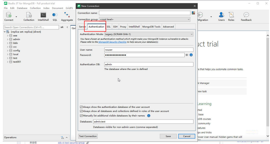
图 6-36 连接 Authentication
