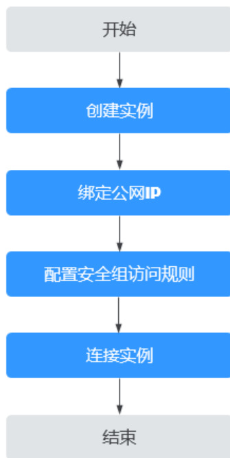
图 1-1 使用流程
