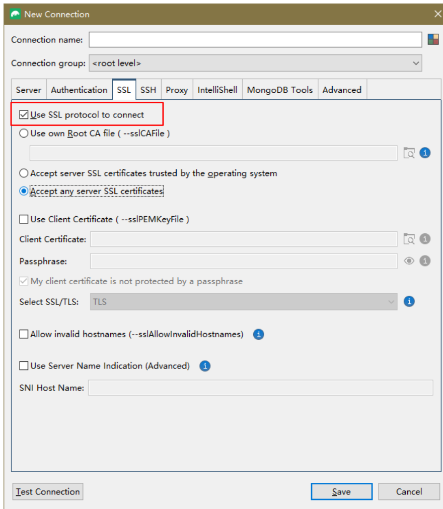
图 6-48 连接 SSL
