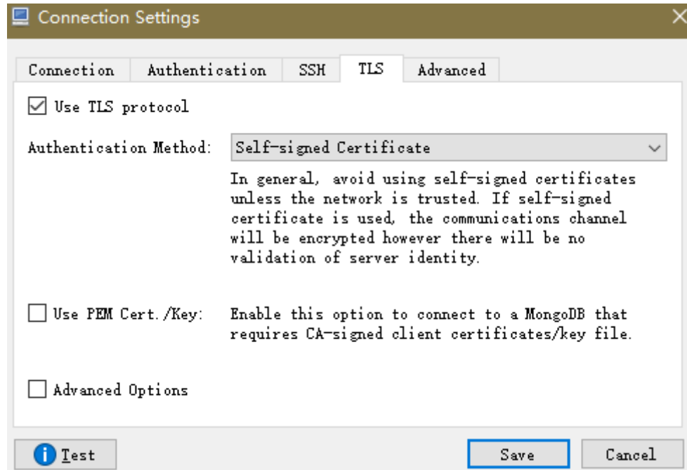
图 4-26 SSL
