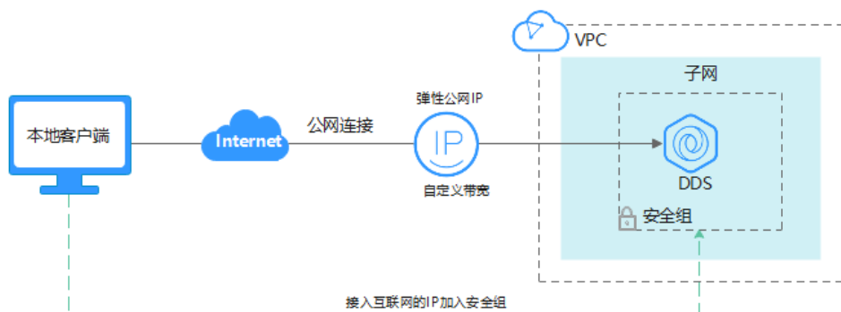
图 2-38 连接示意图
