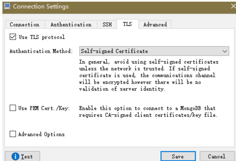
图 2-42 SSL
