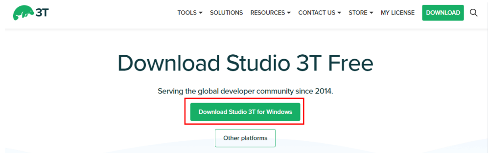
图 6-31 下载工具
