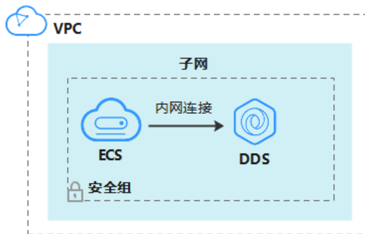
图 2-7 相同安全组
