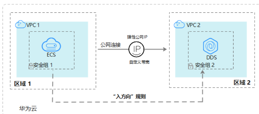
图 4-16 不同区域 ECS 访问 DDS
