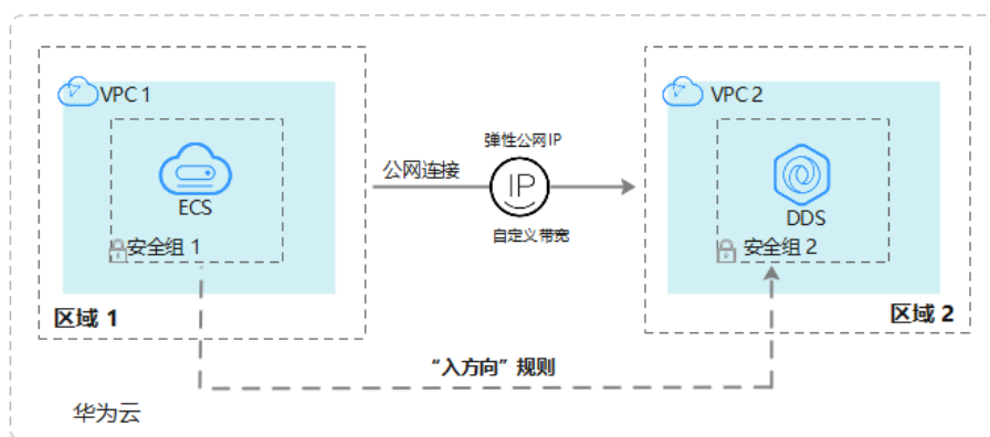
图 2-30 不同区域 ECS 访问 DDS
