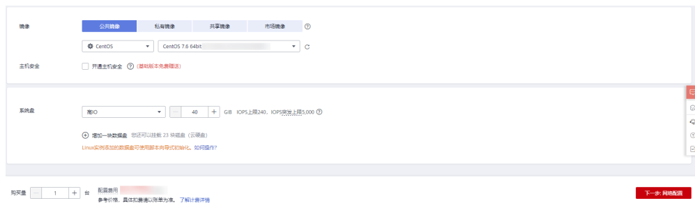
图 6-6 选择镜像
