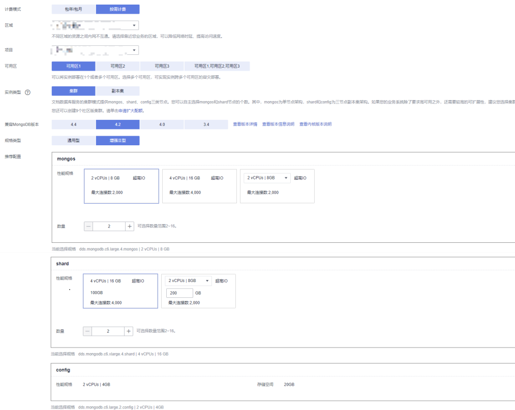
图 2-1 基础配置
