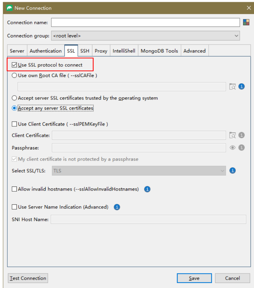
图 6-38 连接 SSL
