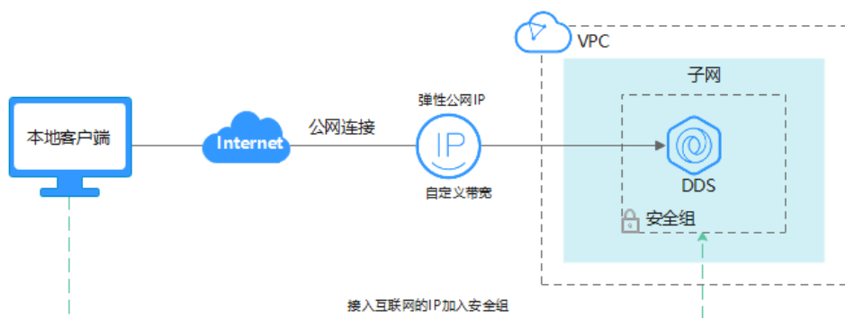
图 3-36 连接示意图
