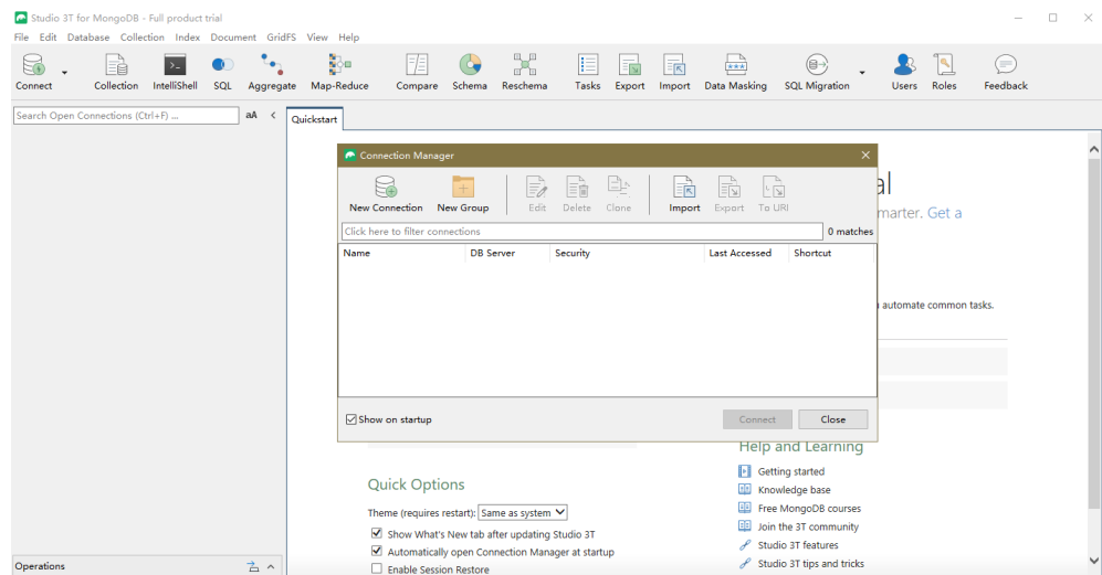
图 6-32 工具主界面
