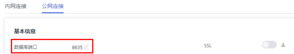
图 4-21 获取端口号
