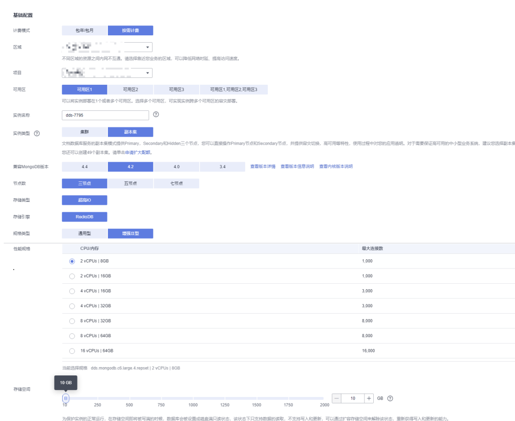
图 3-3 基础配置
