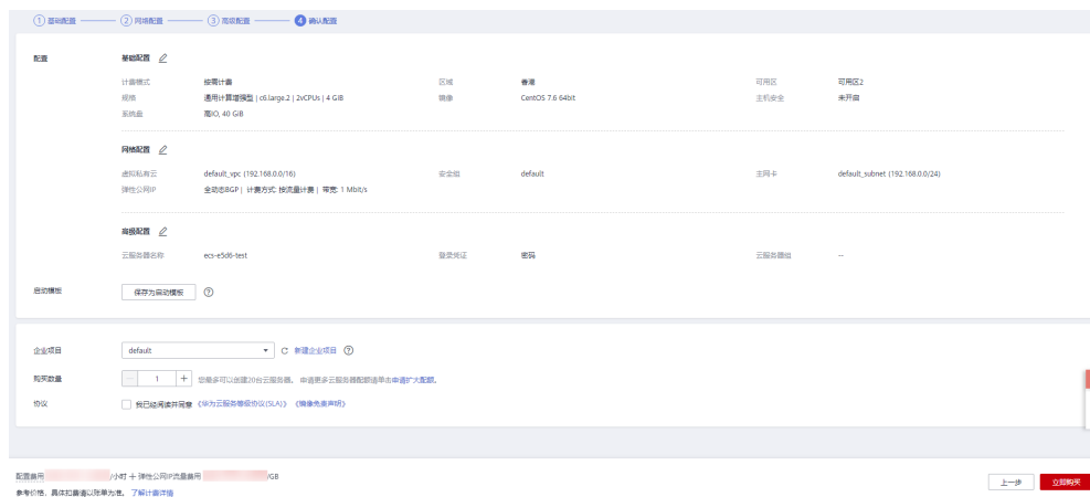
图 6-10 确认配置
