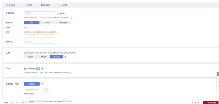
图 6-9 高级配置
