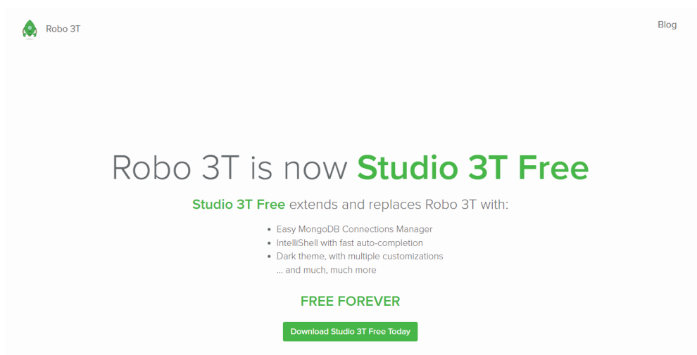
图 6-30 下载页面
