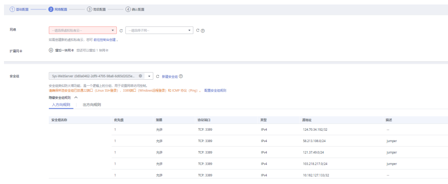
图 6-7 网络配置
