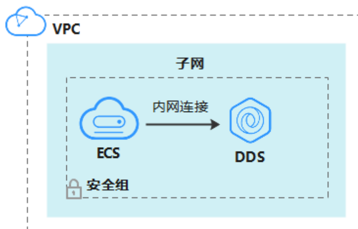
图 3-8 相同安全组
