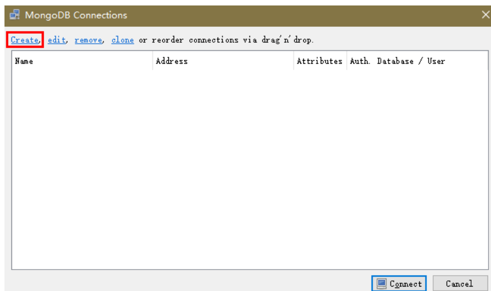
图 3-43 连接信息
