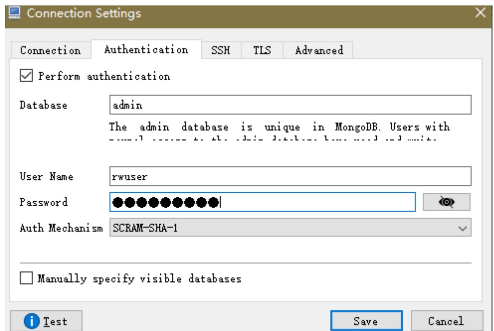
图 3-45 Authentication
