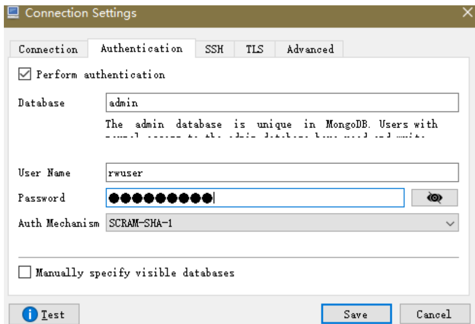
图 4-25 Authentication
