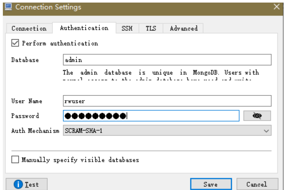
图 3-39 Authentication
