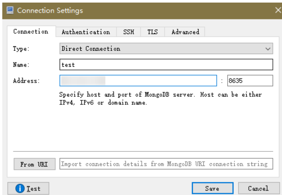
图 2-46 Connection
