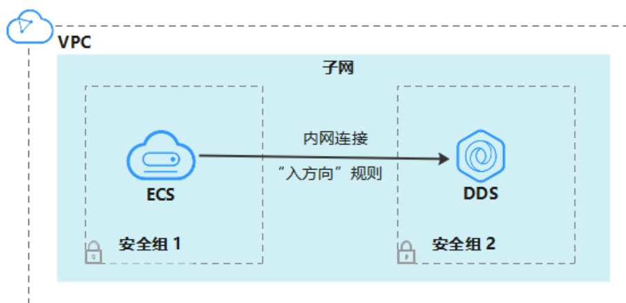
图 3-9 不同安全组
