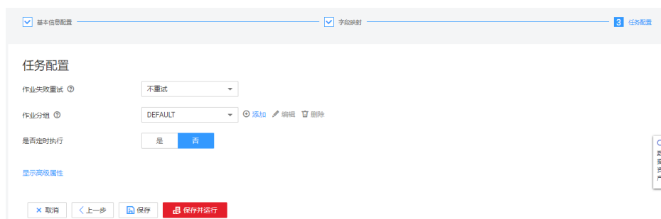
图 4-14 任务配置
