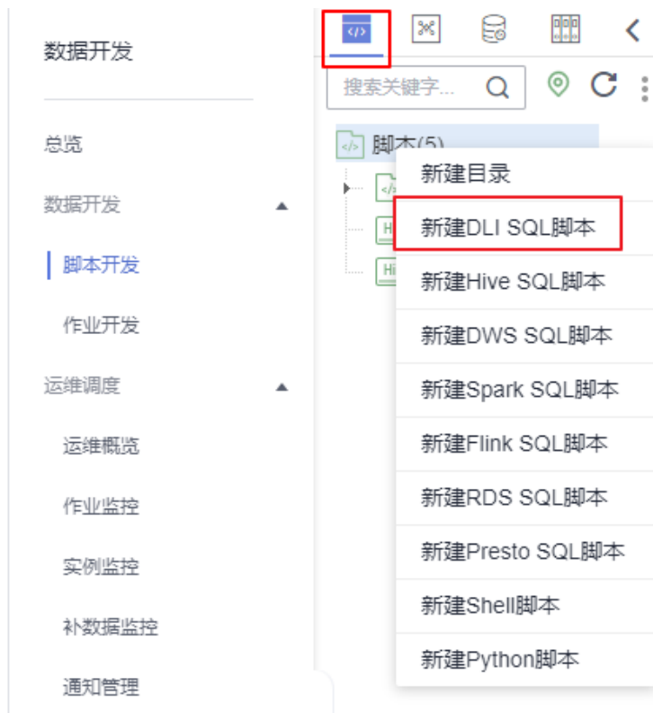
图 2-10 新建脚本
