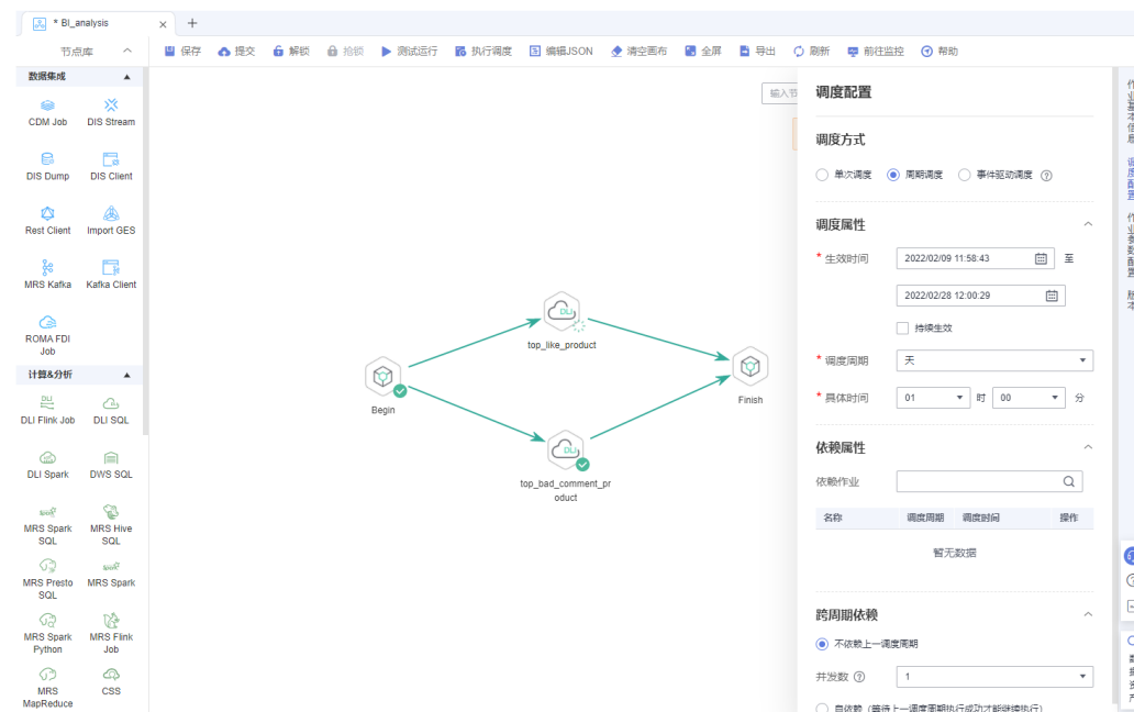
图 2-16 调度配置
