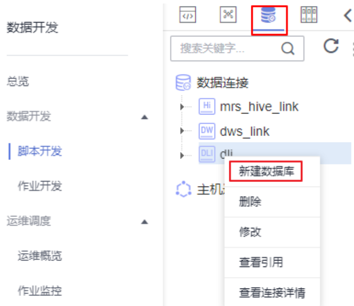
图 2-4 创建数据库
