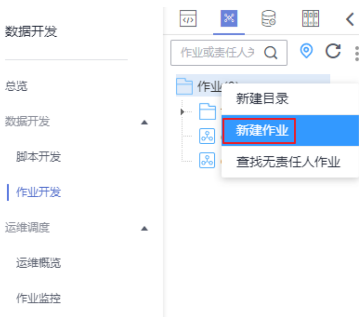
图 2-13 新建作业
