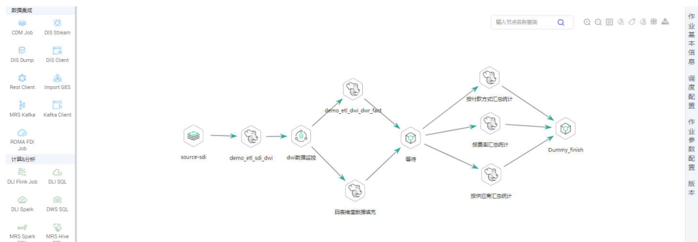
图 4-86 编排作业
