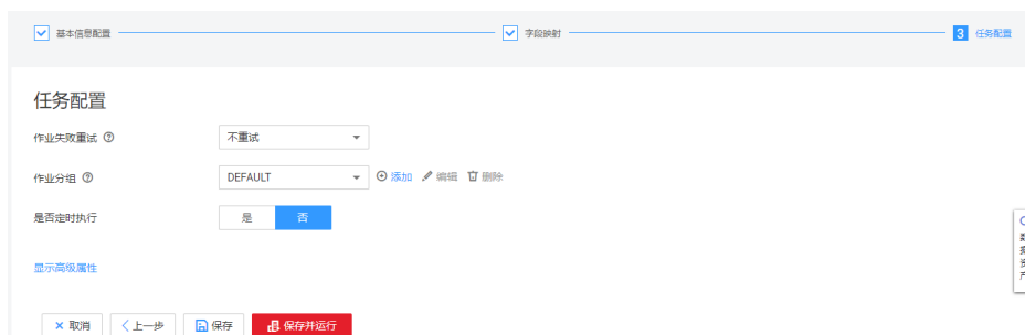
图 4-14 任务配置
