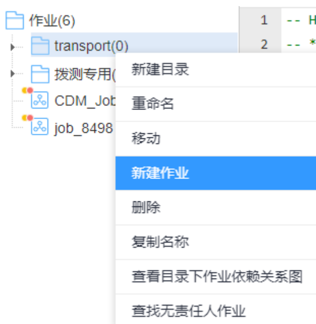
图 4-84 作业
