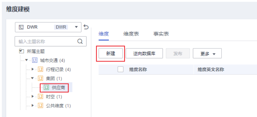
图 4-59 维度建模
