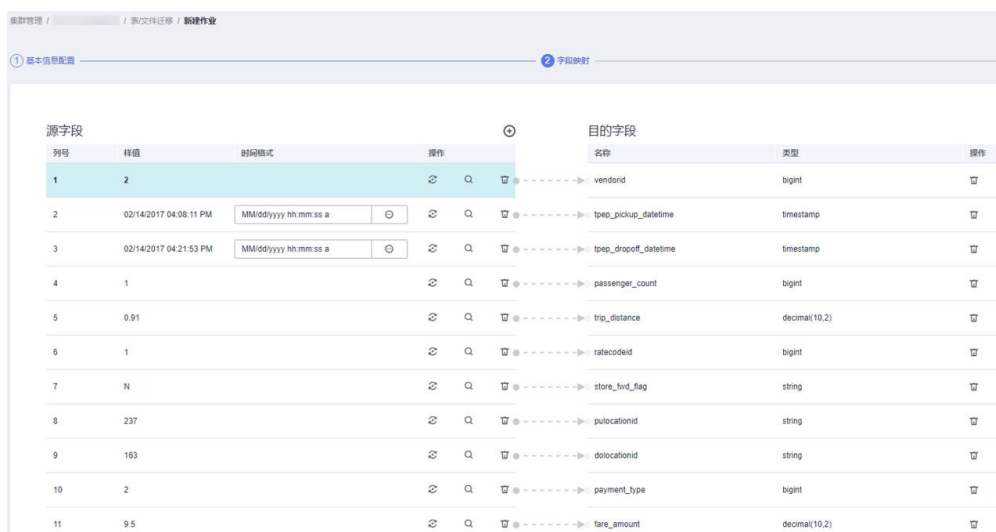
图 4-13 字段映射
