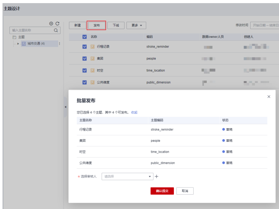
图 4-32 发布主题域
