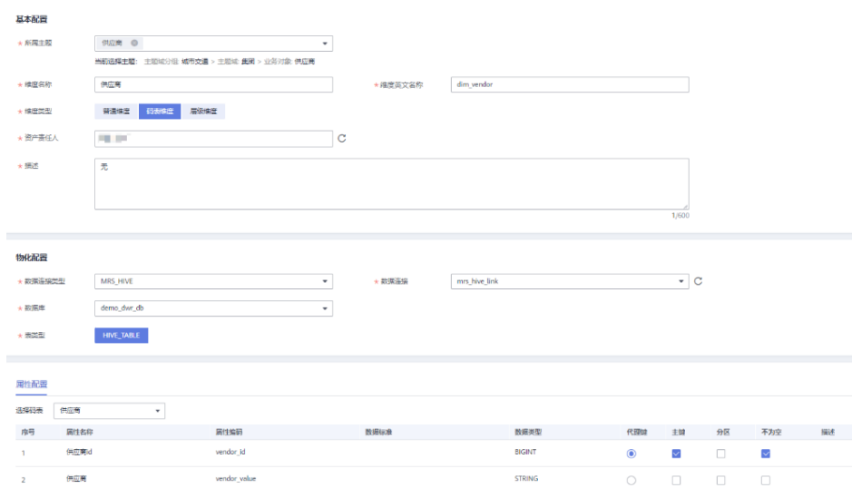
图 4-60 新建维度
