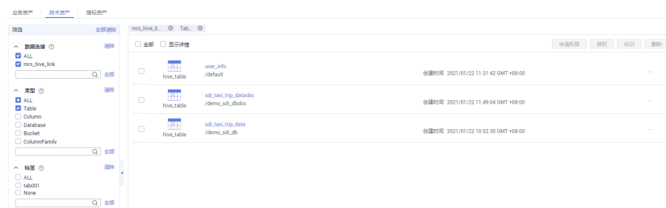
图 4-23 技术资产
