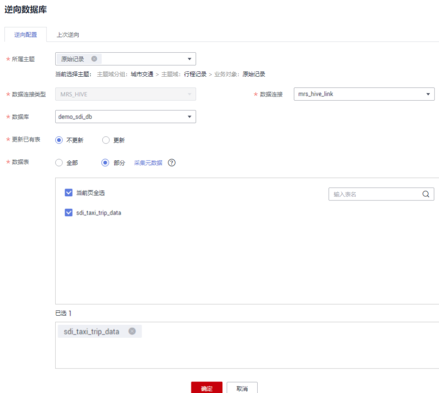
图 4-50 逆向数据库
