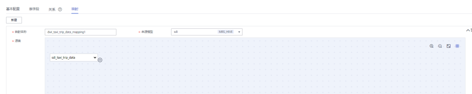
图 4-54 新建映射
