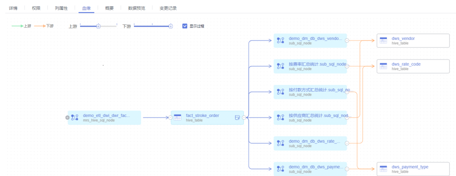
图 4-111 血缘
