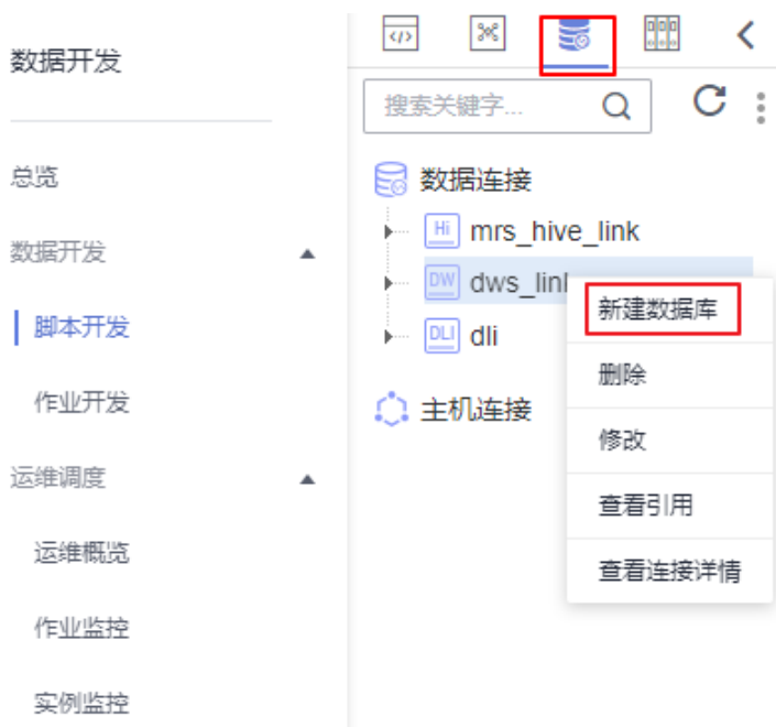
图 3-4 创建数据库
