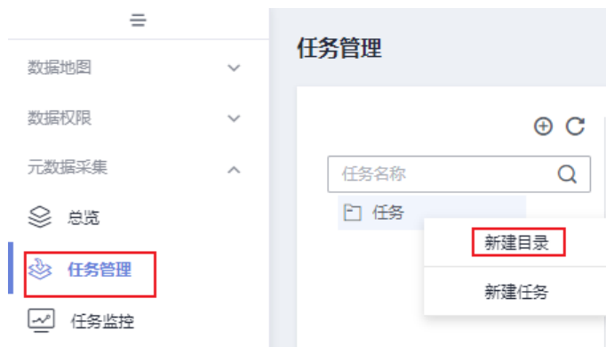
图 4-17 任务管理
