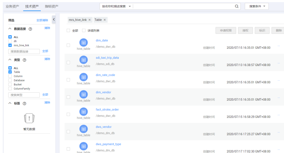
图 4-110 技术资产
