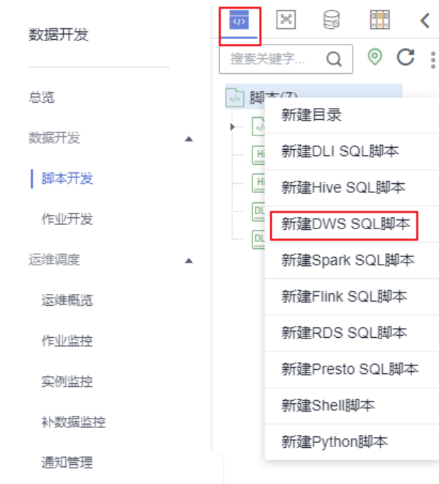
图 3-25 新建脚本
