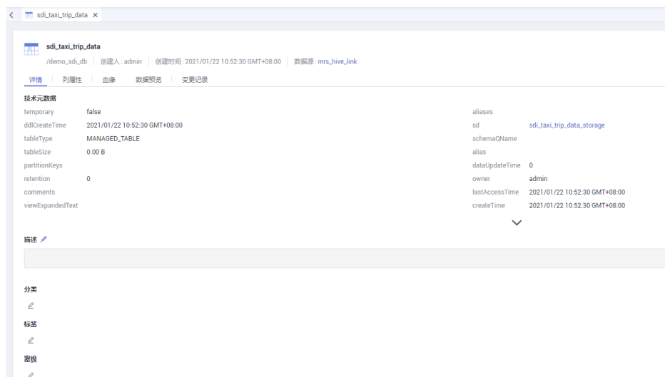
图 4-24 元数据详情
