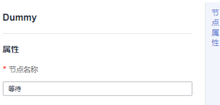
图 4-92 等待节点
